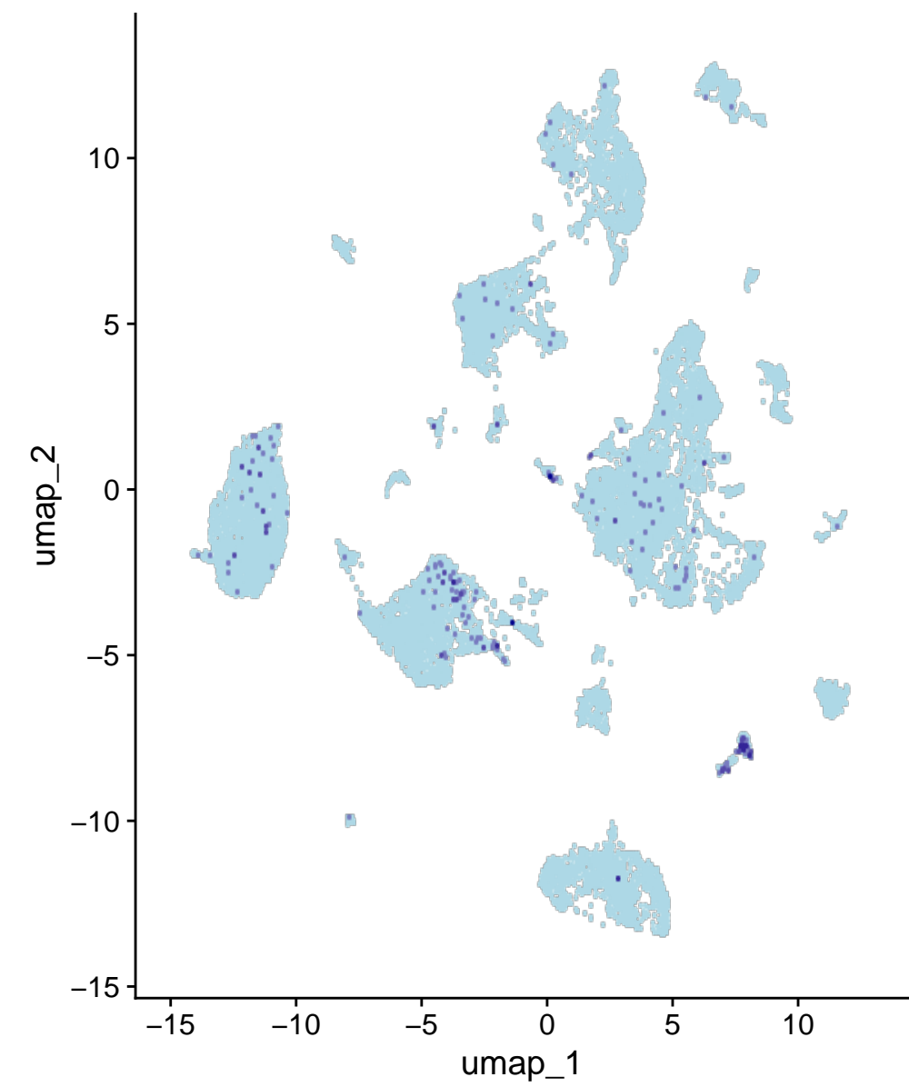
Ctxn3
