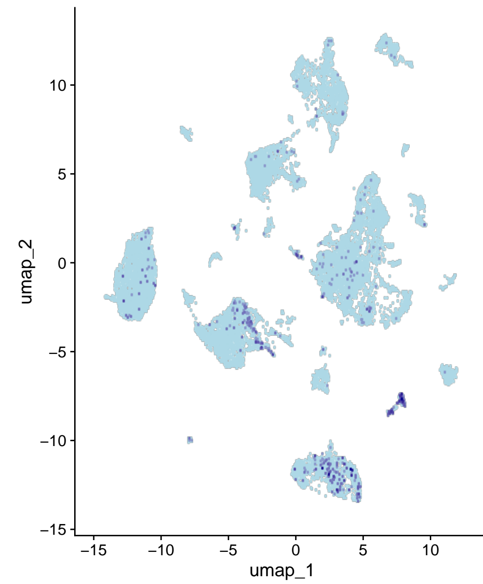
Kih1
