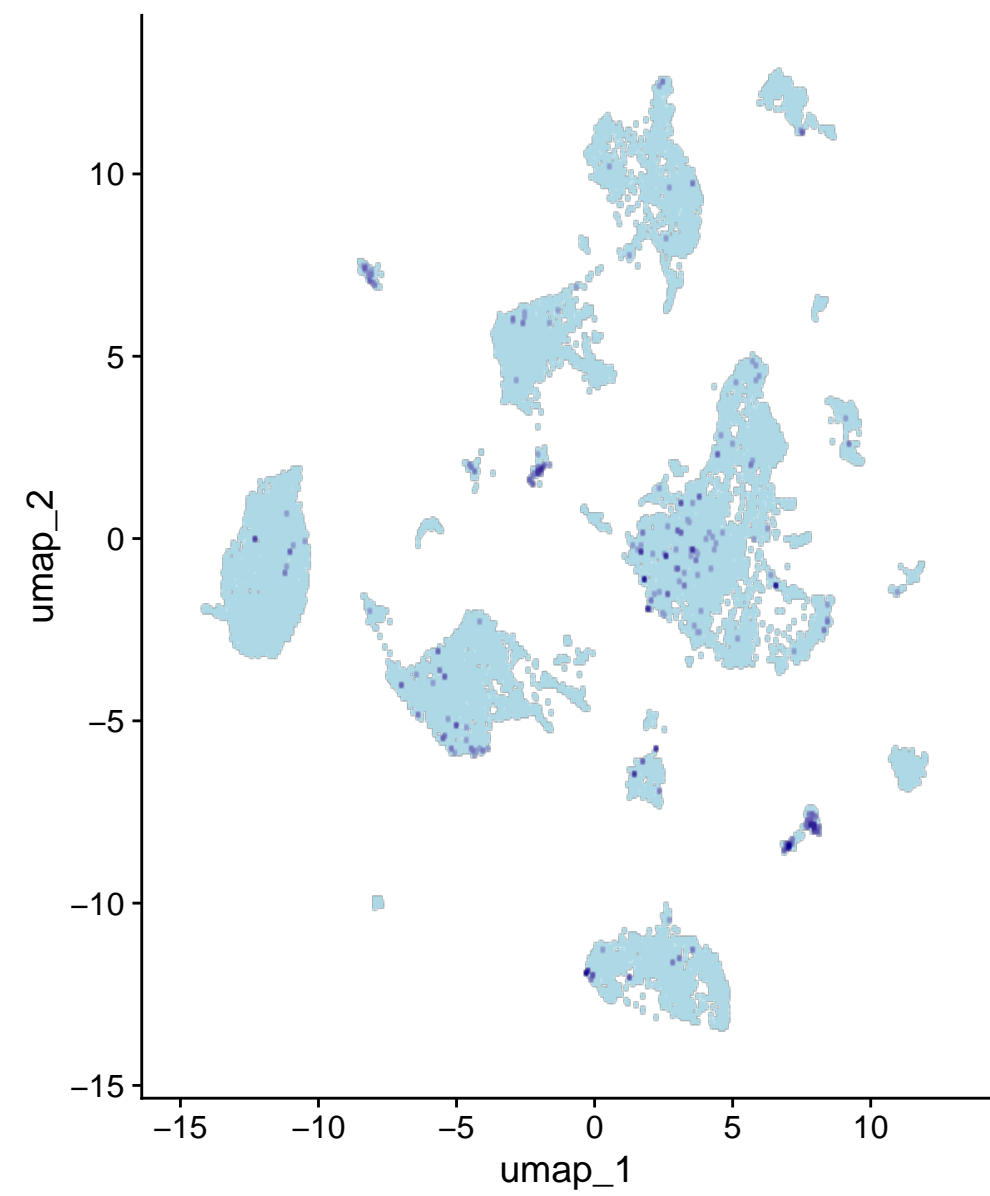
Pdgfd
