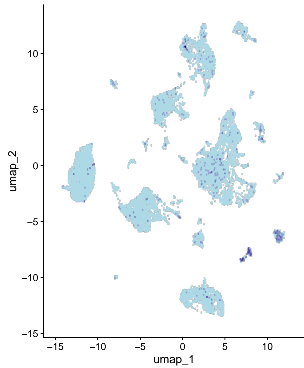
Plpp4
