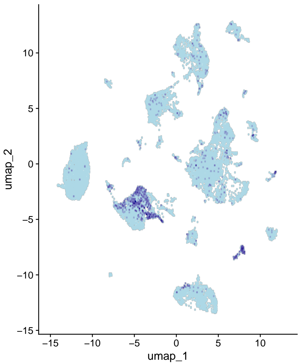
Trdn
