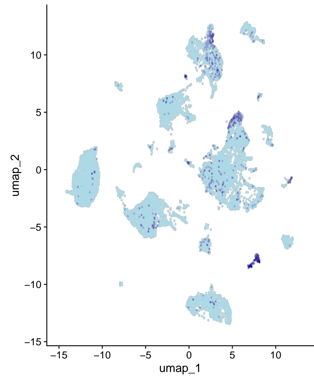
9130008F23Rik
