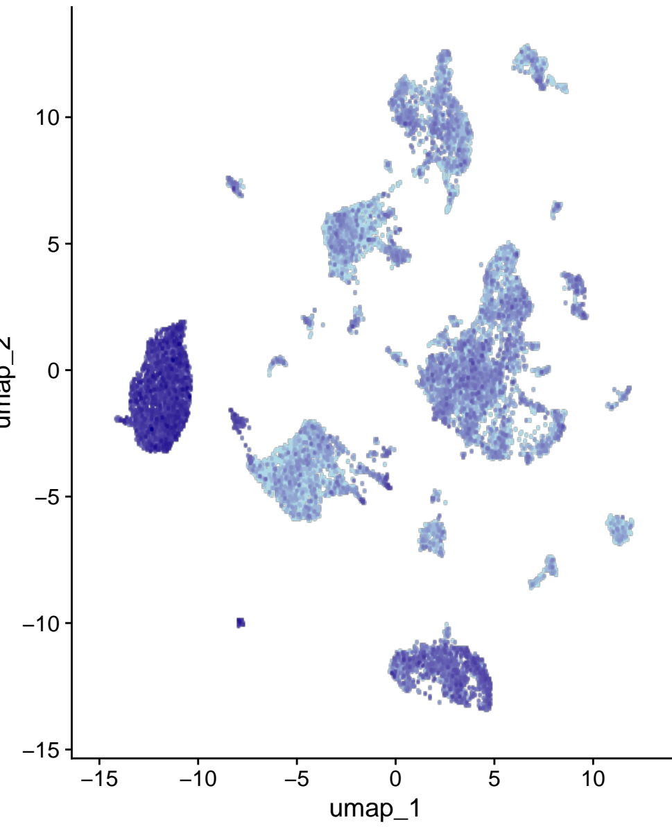
Plcl1
