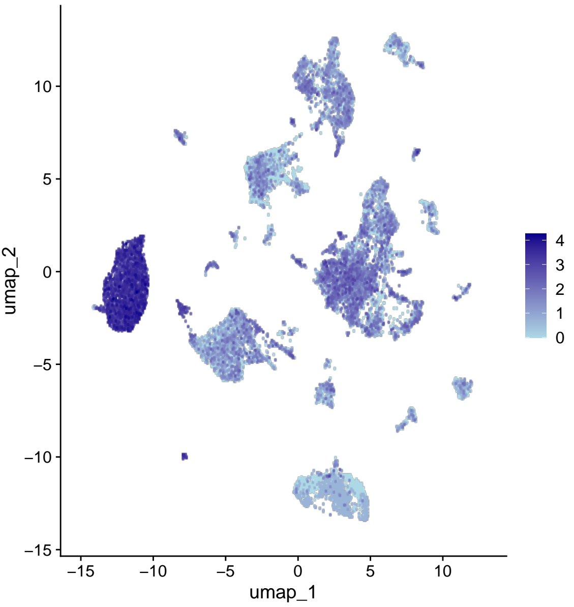
Pde4b
