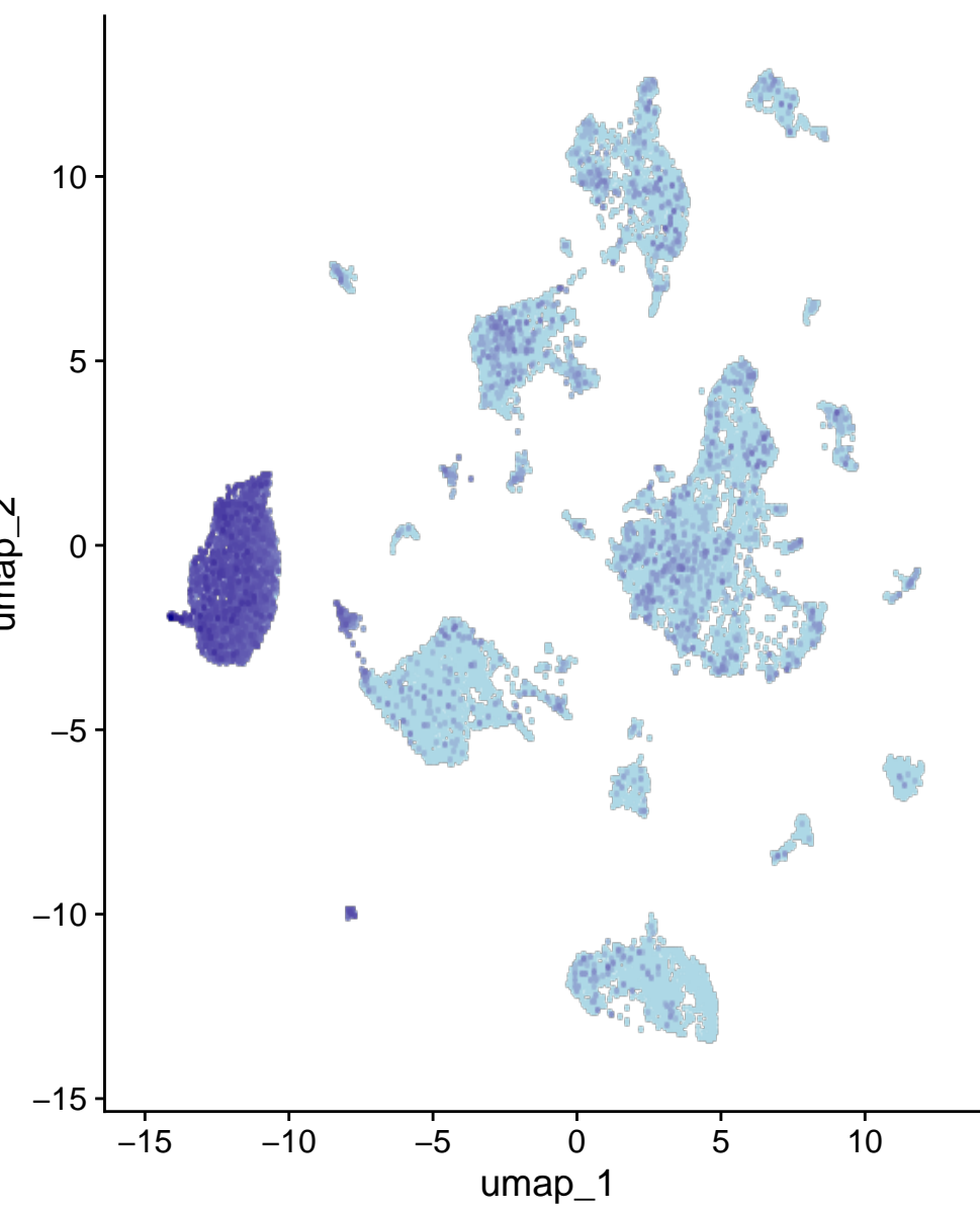
Enpp2
