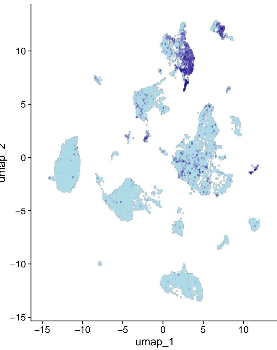
Rxfp1
