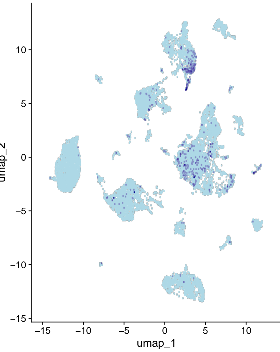
Klhl14
