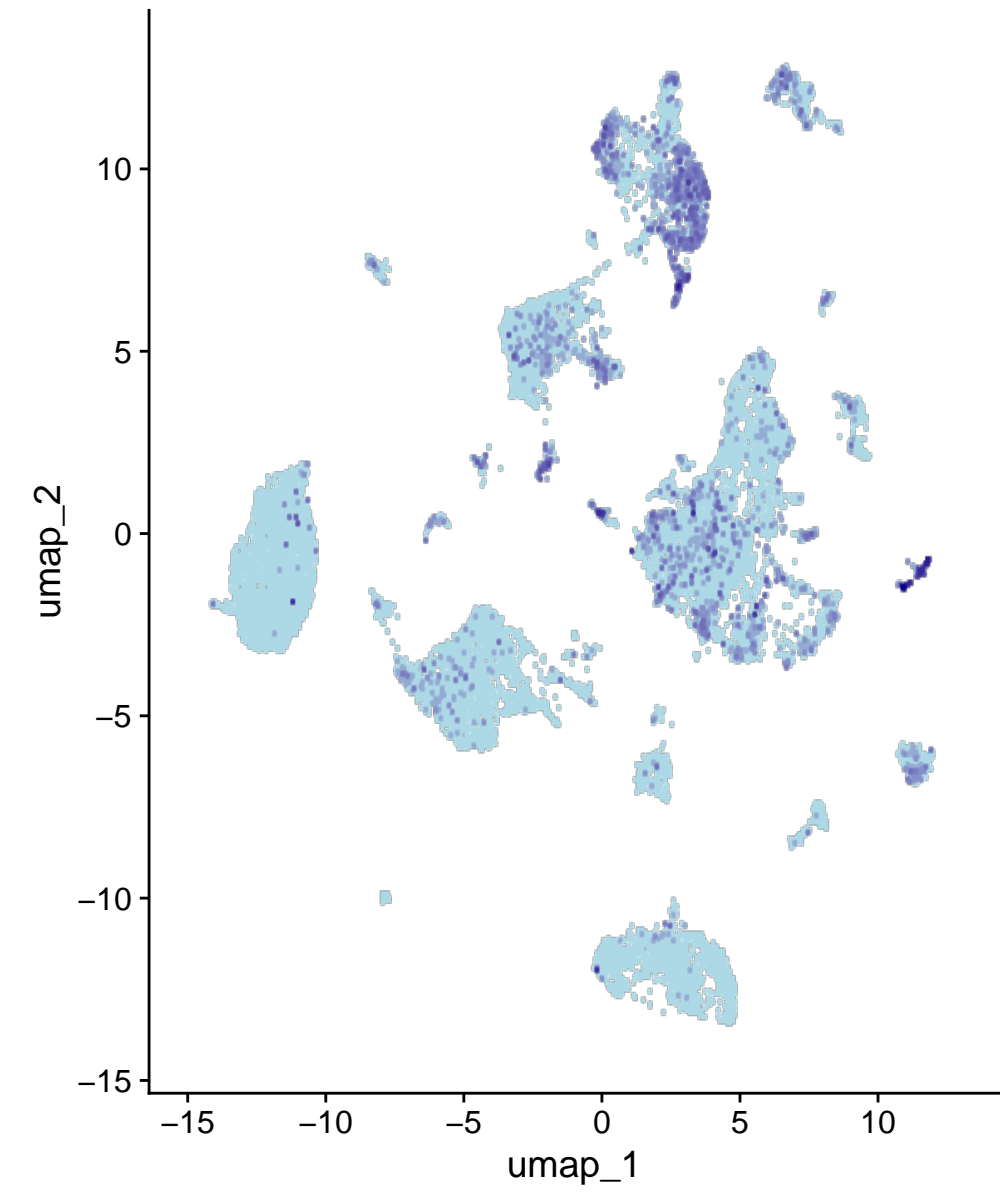
Lhfp
