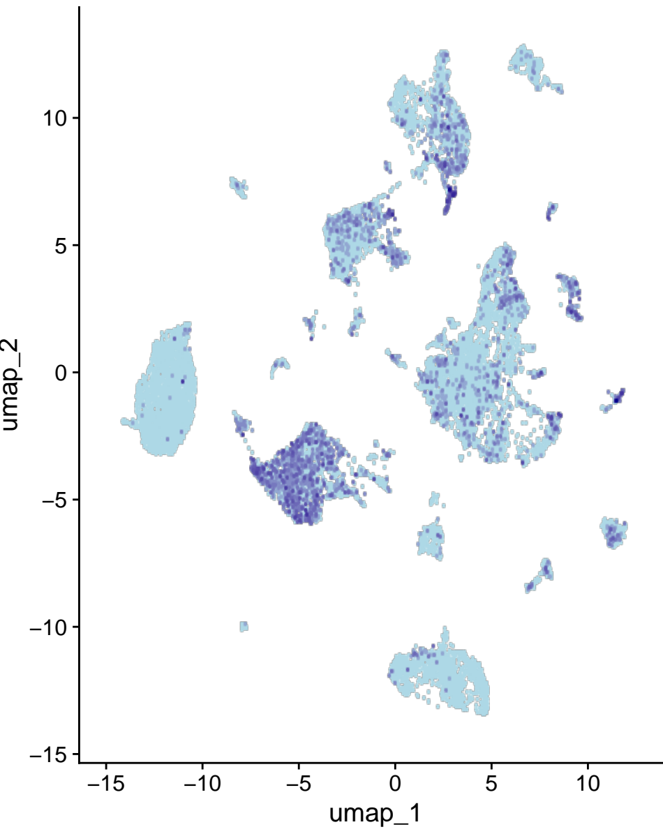
Tll1
