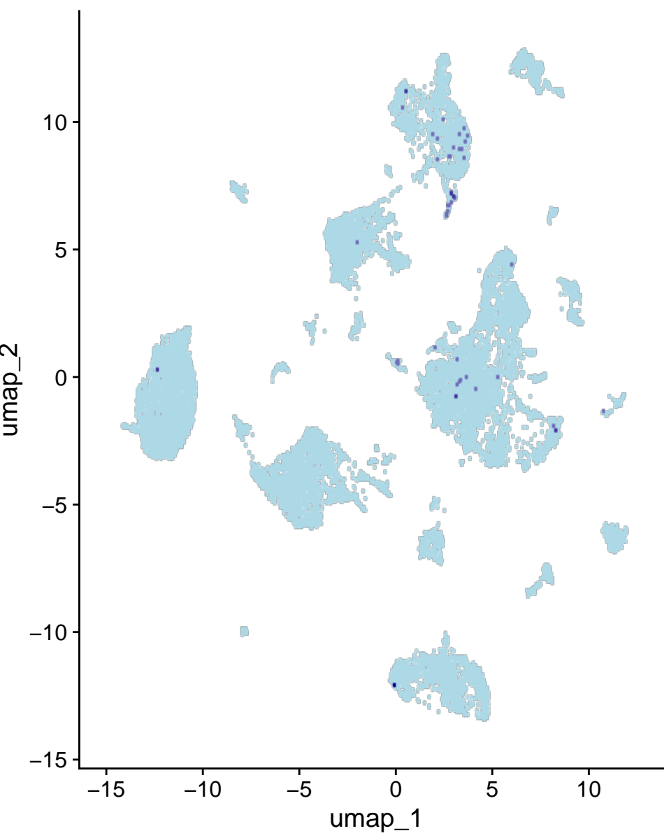
L3mbtl4
