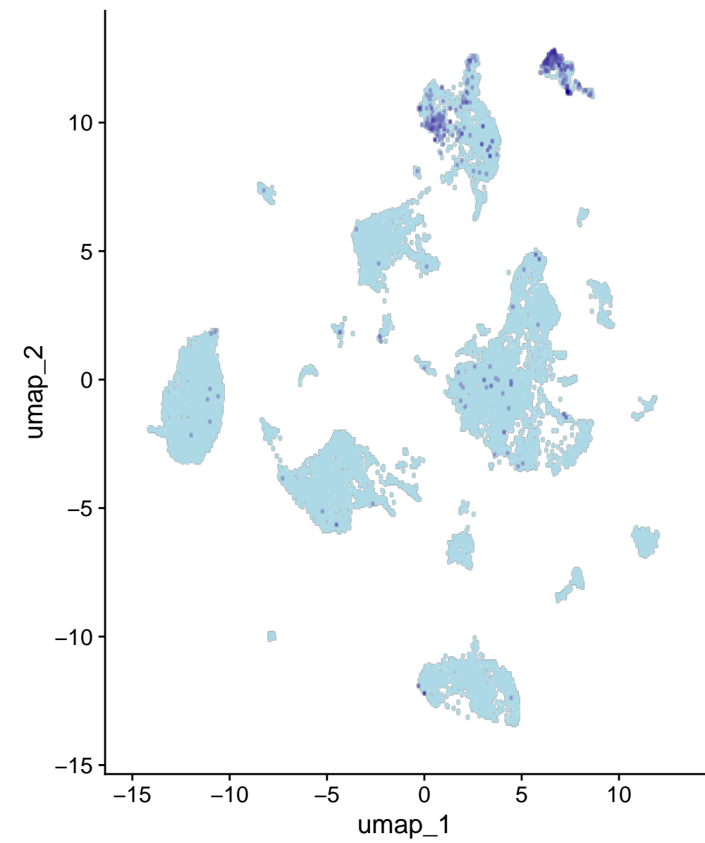
Trabd2b
