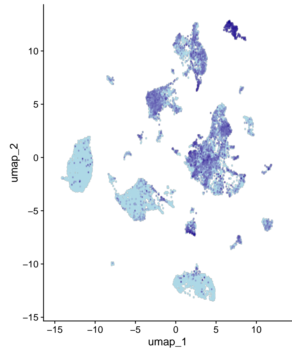
Rai14
