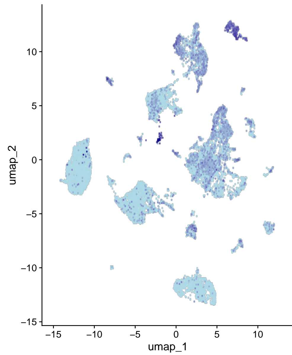
Prss12
