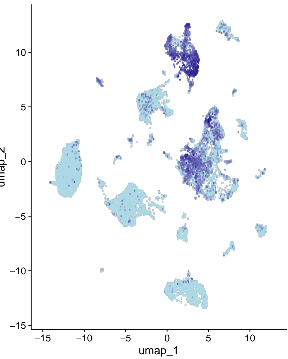
Syt17
