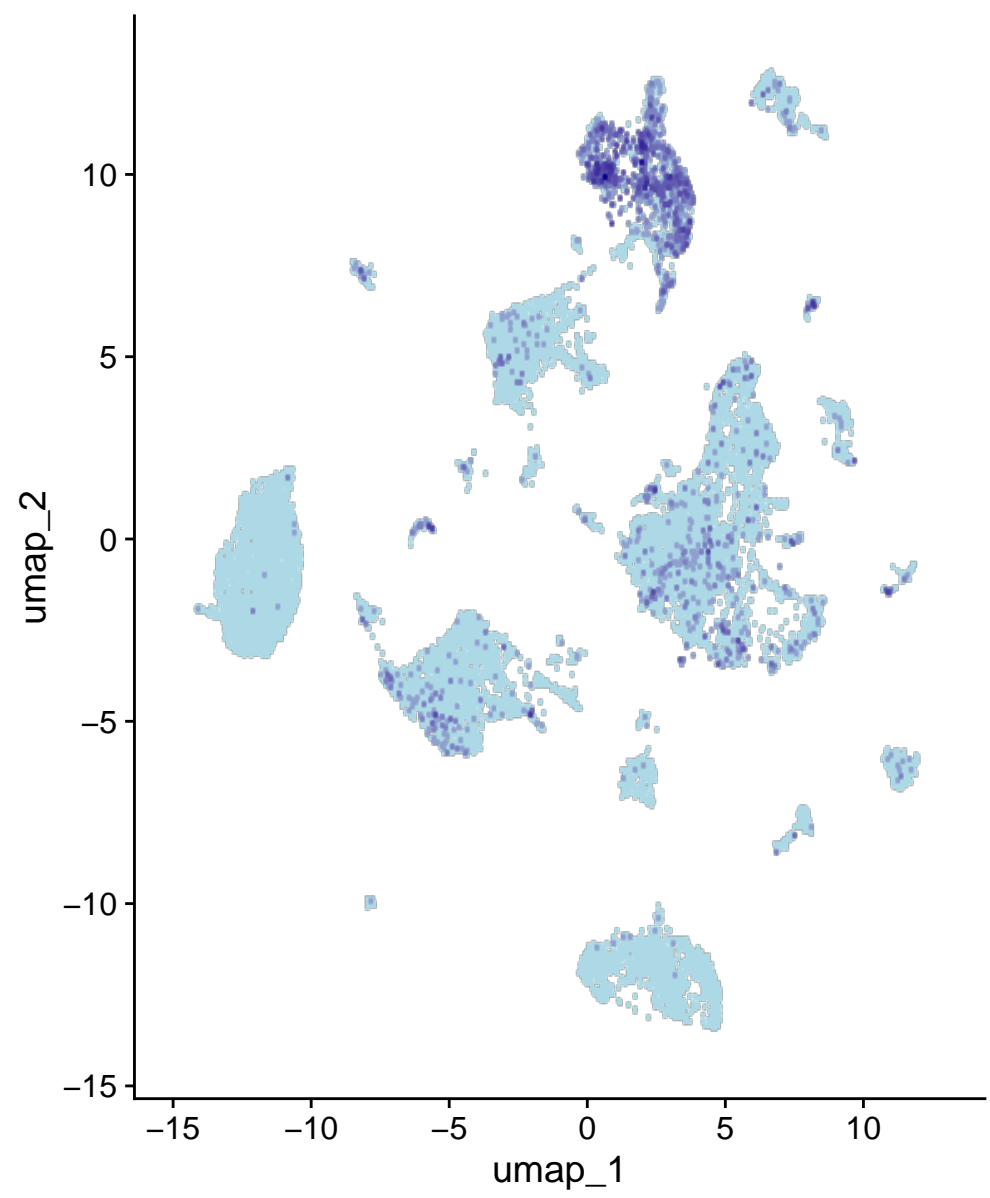
Ccdc3
