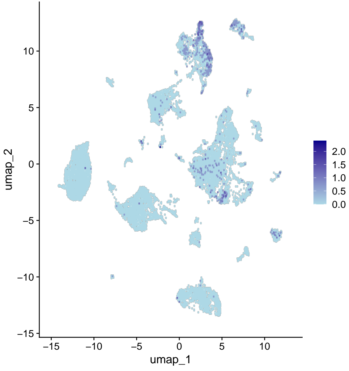
Npr3
