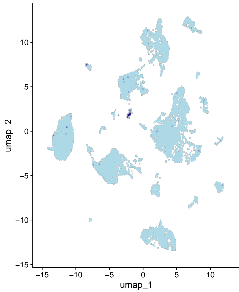
Gja1
