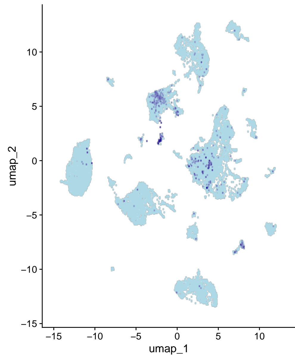
Ntsr2
