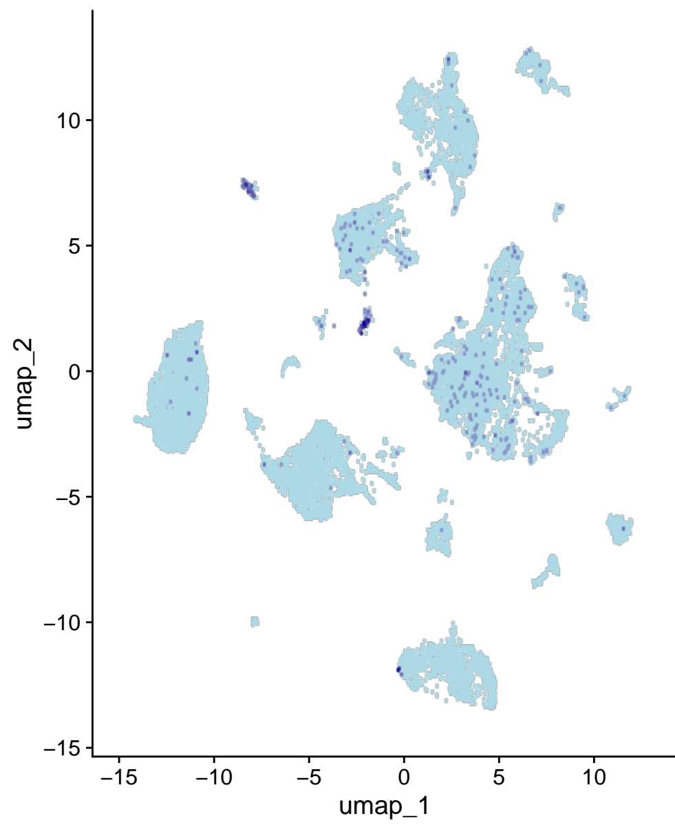
Etnppl
