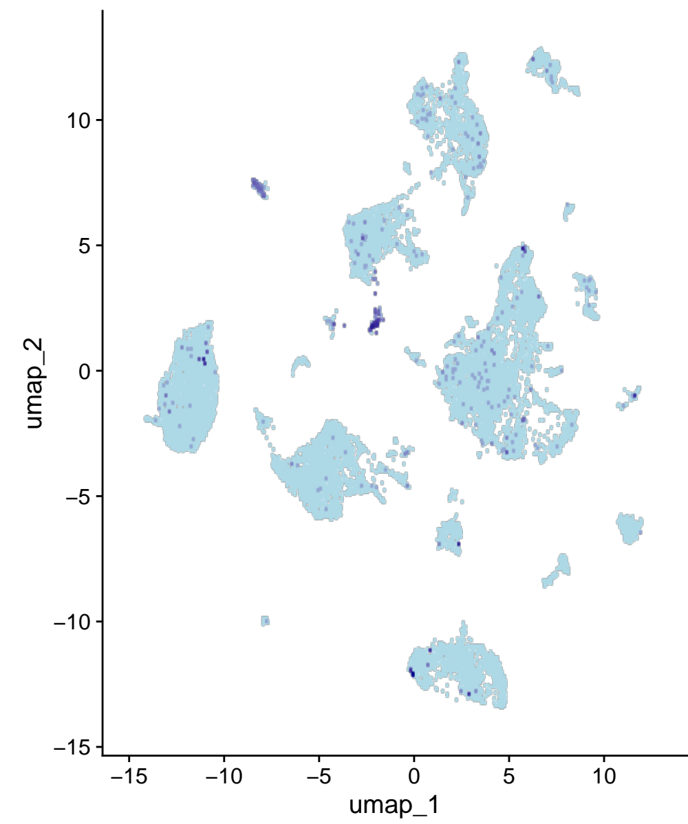
Slco1c1
