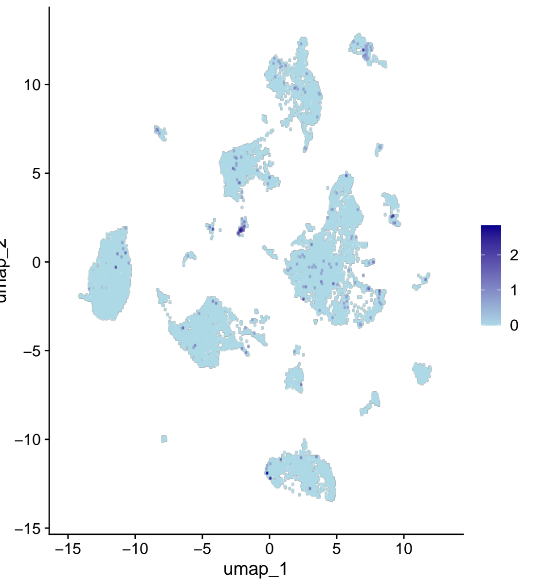
Gpr37l1
