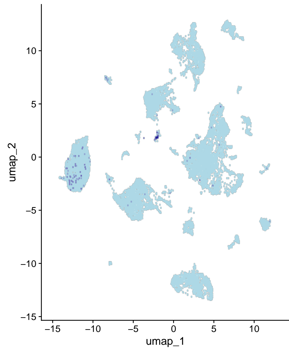
Itih3
