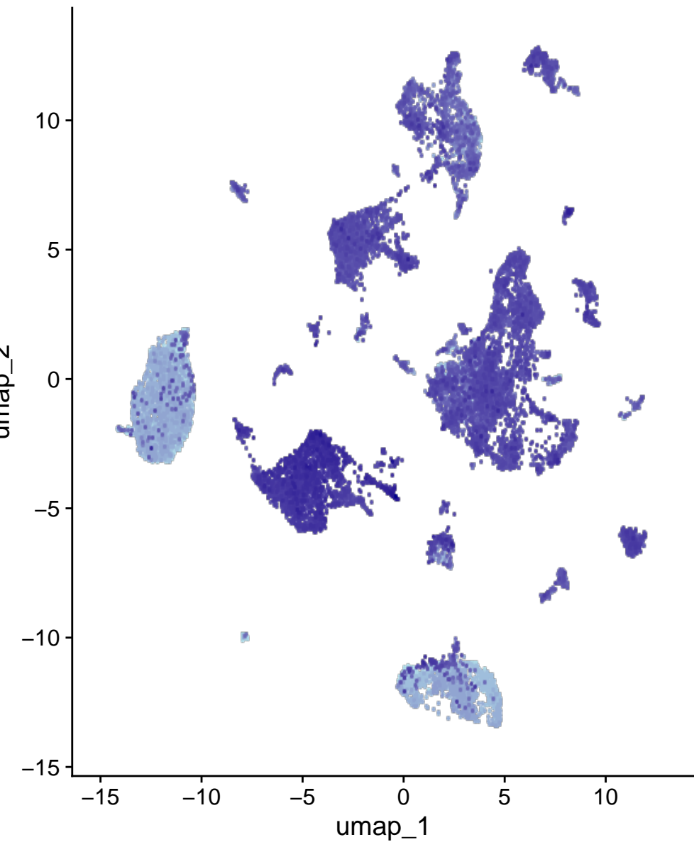
Tenm3
