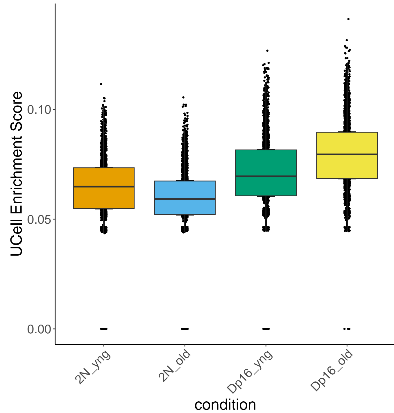
oligo : Tri16_UCell
