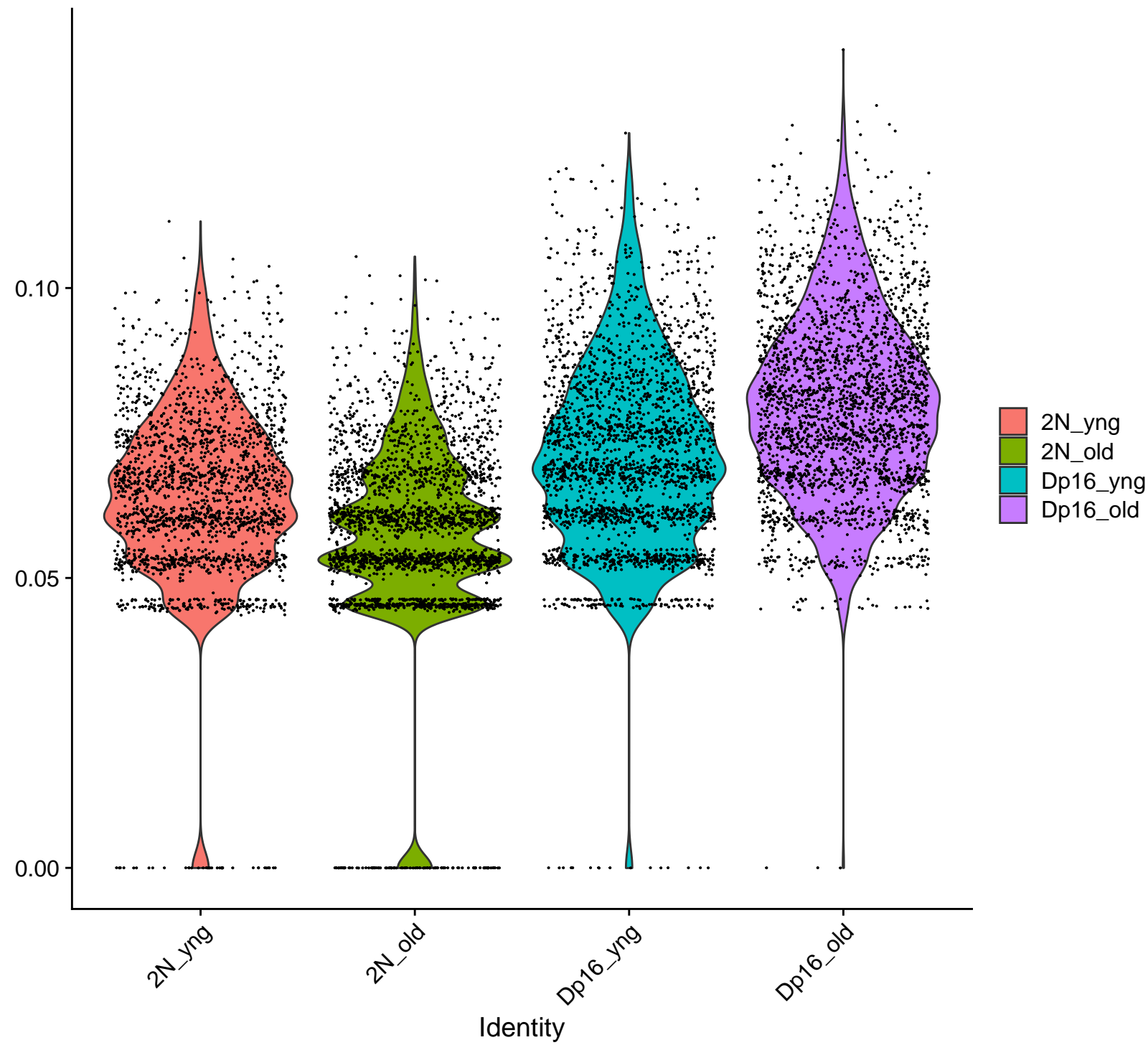
oligo : Tri16_UCell
