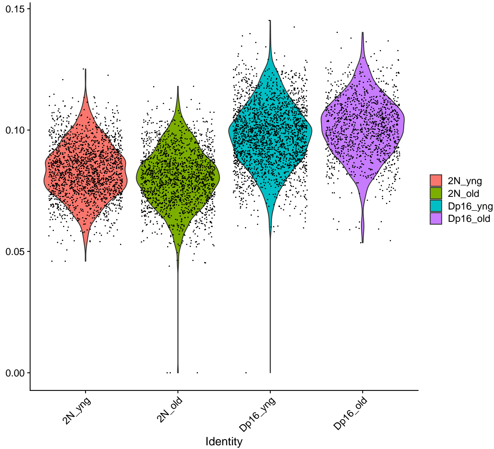
GABA2 : Tri16_UCell
