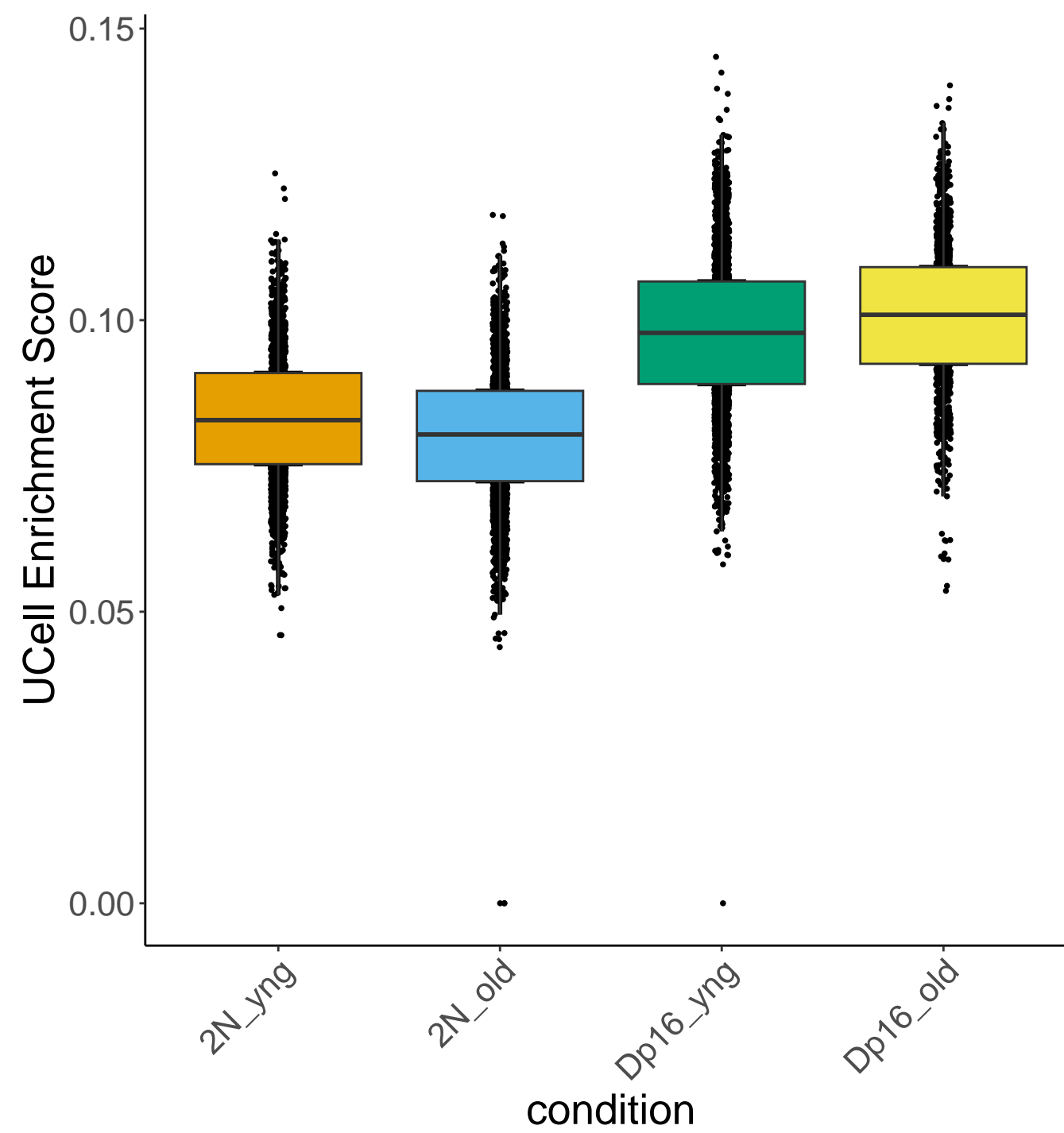
GABA2 : Tri16_UCell
