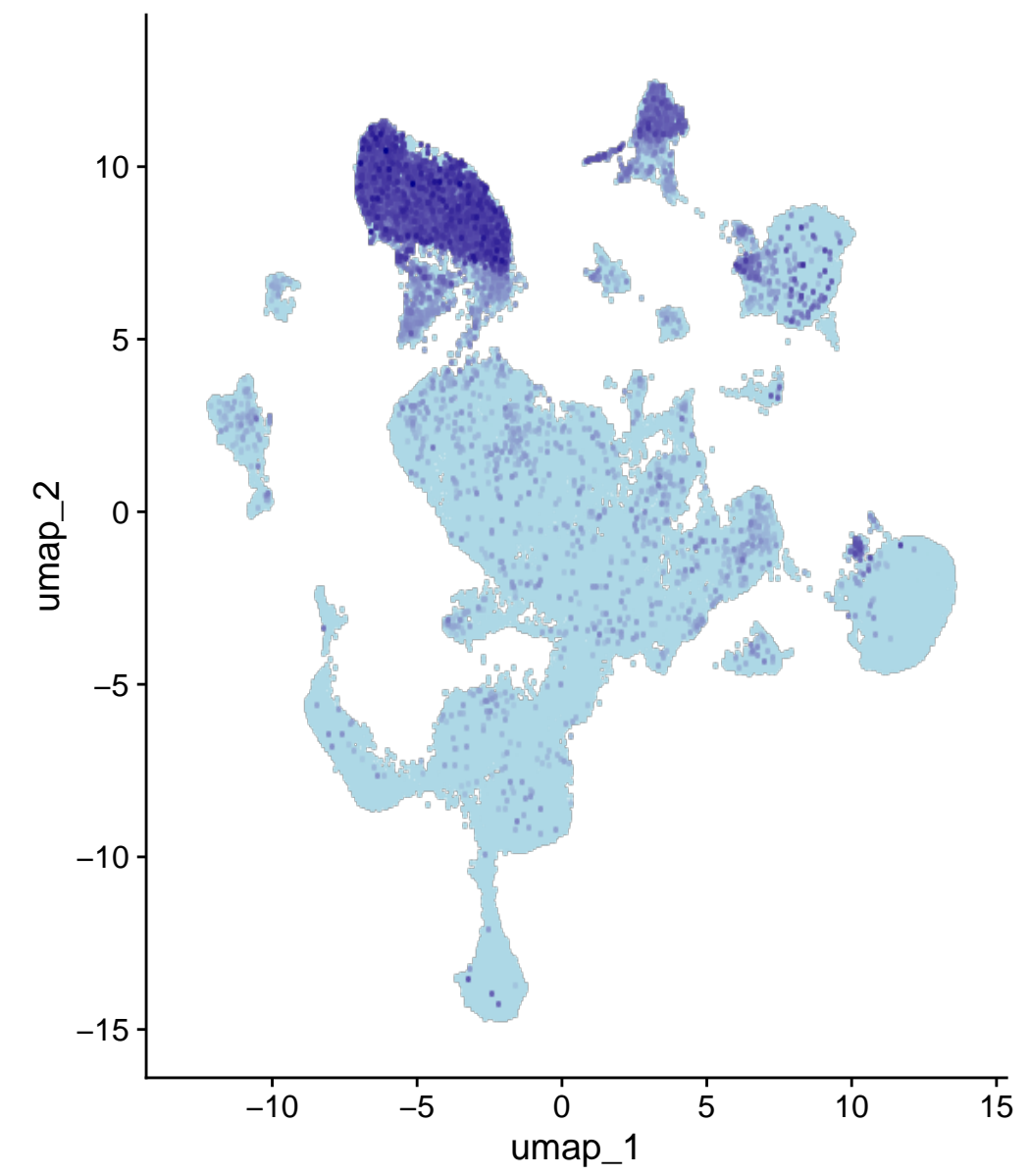
Olig1
