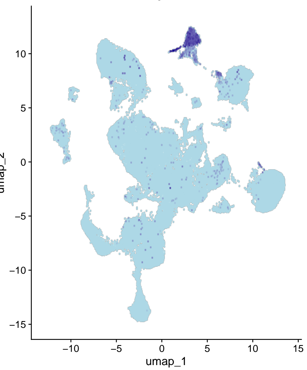
Enpp6
