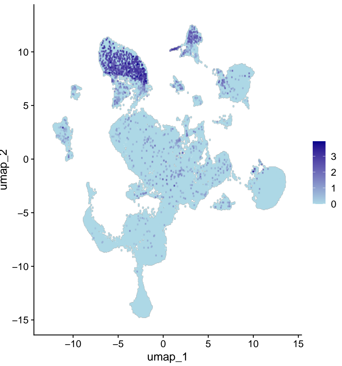
Bfsp2
