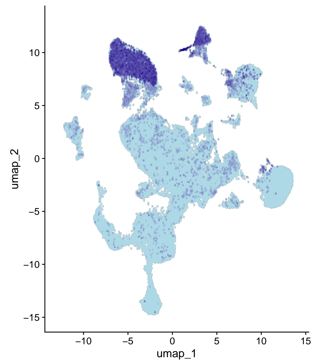
1700047M11Rik
