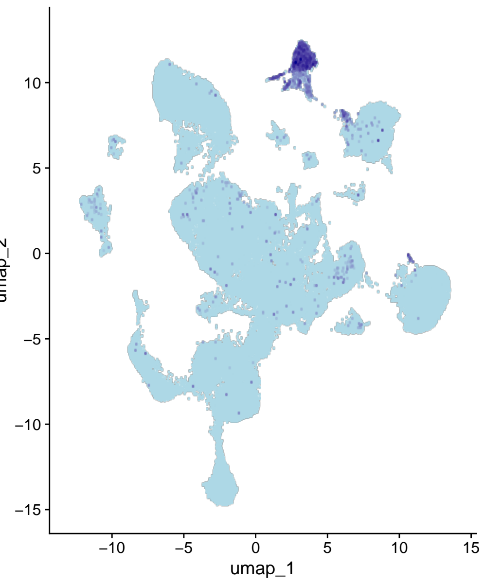
Neu4
