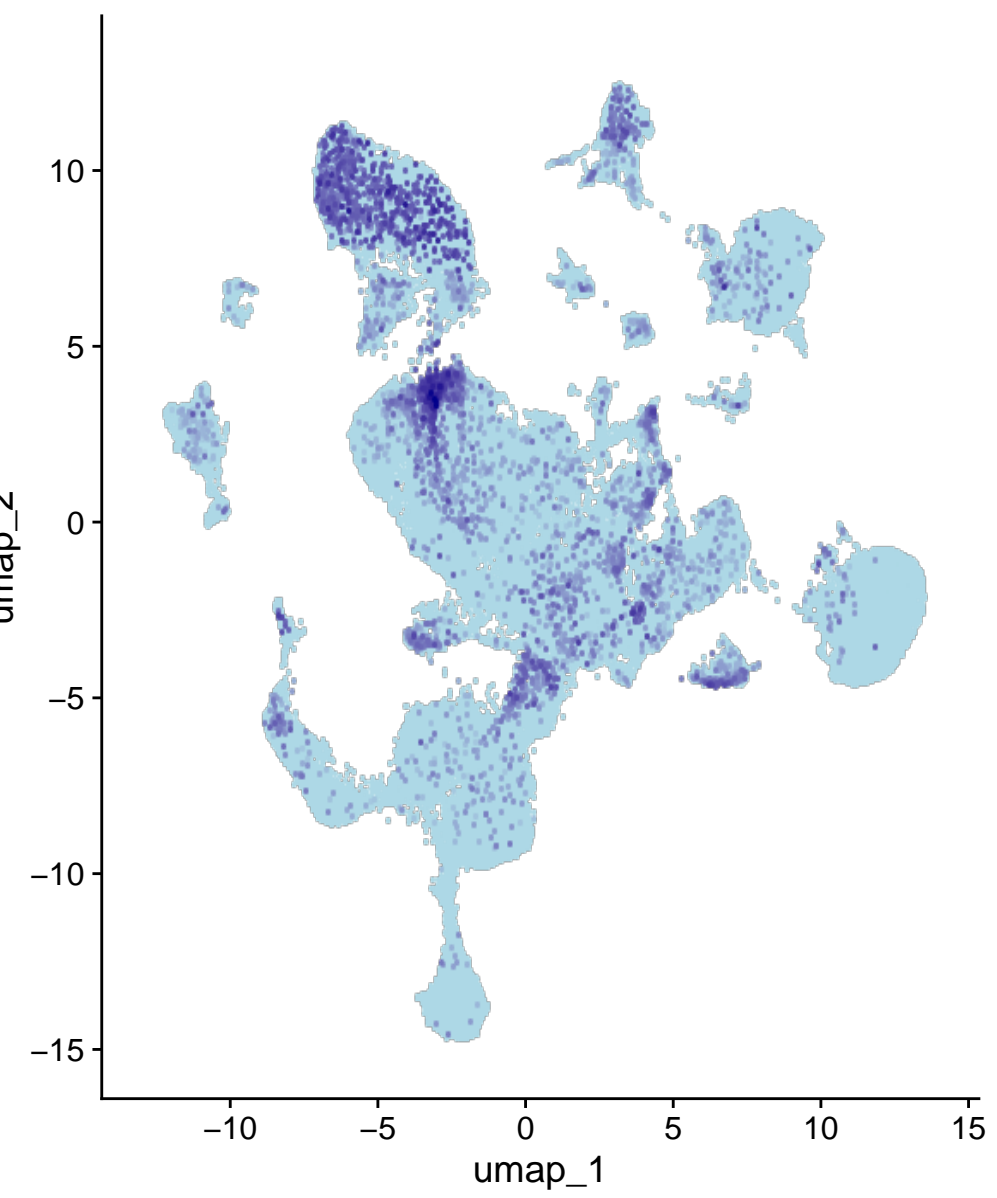
Ppm1e
