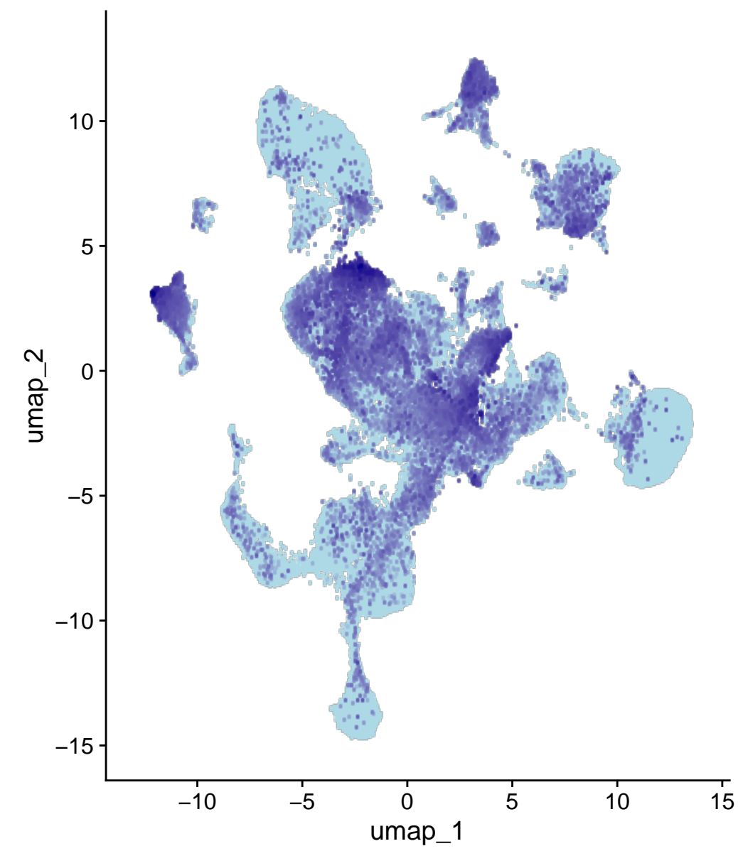
Dgkg
