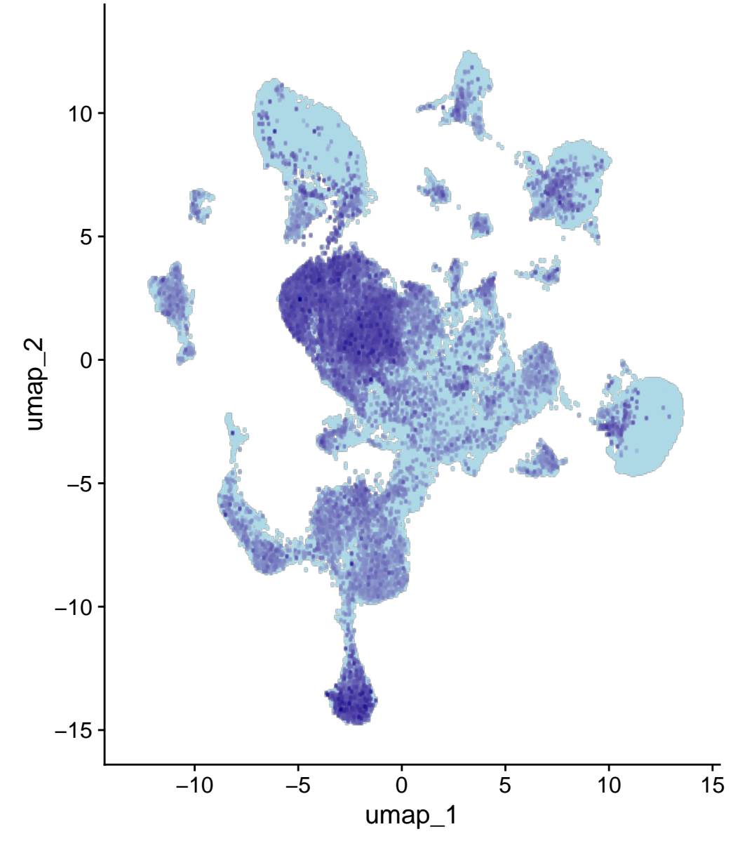
Myo5b
