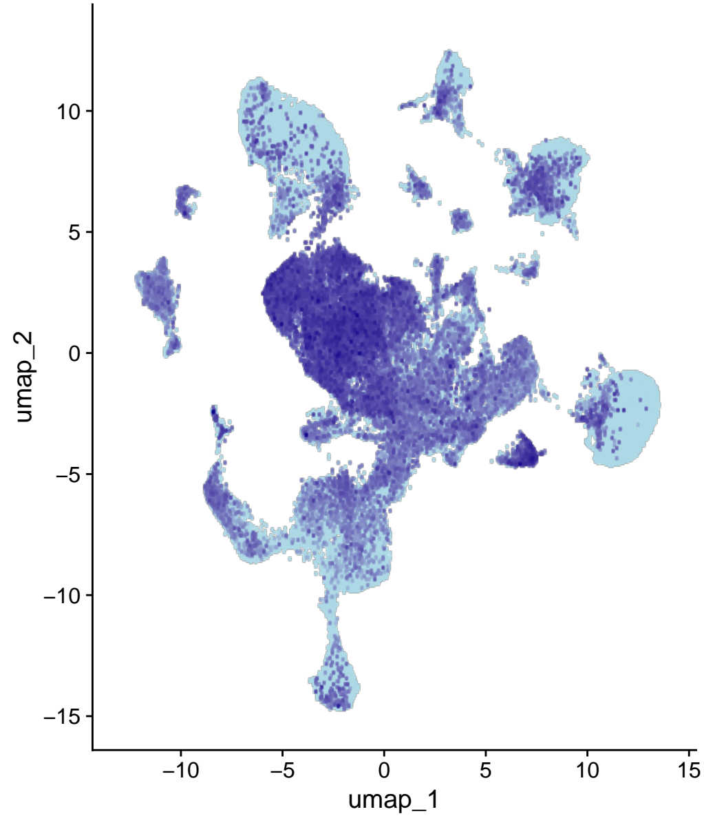
Trpc4
