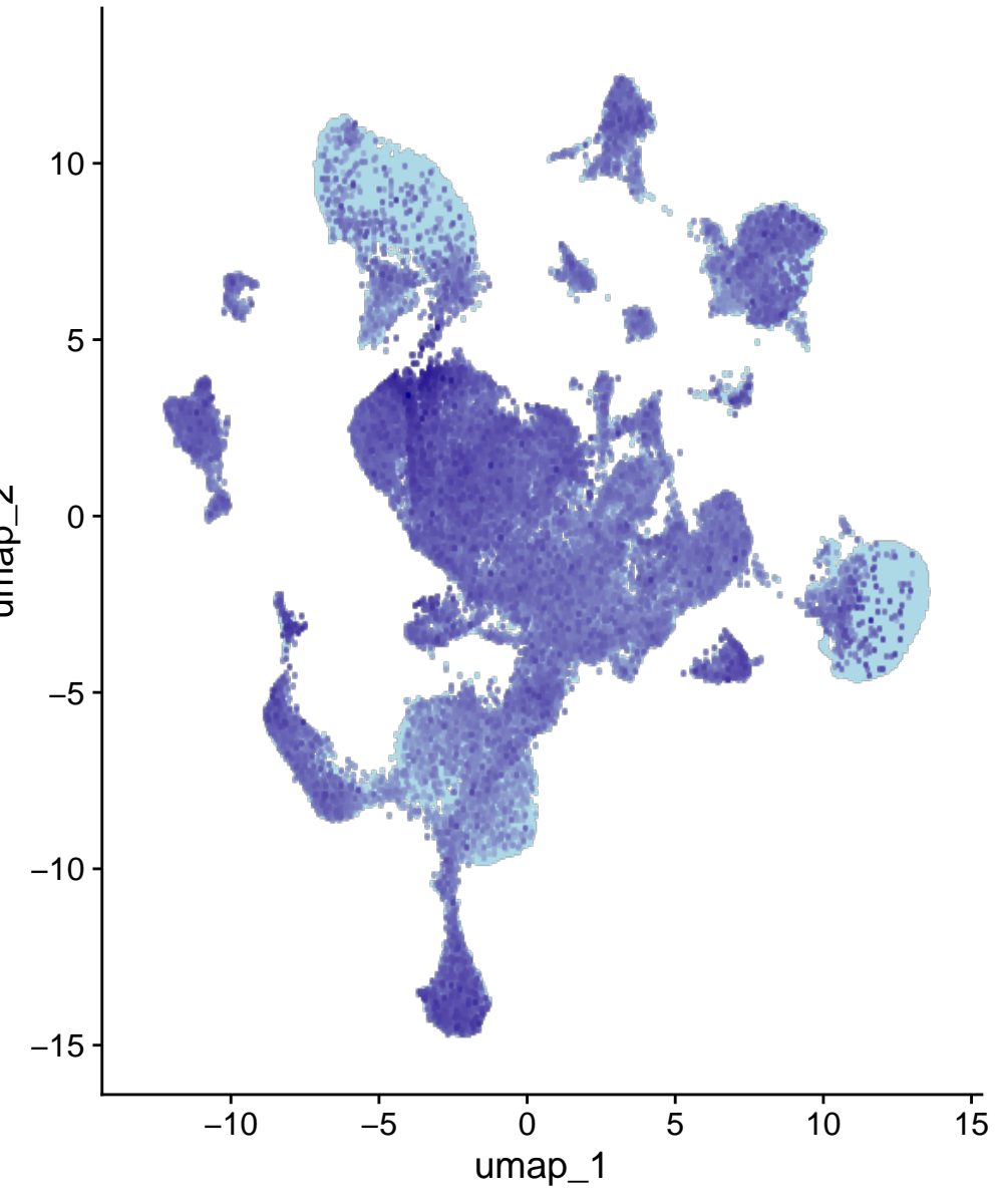
Ryr3
