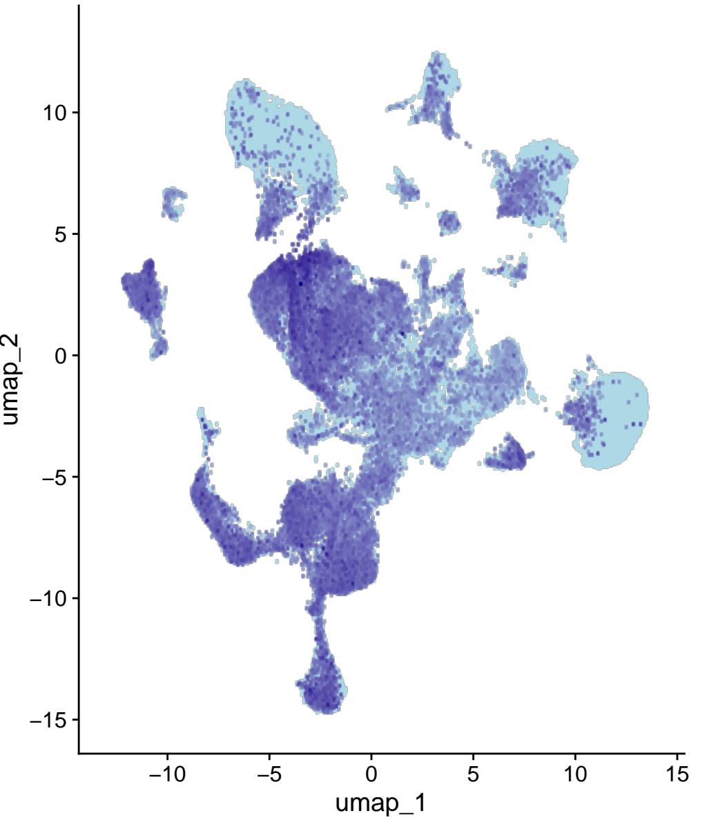
Hectd2
