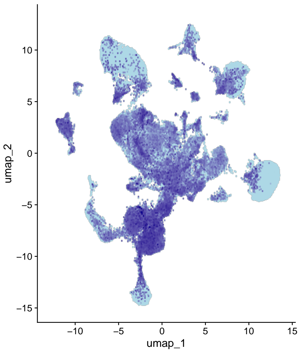
Greb1l
