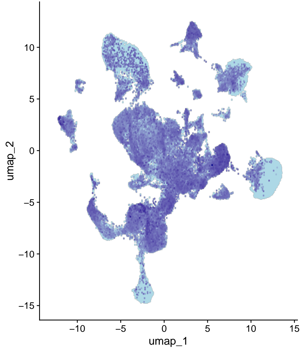
Sorcs3
