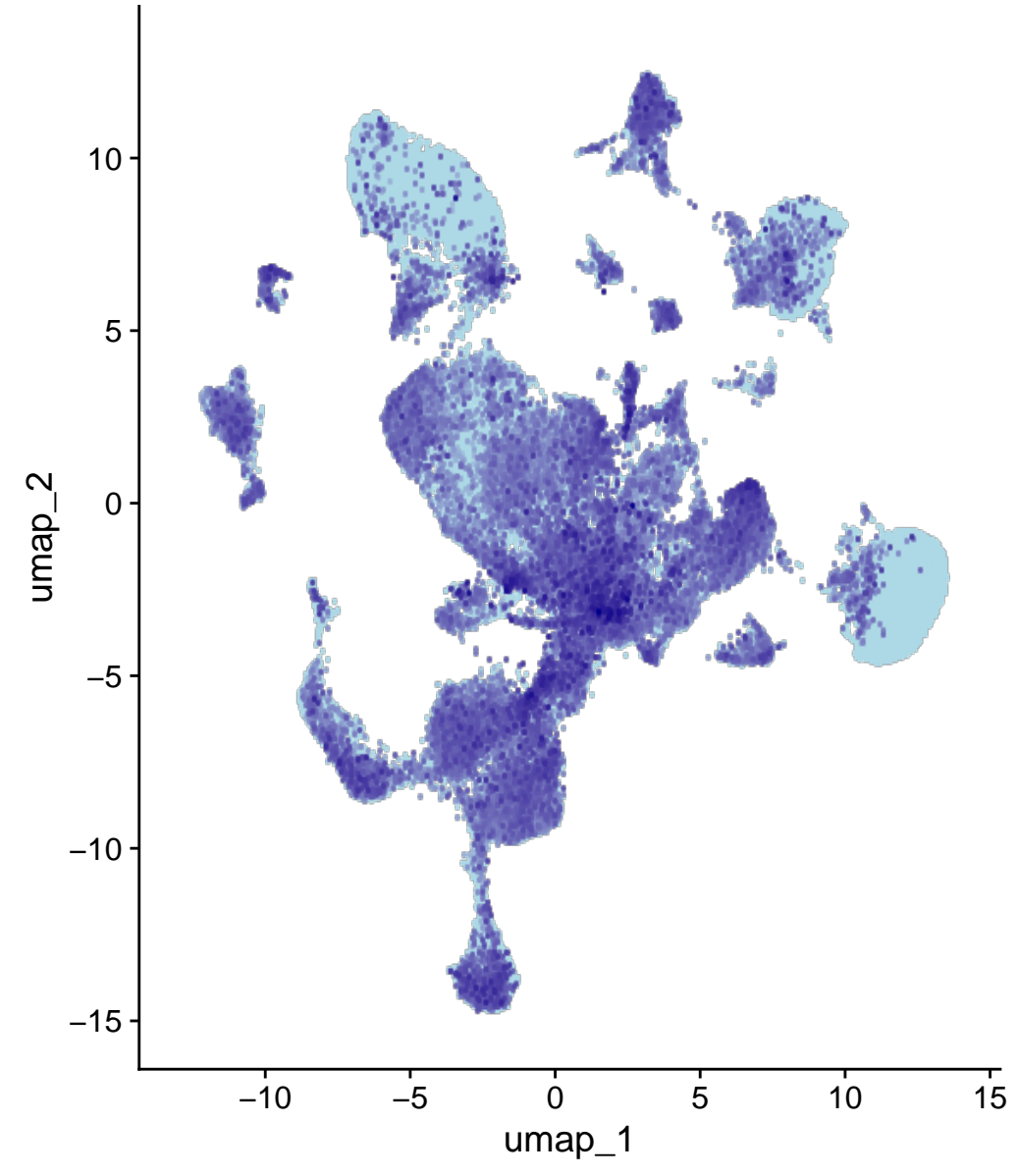
Pdzn4
