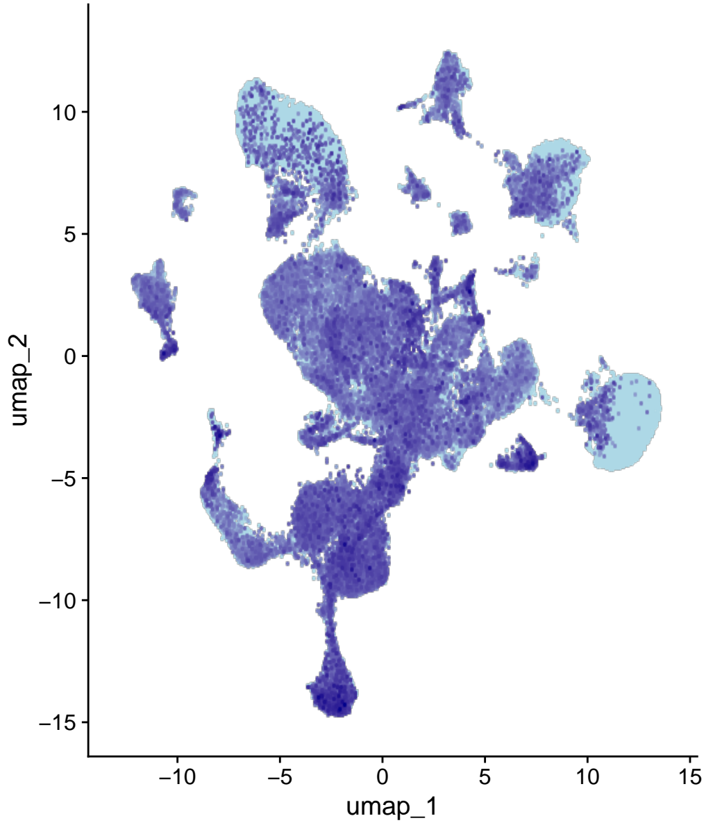
Chsy3
