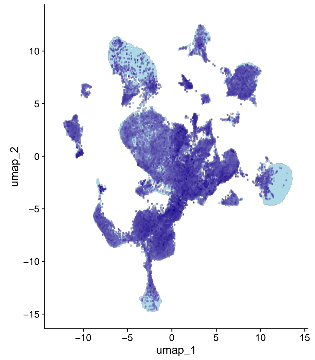
Dpyd
