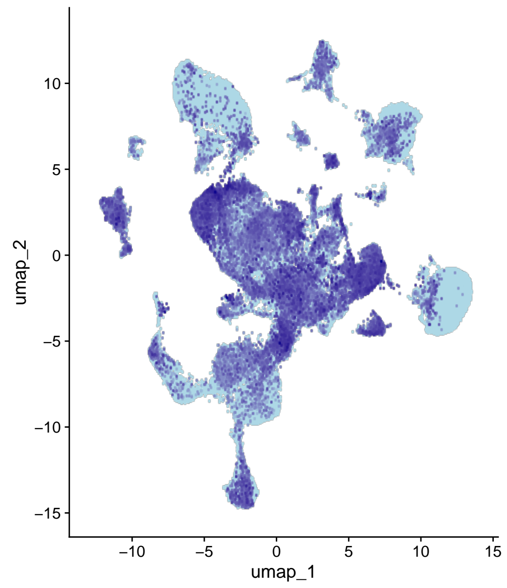
Zfp804b
