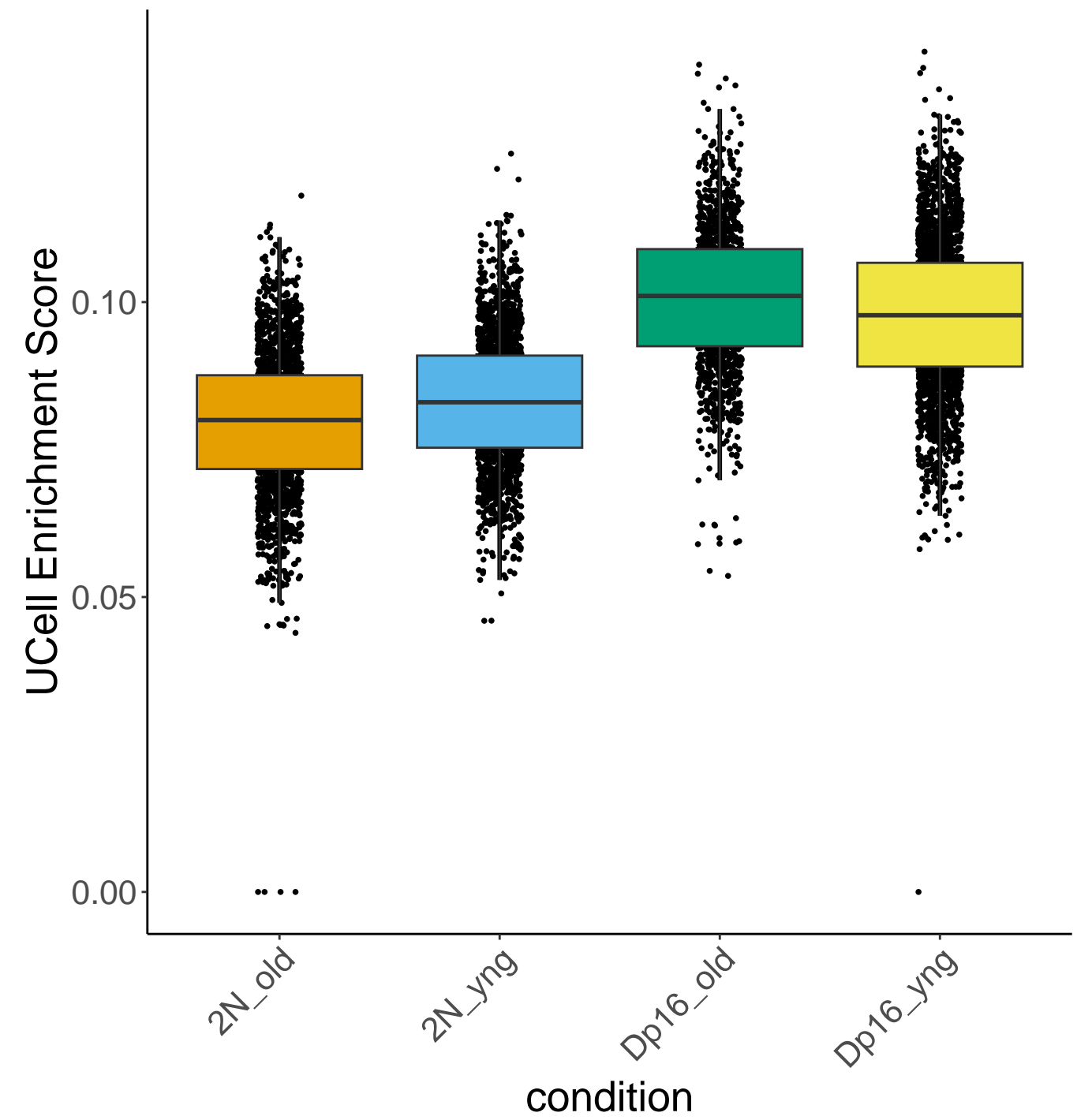
cl5 :Trisomic.Genes.Dp16
