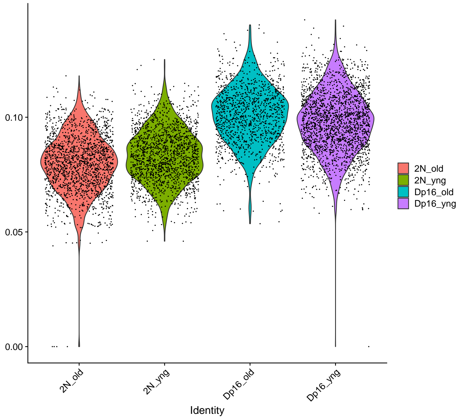
cl5 :Trisomic.Genes.Dp16
