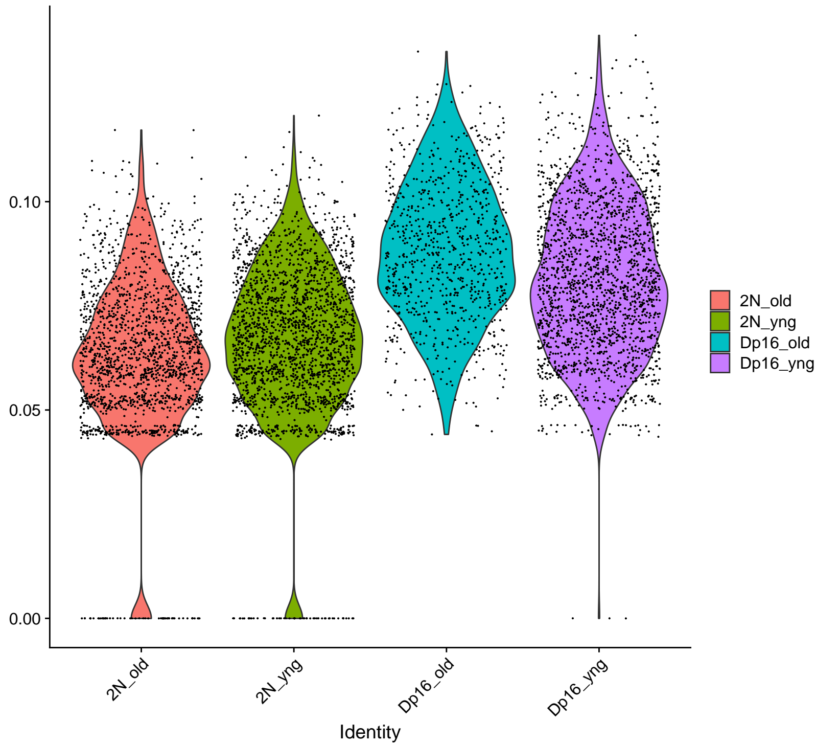
cl4 :Trisomic.Genes.Dp16
