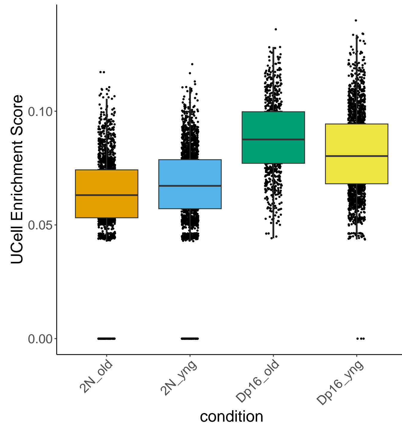
cl4 :Trisomic.Genes.Dp16
