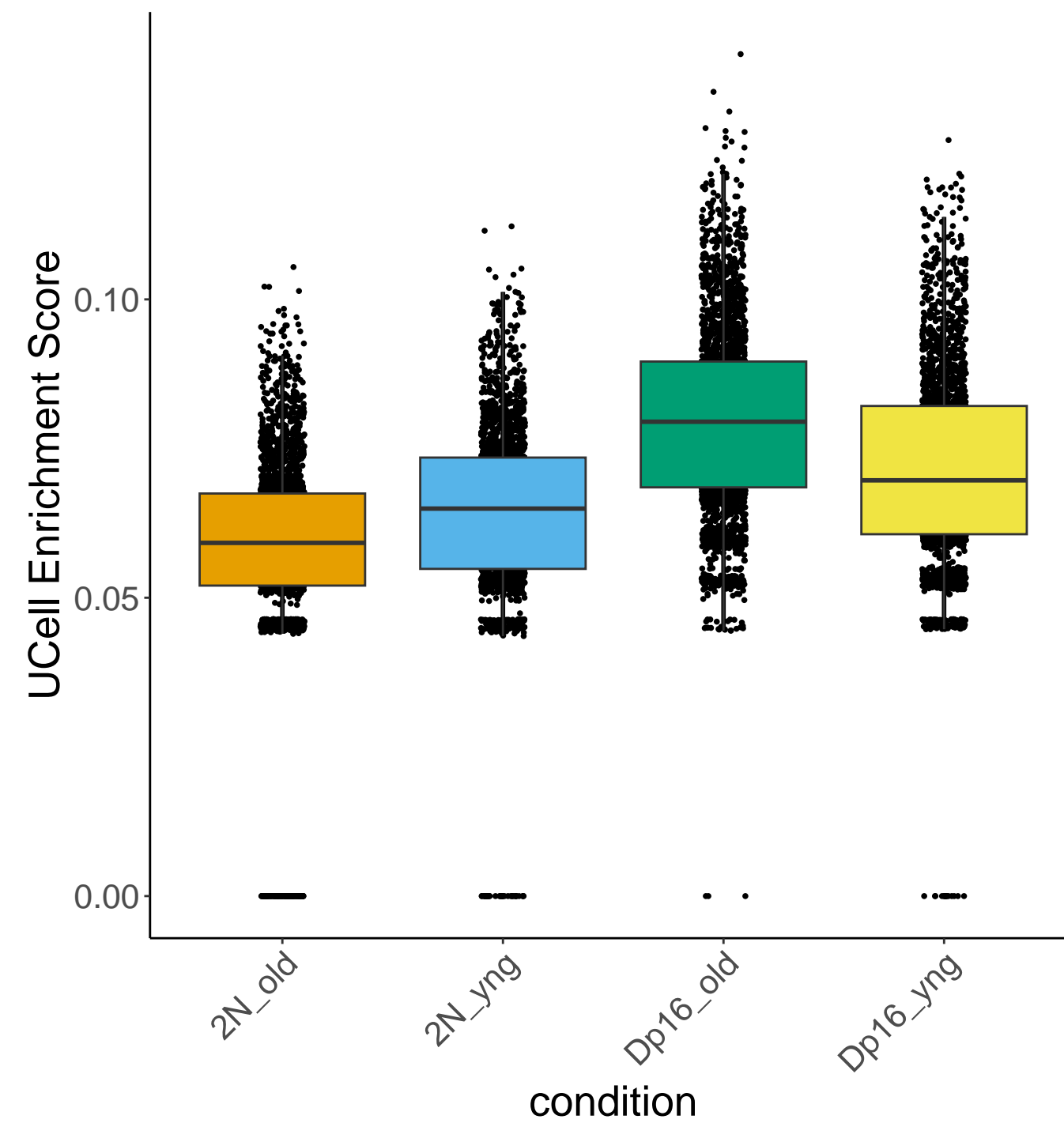
cl2 :Trisomic.Genes.Dp16
