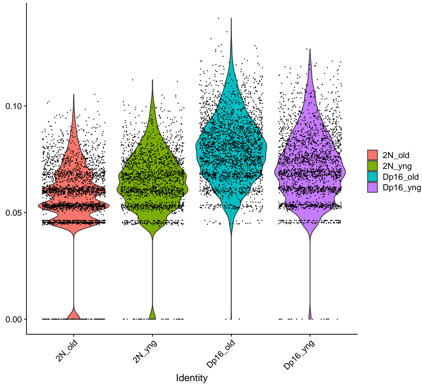
cl2 :Trisomic.Genes.Dp16
