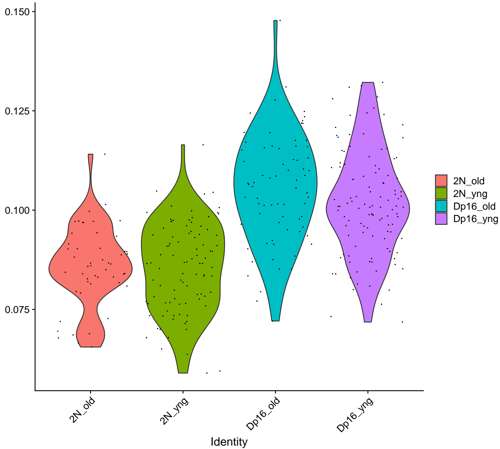
cl23 :Trisomic.Genes.Dp16
