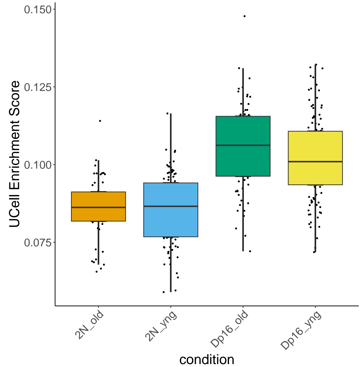
cl23 :Trisomic.Genes.Dp16
