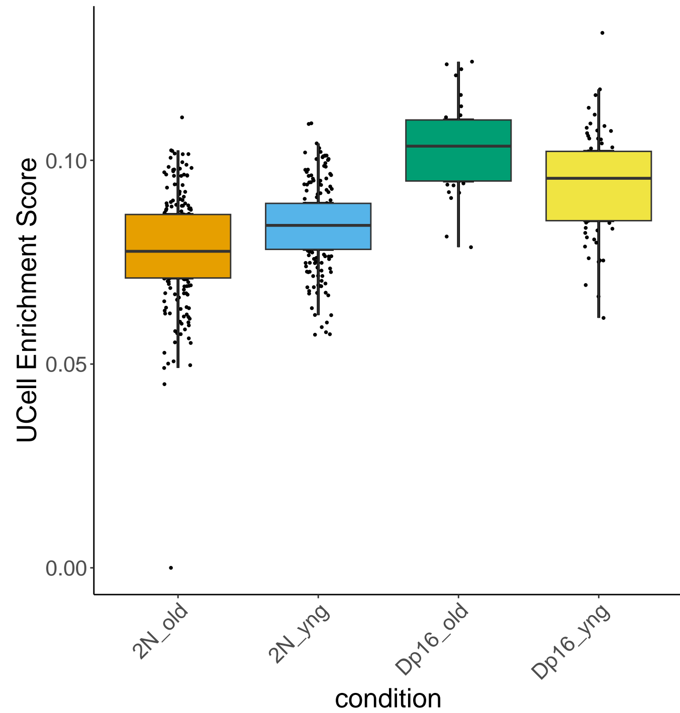
cl21 :Trisomic.Genes.Dp16
