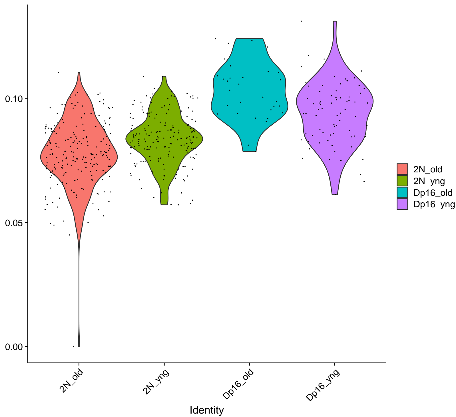
cl21 :Trisomic.Genes.Dp16
