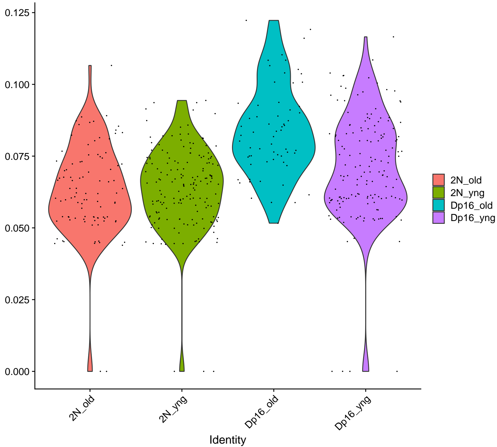
cl20 :Trisomic.Genes.Dp16
