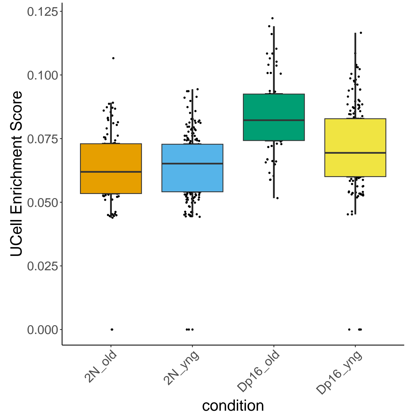
cl20 :Trisomic.Genes.Dp16
