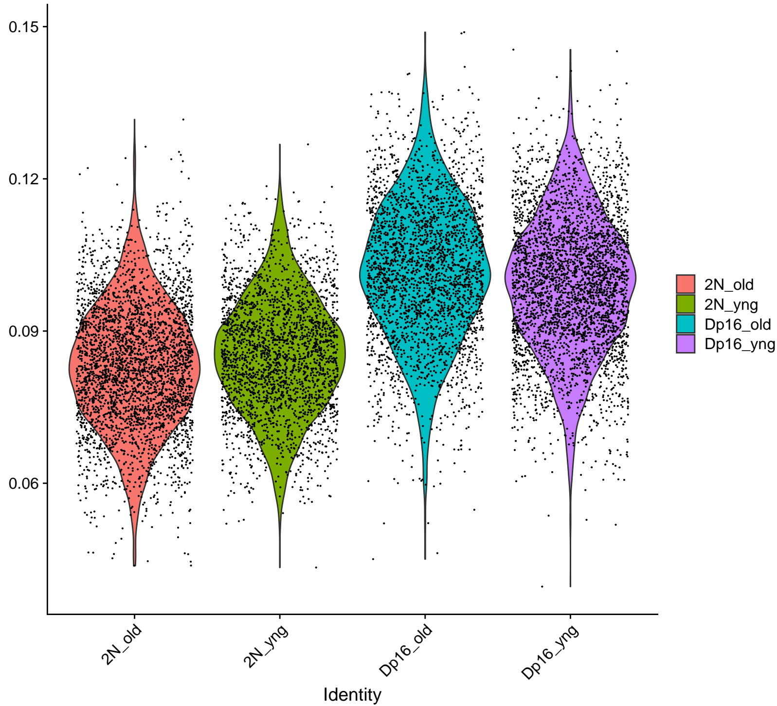
cl1 :Trisomic.Genes.Dp16
