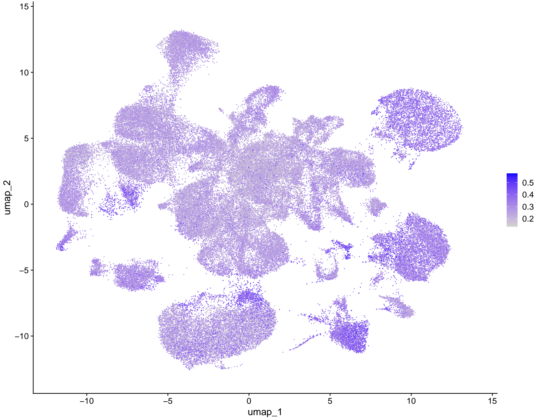
qn.DF.scores
