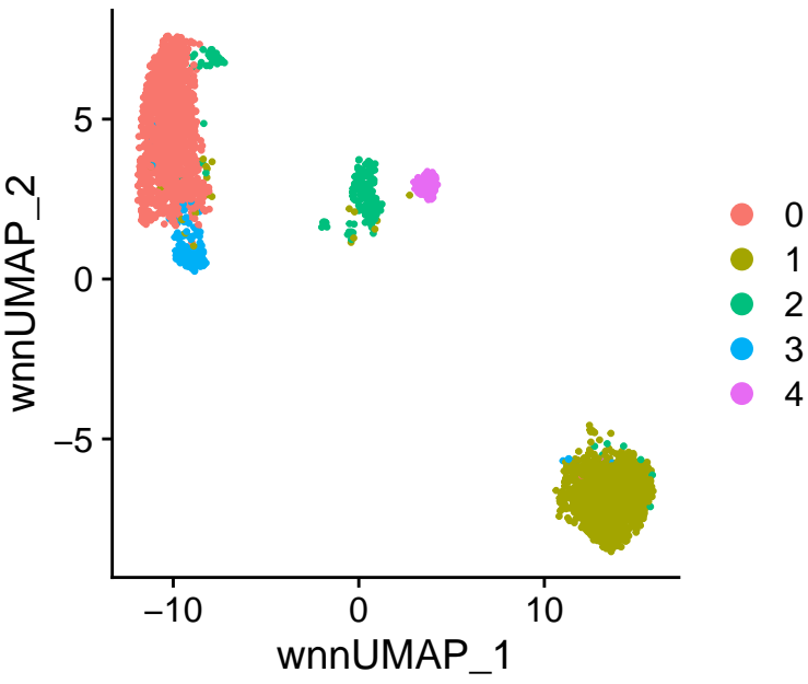
seurat_clusters
