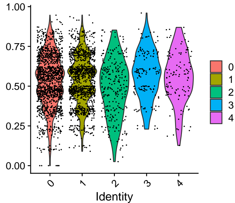
phago_proteo_UCell
