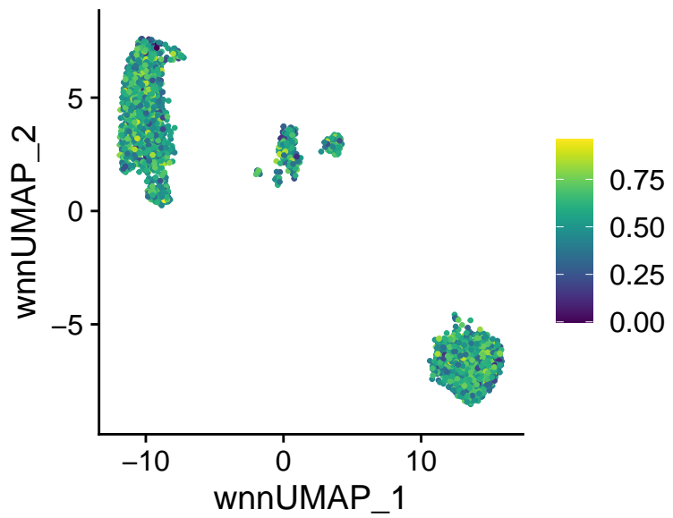
phago_proteo_UCell
