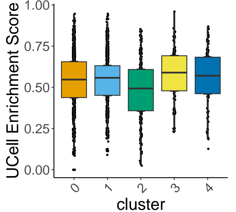
phago_proteo_UCell
