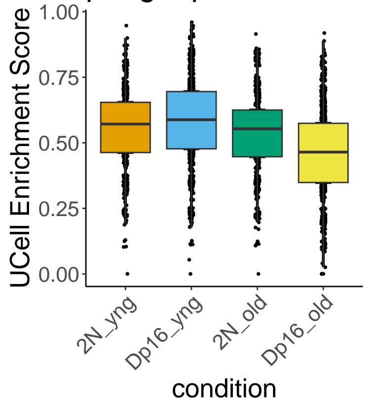
phago_proteo_UCell
