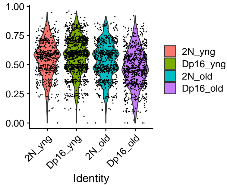
phago_proteo_UCell
