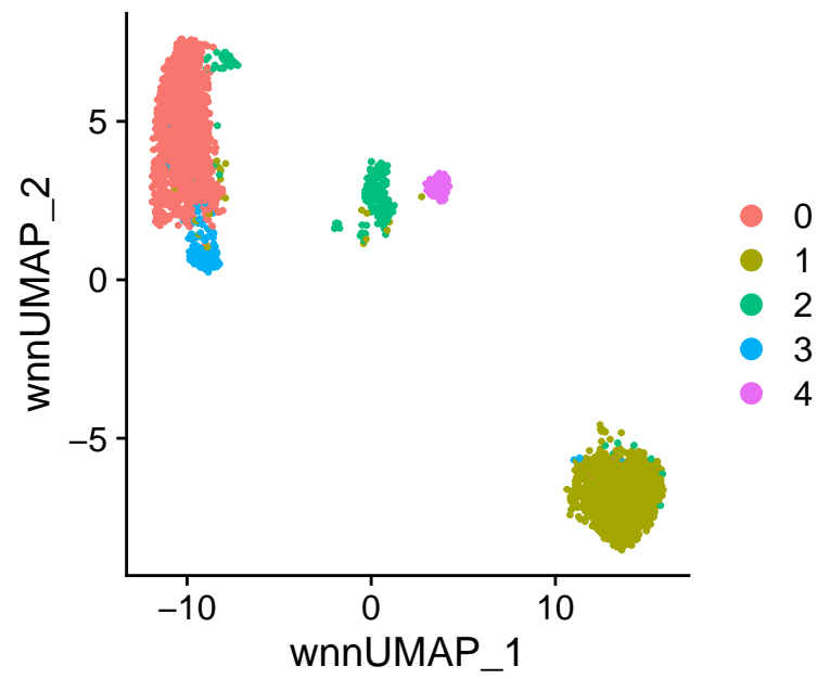
seurat_clusters
