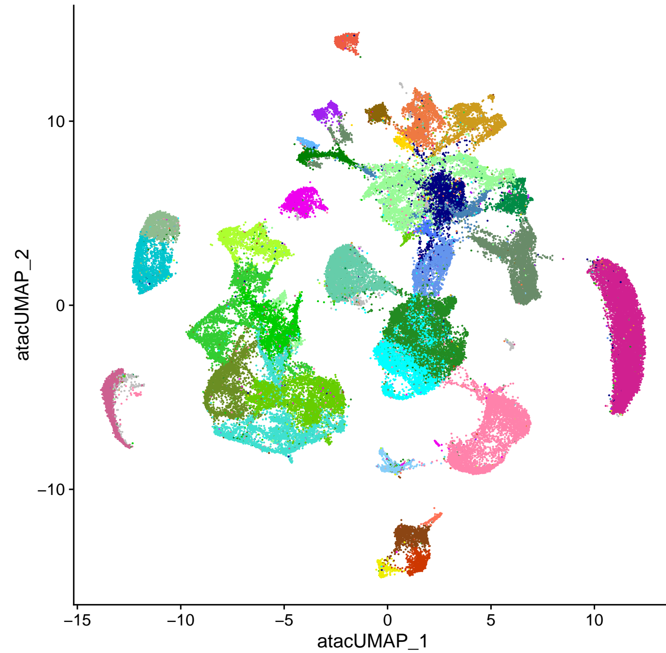
snATAC
