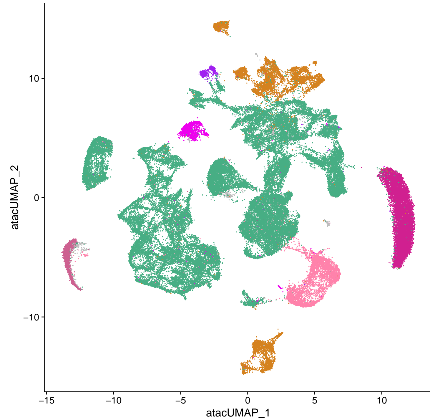
snATAC
