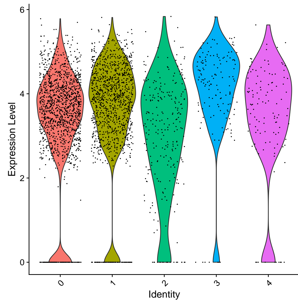
Cts1
