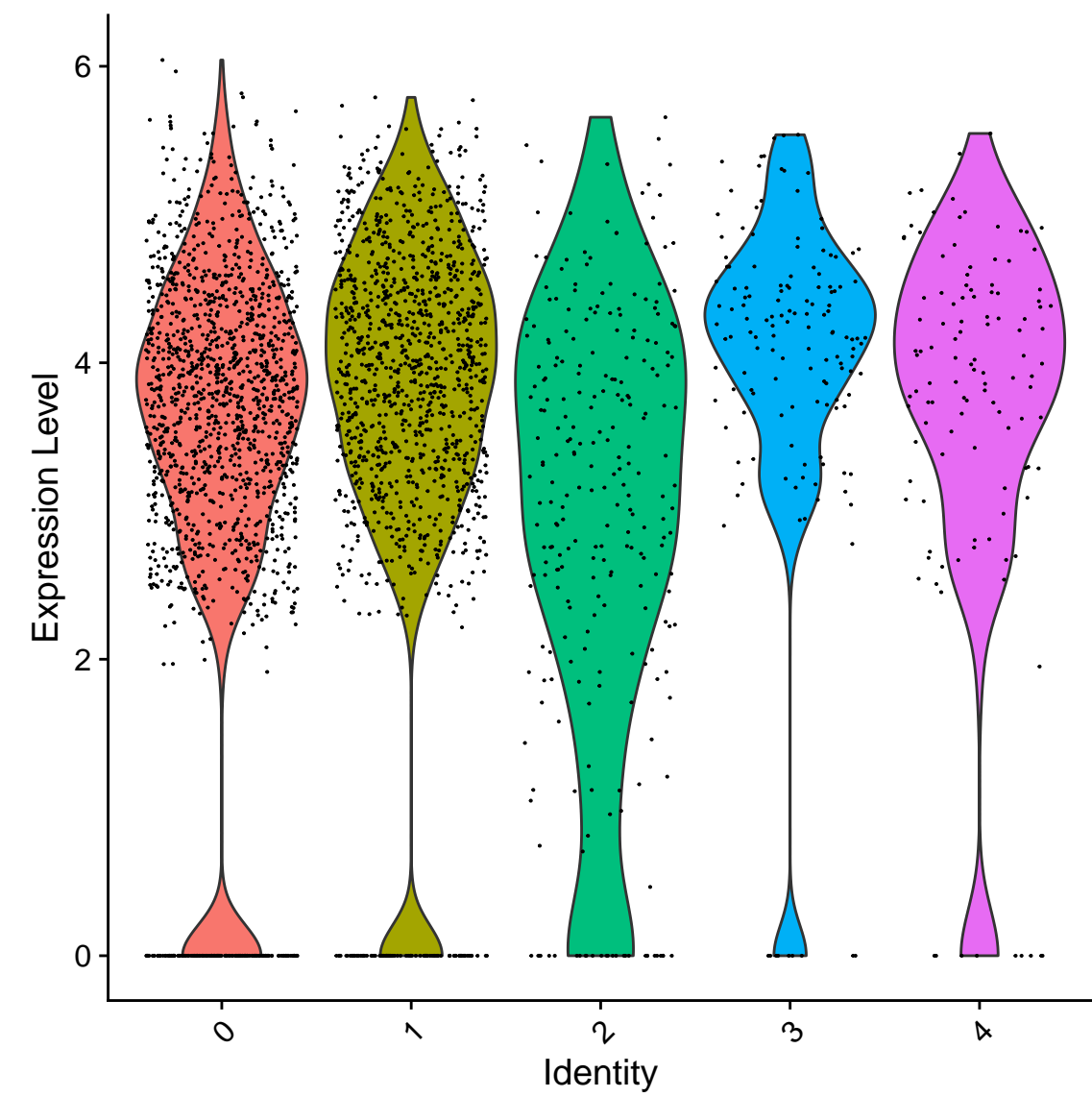
Trem2
