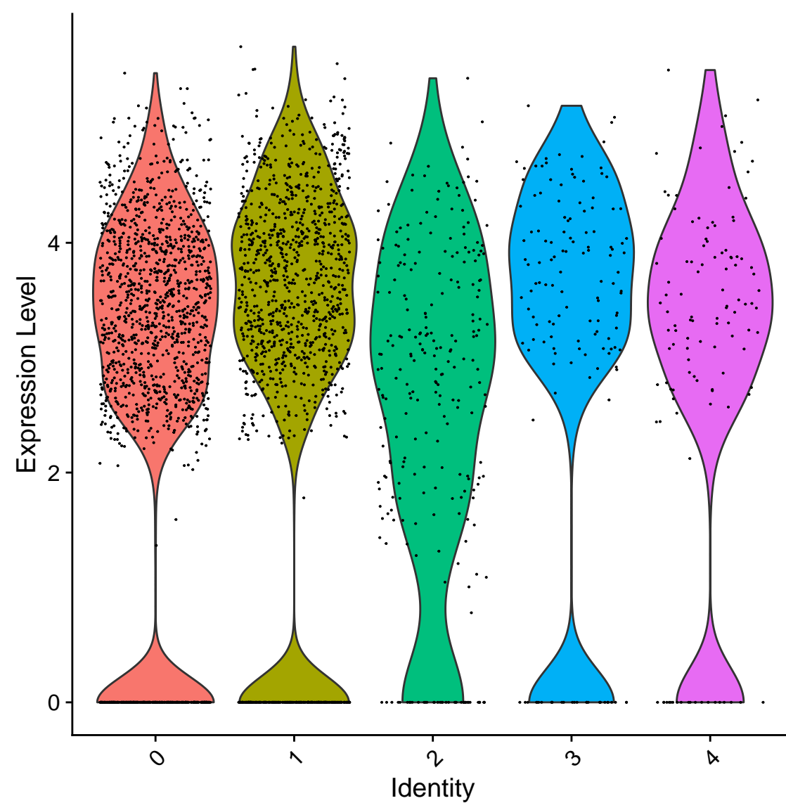
Ctsd
