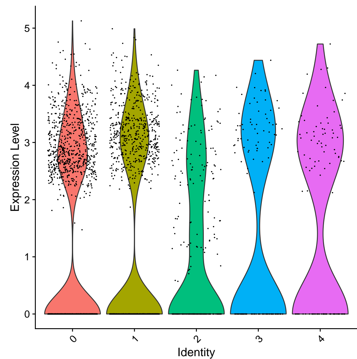
ApoE
