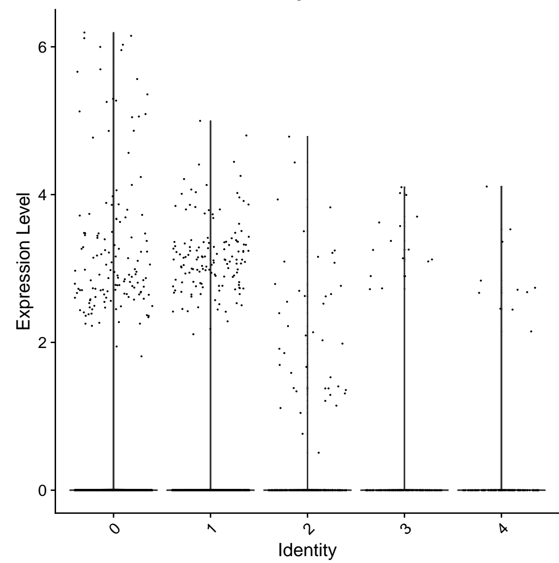
ApoE
