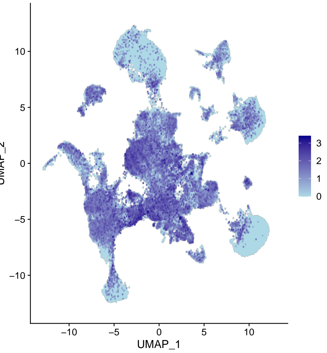
Nrxn1
