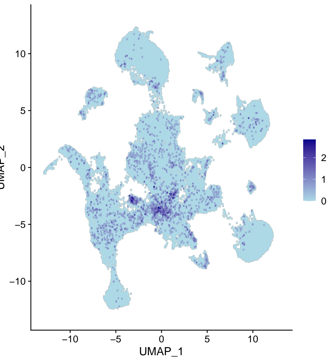
Cntnap5b
