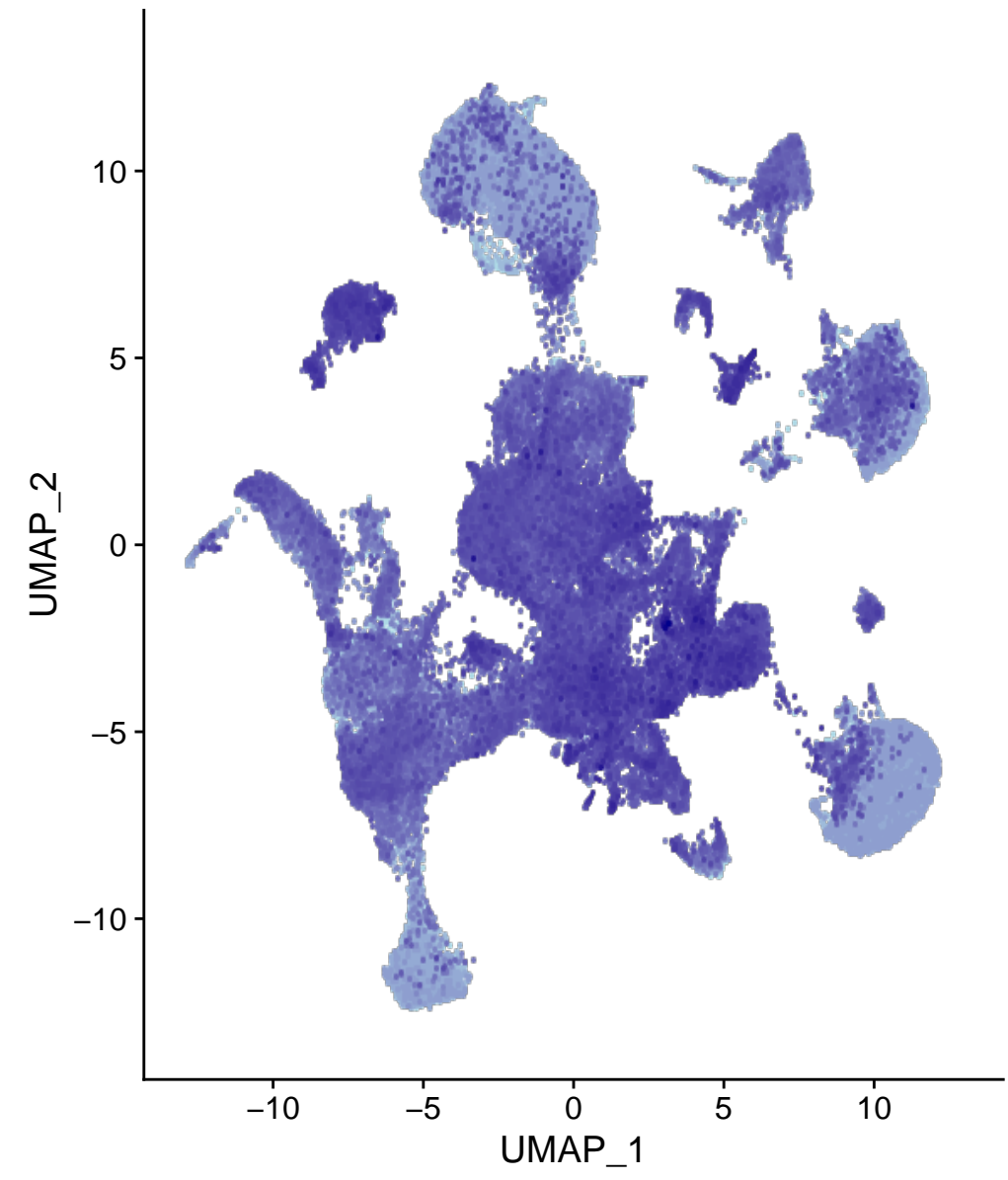
Nrg3
