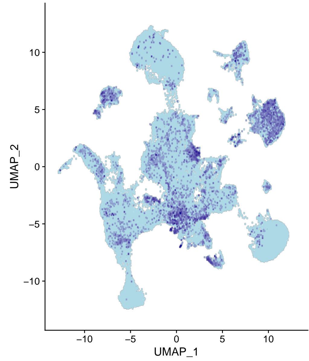
Angpt1
