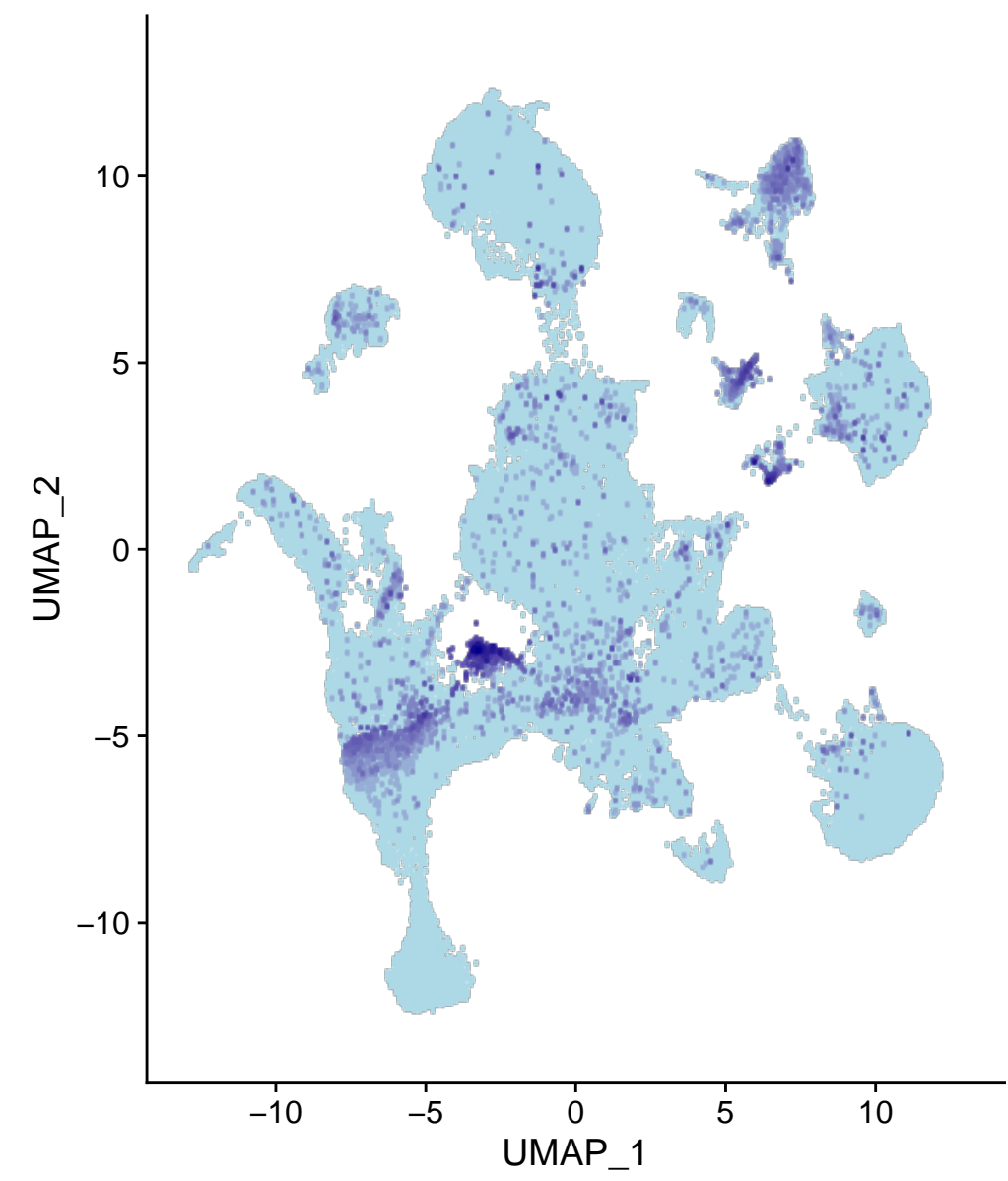
Cntnap2
