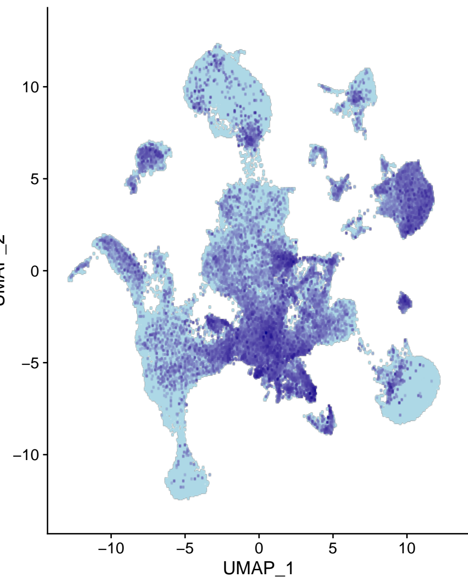
Mgat4c
