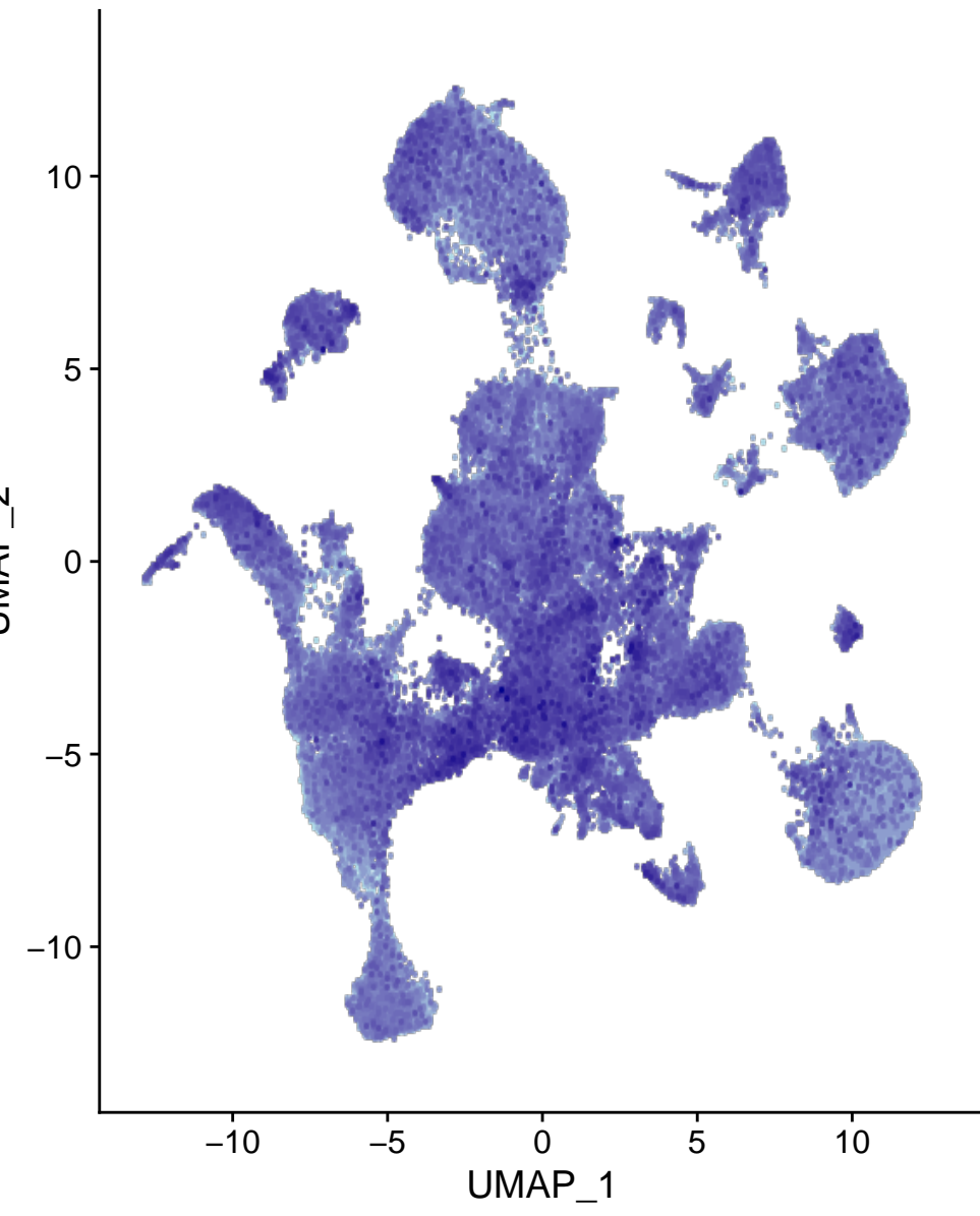
Pde4d
