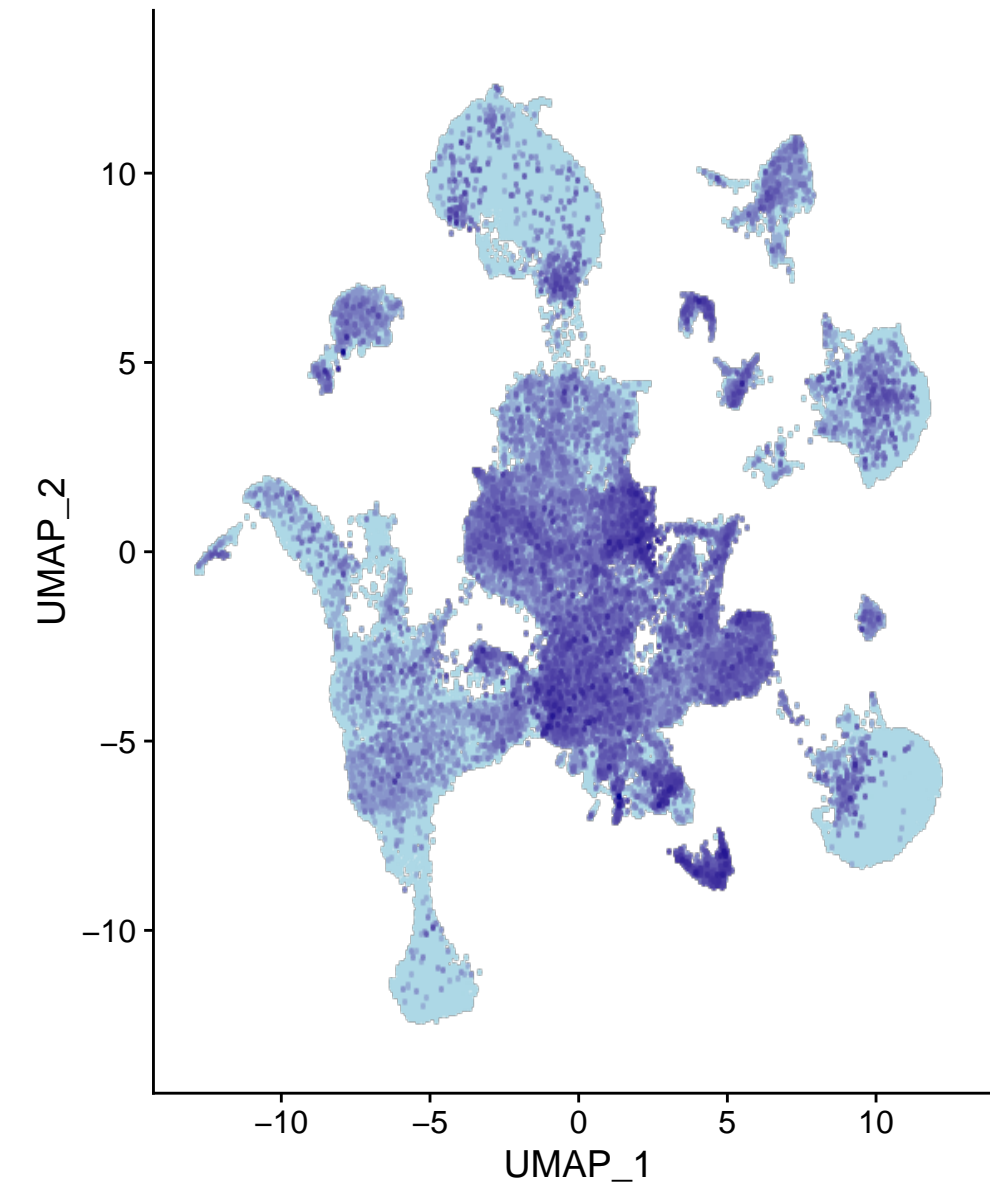
Fstl5
