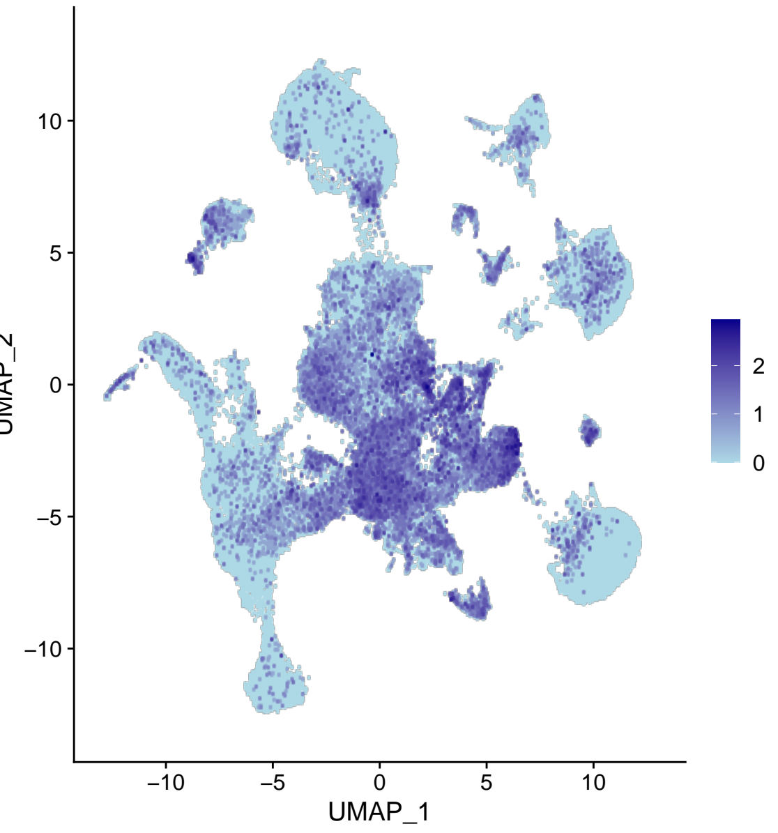
Cntnap4
