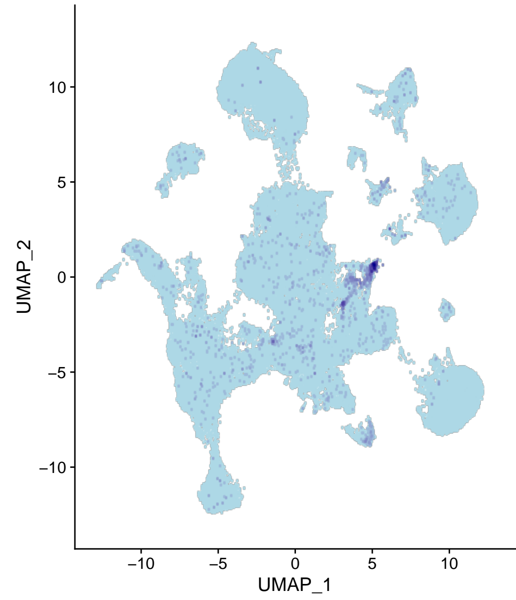
Npy
