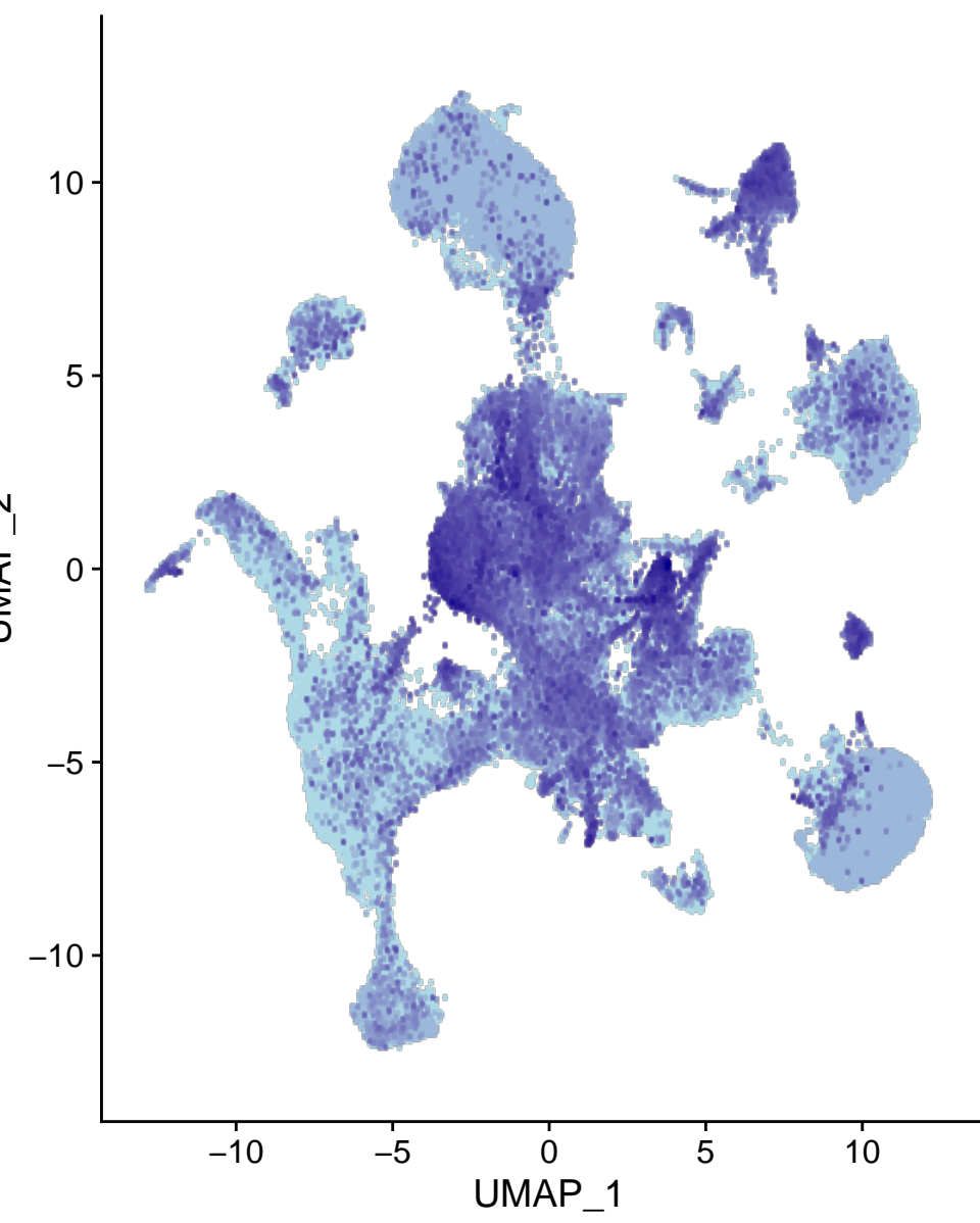
Elavl2
