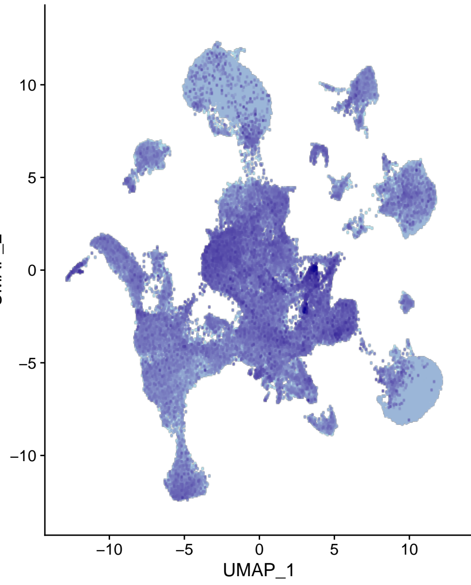
Grip1
