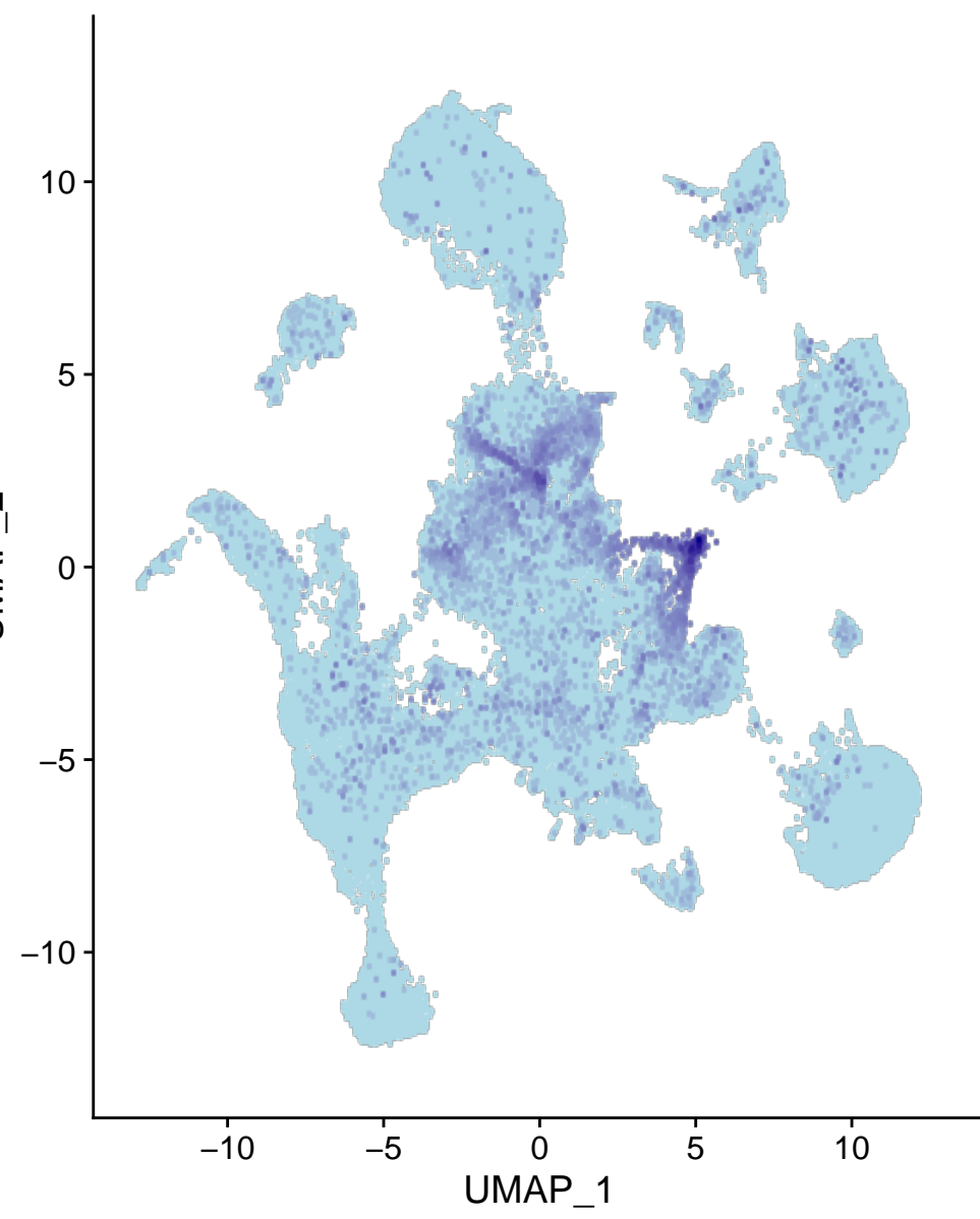
Tcf4
