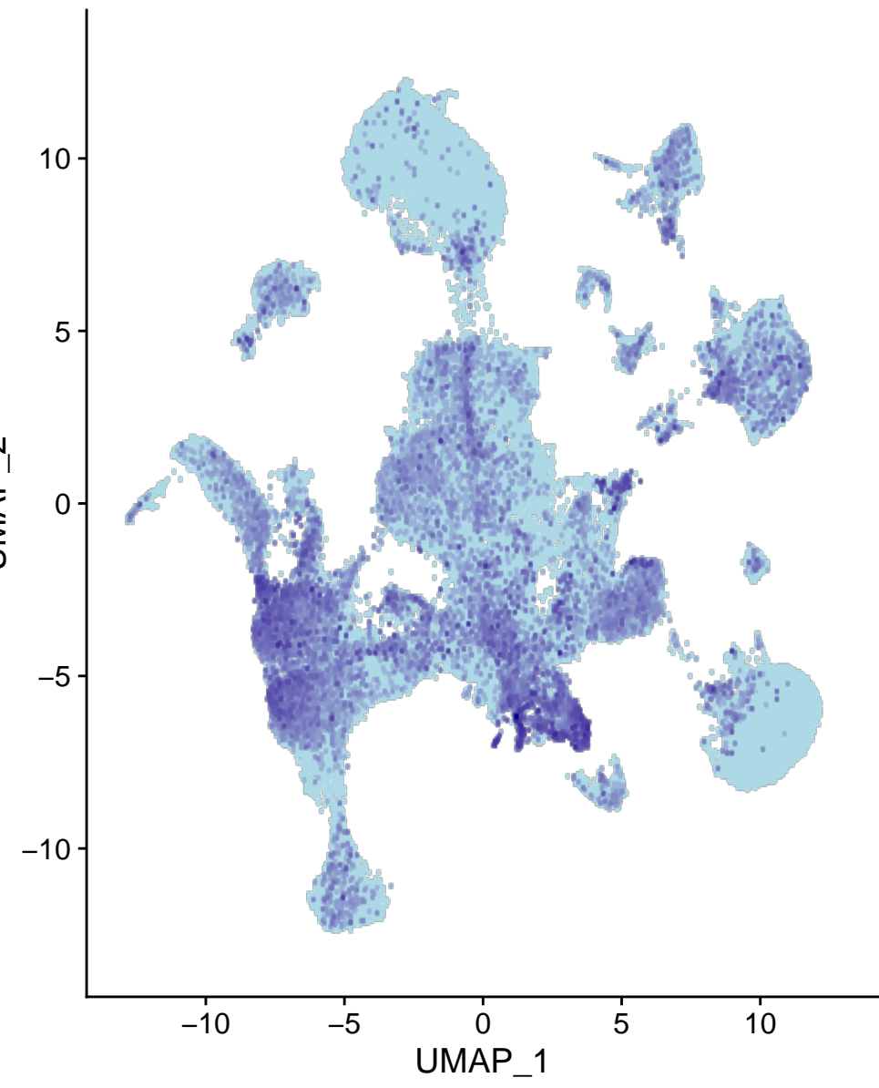
Hs3st4
