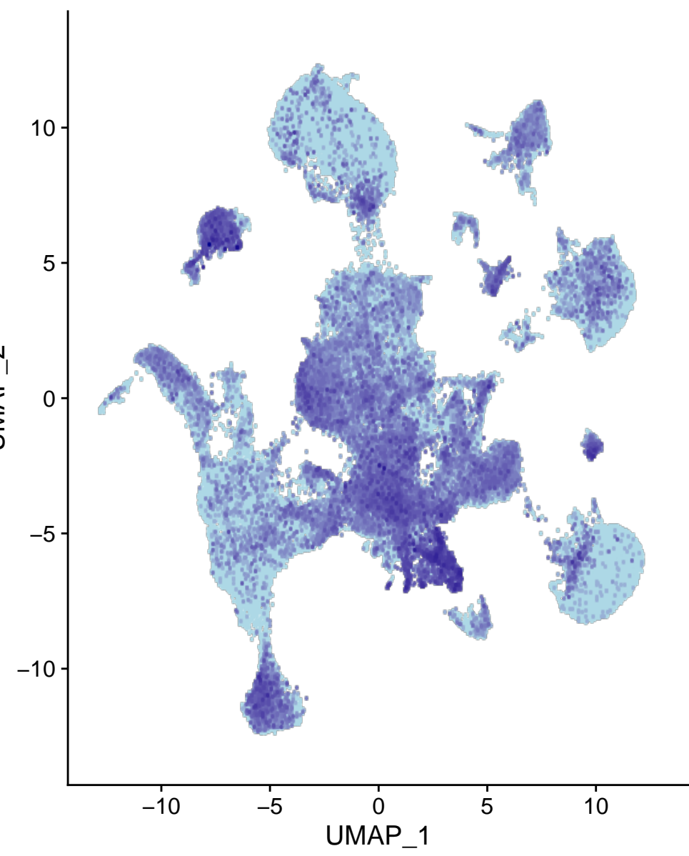
Dach1
