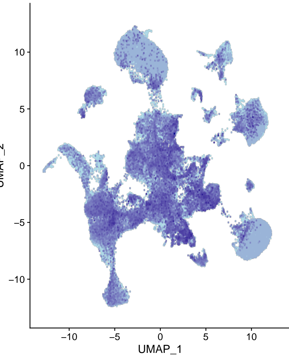
Reln
