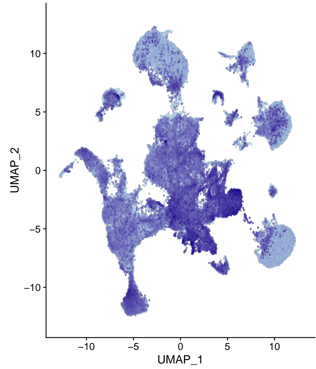
Galnt16
