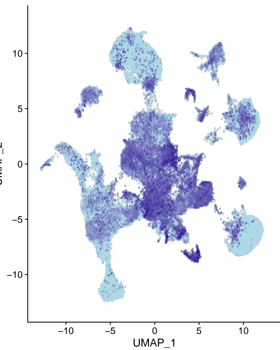
Tcf4
