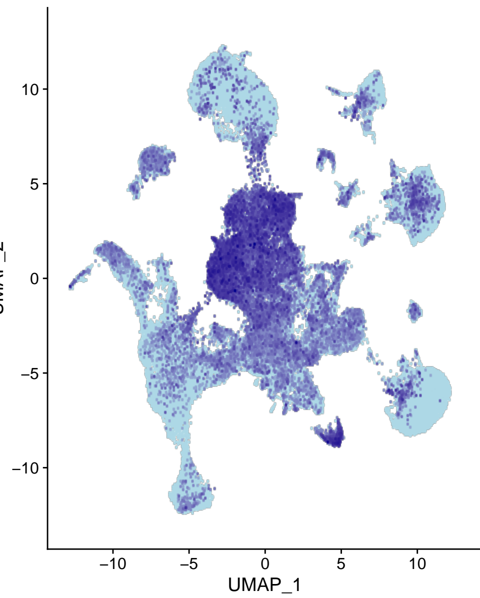
Trpc4
