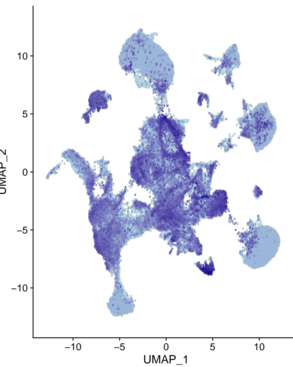
Cpne4
