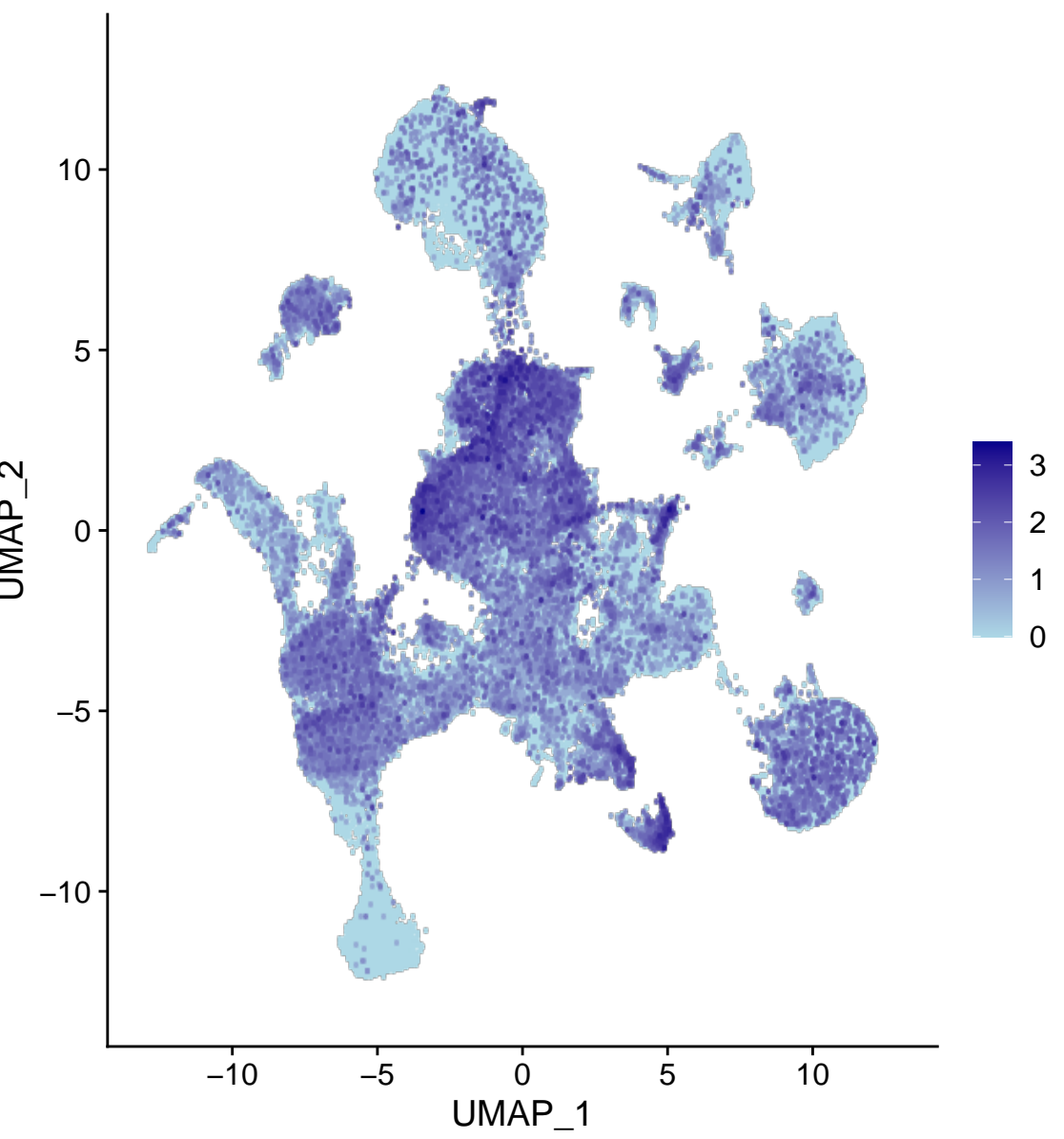
Ii1rapl2
