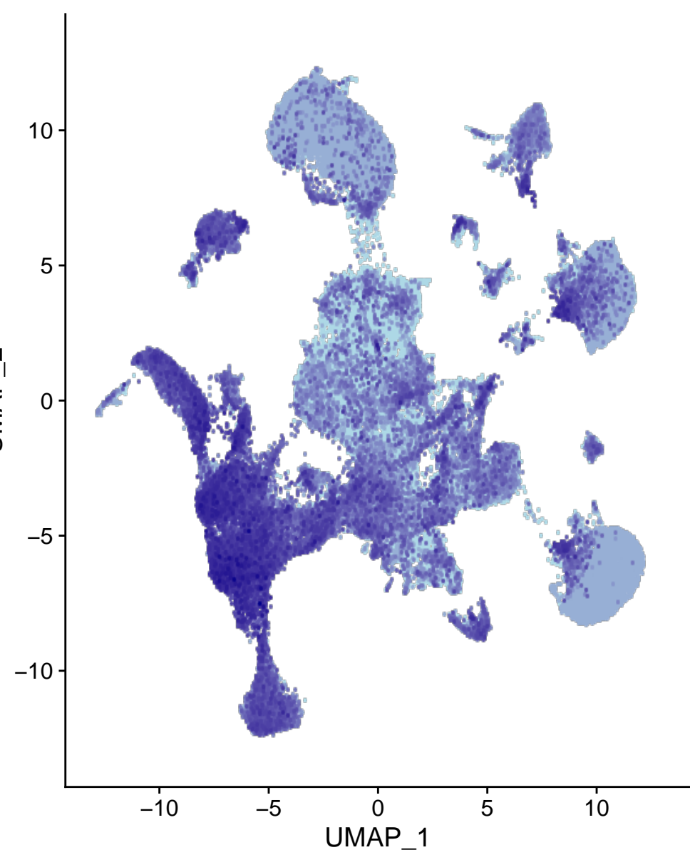
Fstl4
