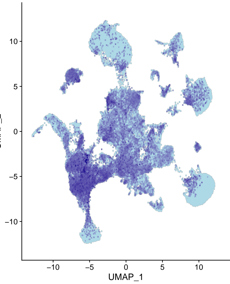
Meis2
