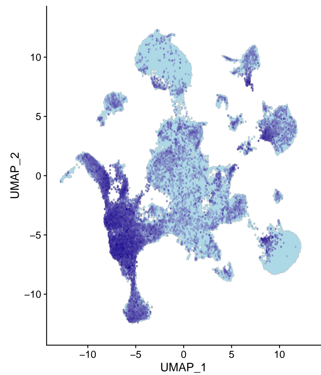
Slit3
