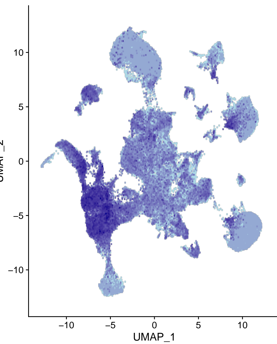
Kcnq5
