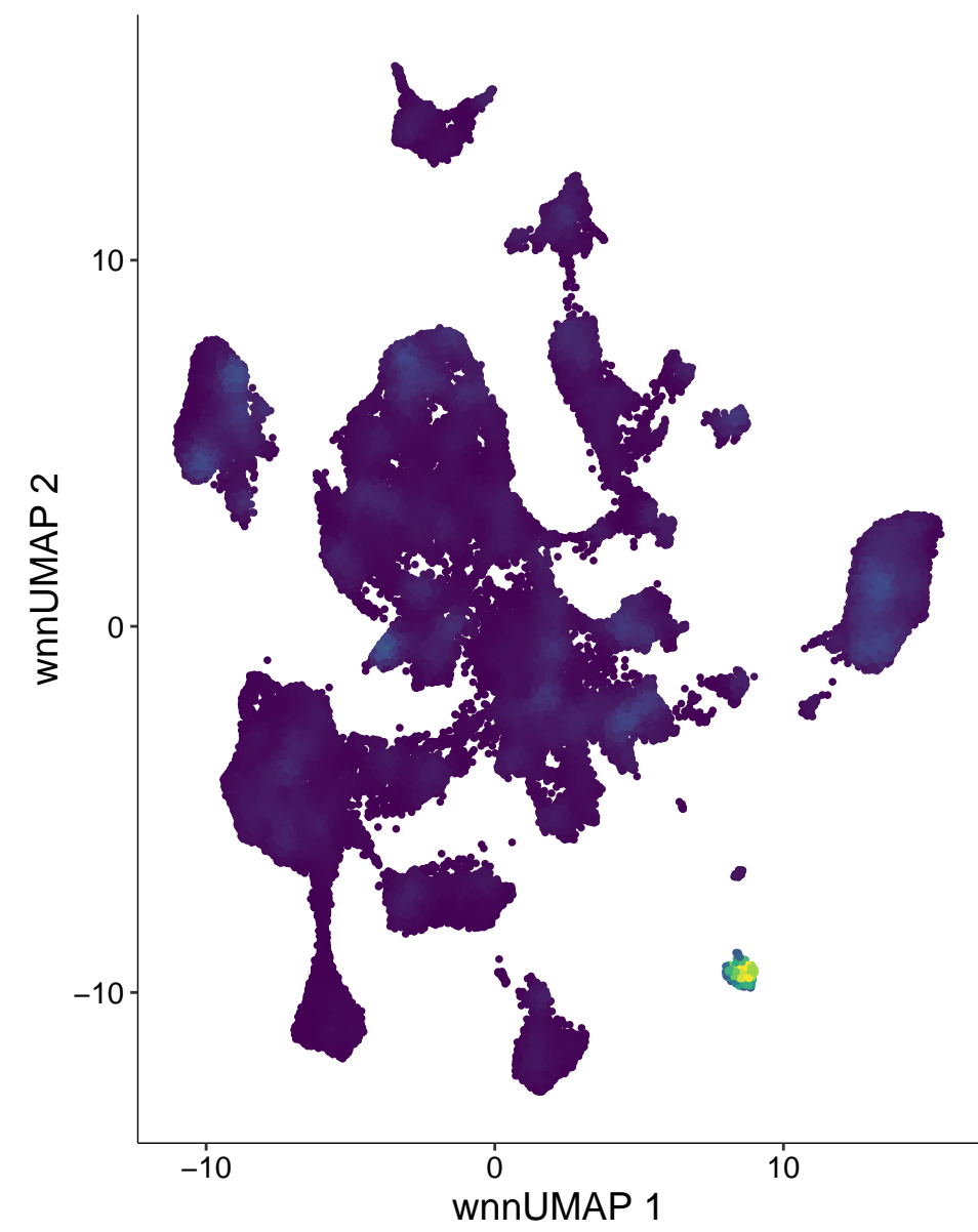
chr9-56700801-56701300
