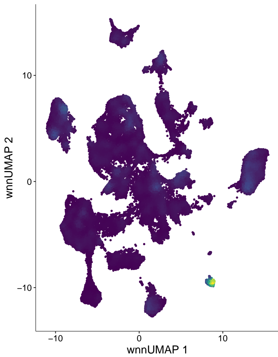
chr15-78082014-78082513
