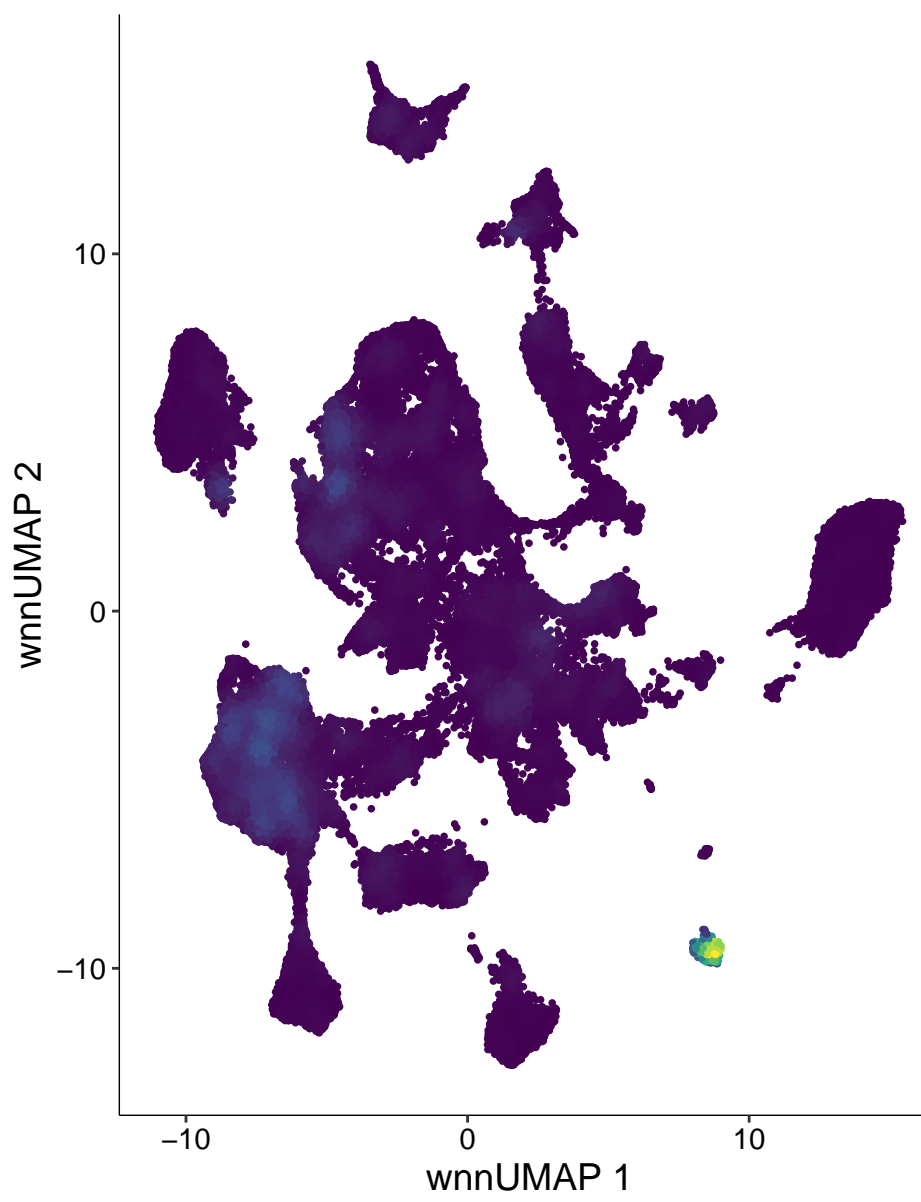
chr5-95978352-95978851
