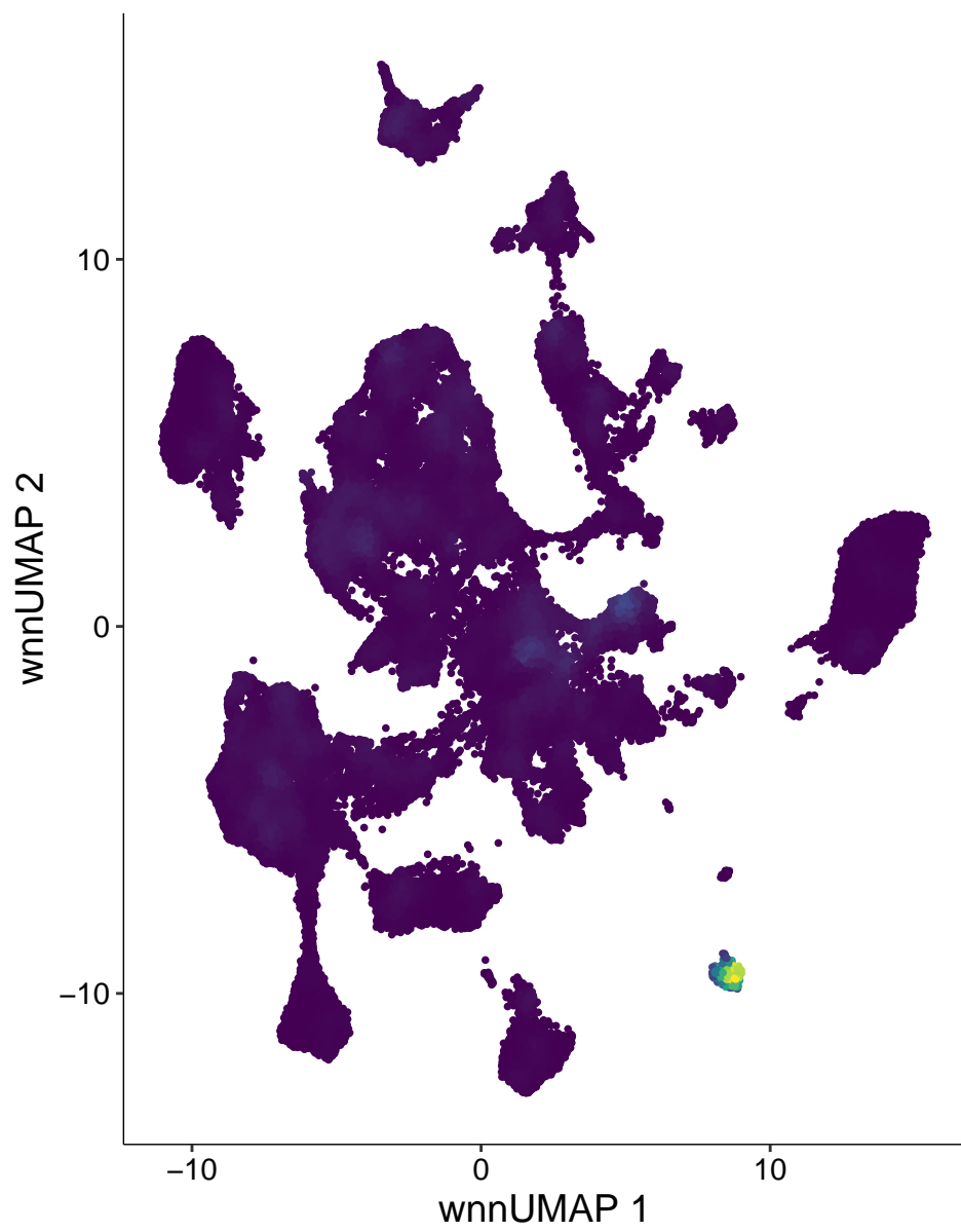
chr1-159358578-159359077
