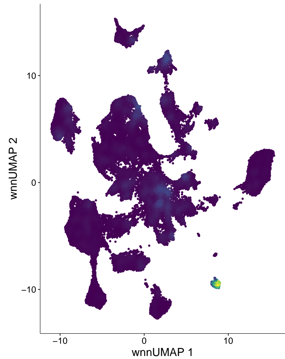
chr17-67451711-67452210
