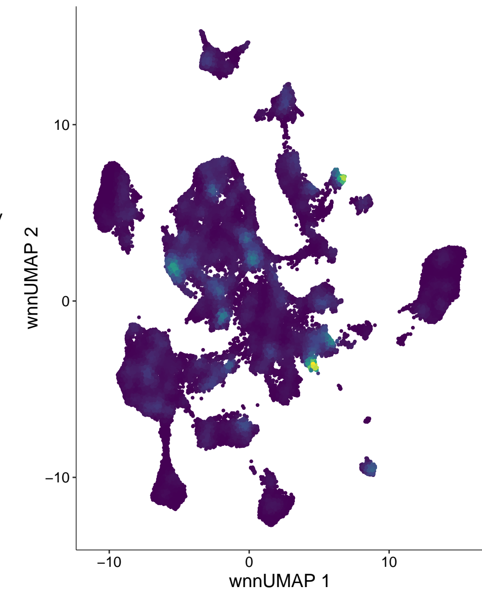
chr8-121458574-121459073
