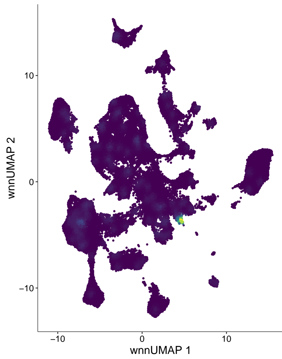
chr10-26228125-26228624
