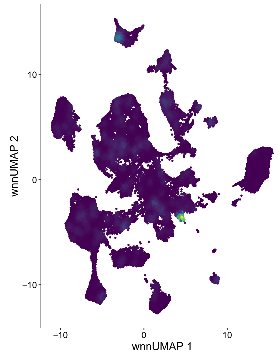
chr14-15681482-15681981
