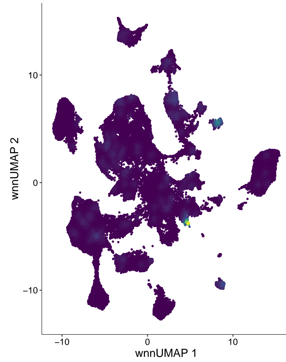
chr9-76829465-76829964
