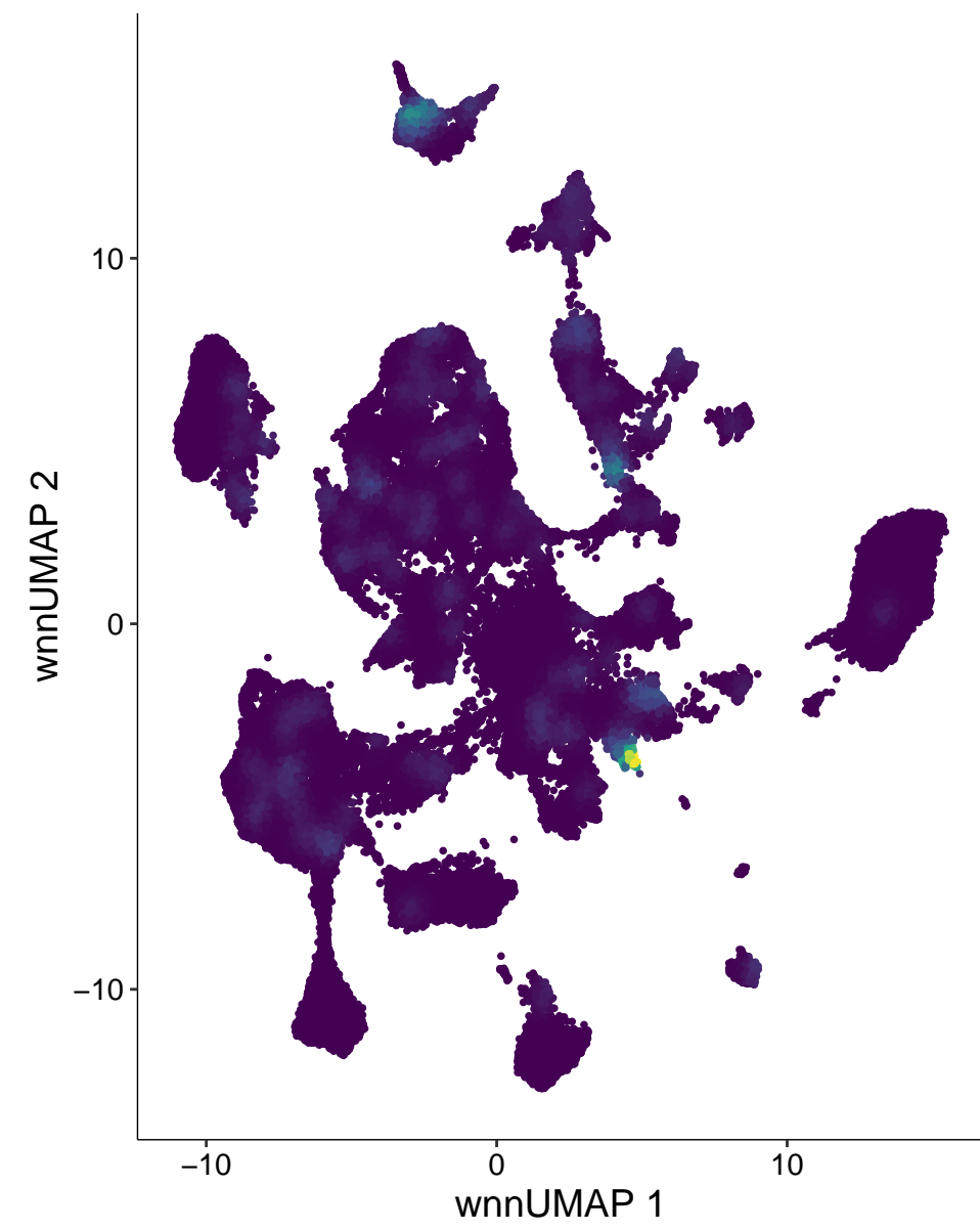
chr6-11583527-11584026
