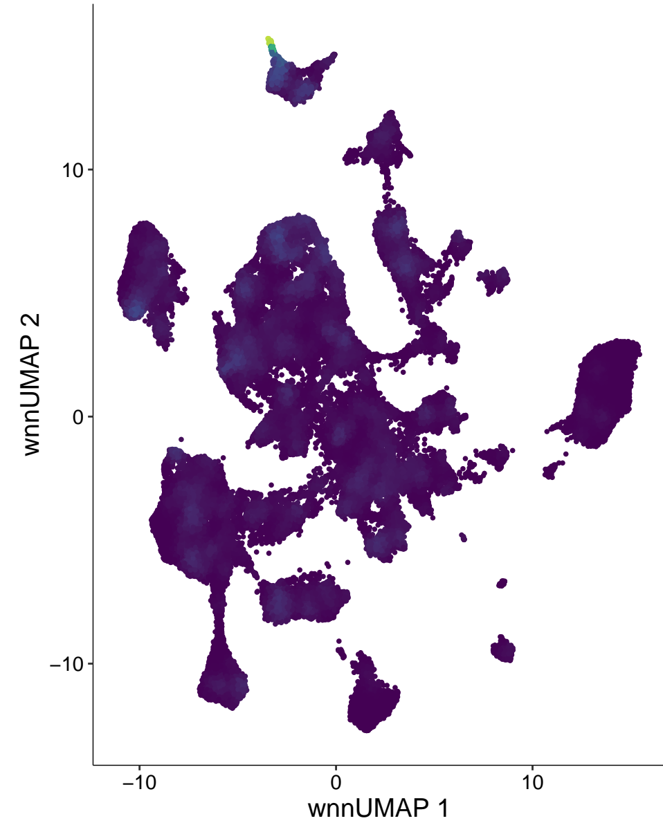
chr15-87538692-87539191
