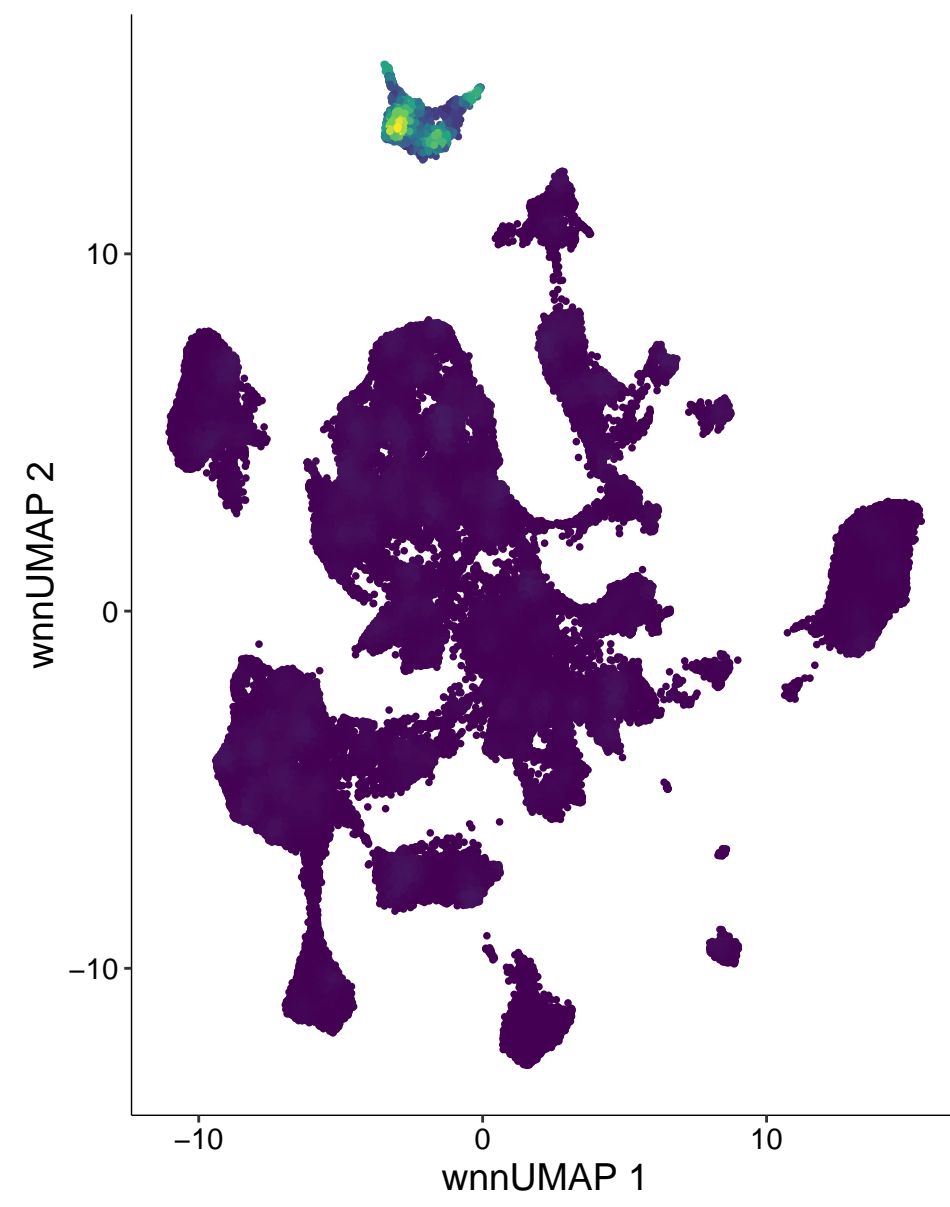
chr6-39797040-39797539
