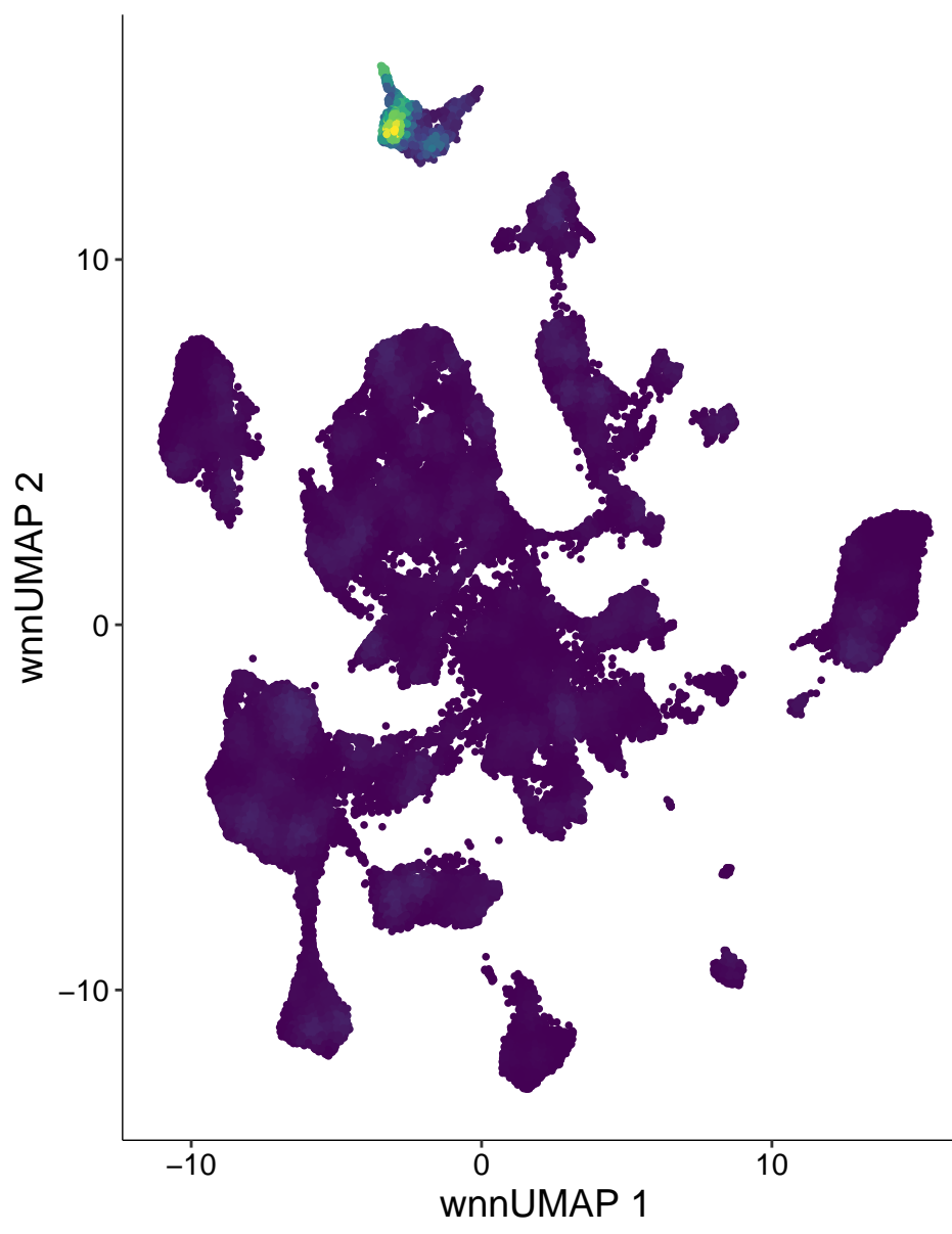
chr14-56173307-56173806
