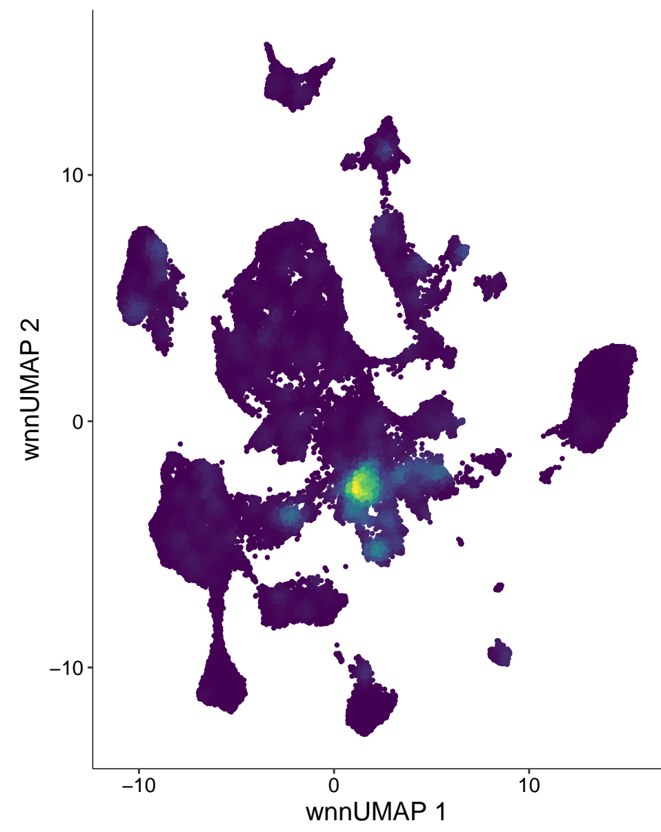
chr6-5807643-5808142
