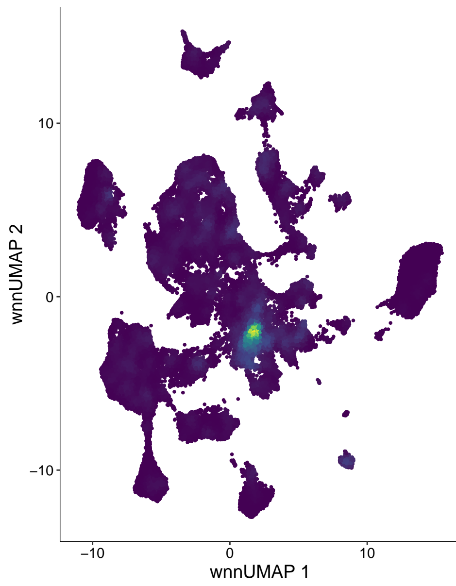
chr12-27444963-27445462
