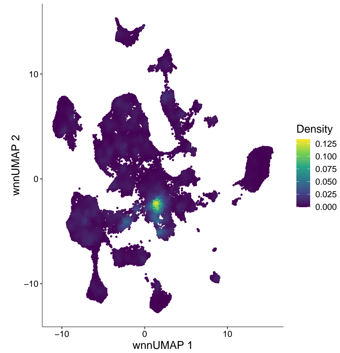
chr1-38852129-38852628
