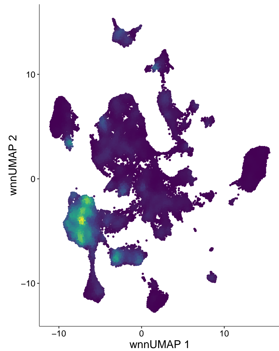
chr2-152321752-152322251
