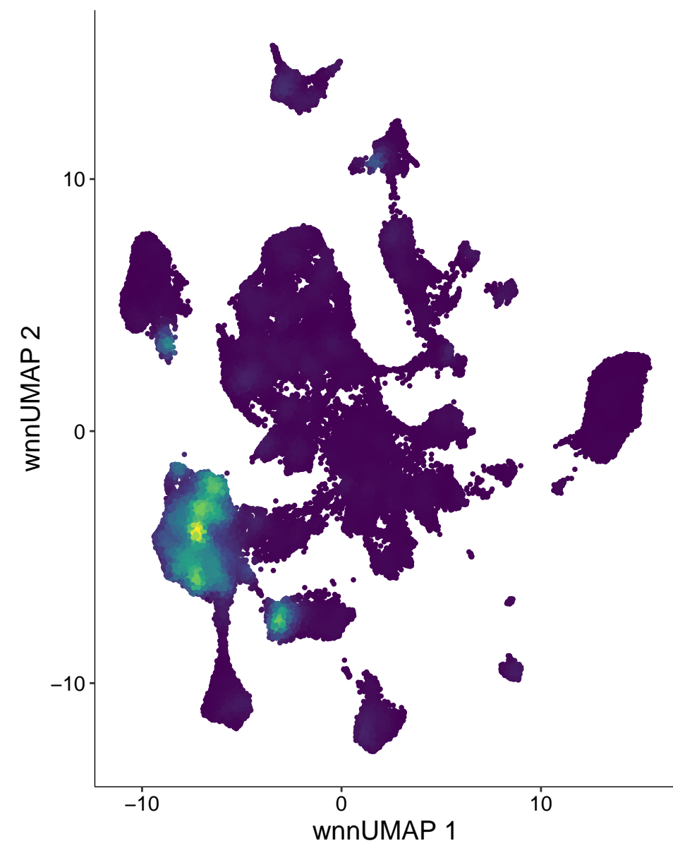
chr9-66752687-66753186
