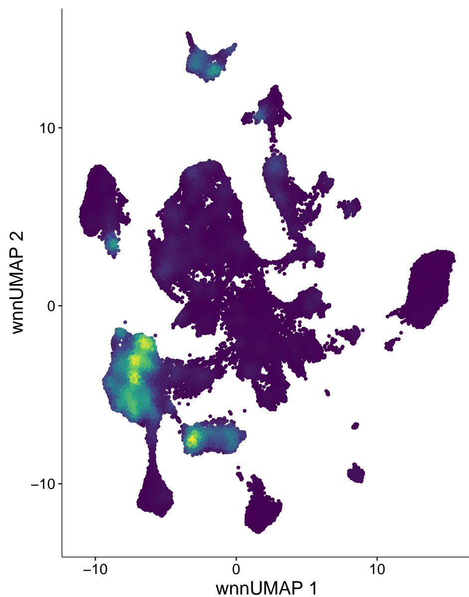
chr4-102148686-102149185
