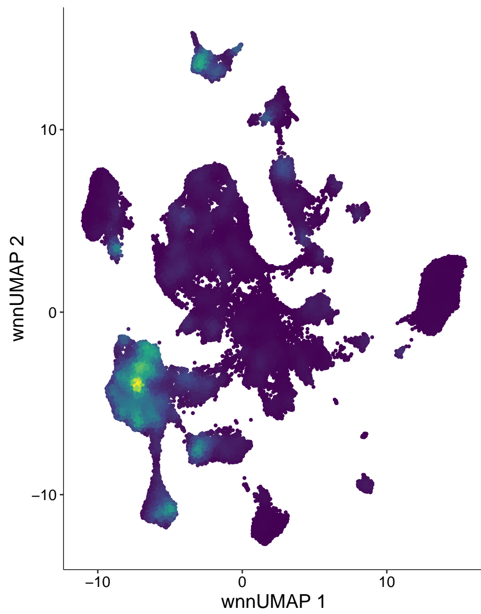
chr18-74921581-74922080
