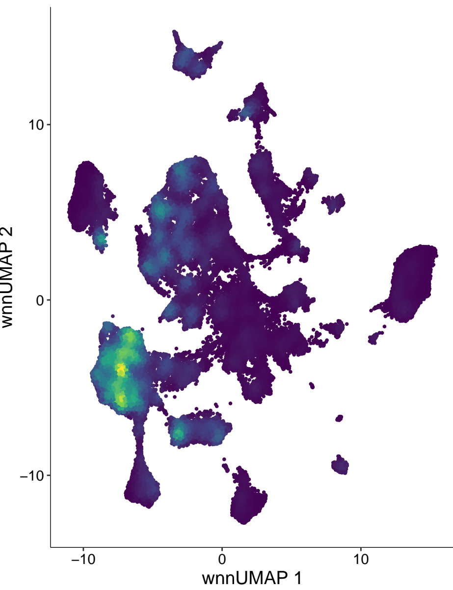
chr4-142633900-142634399
