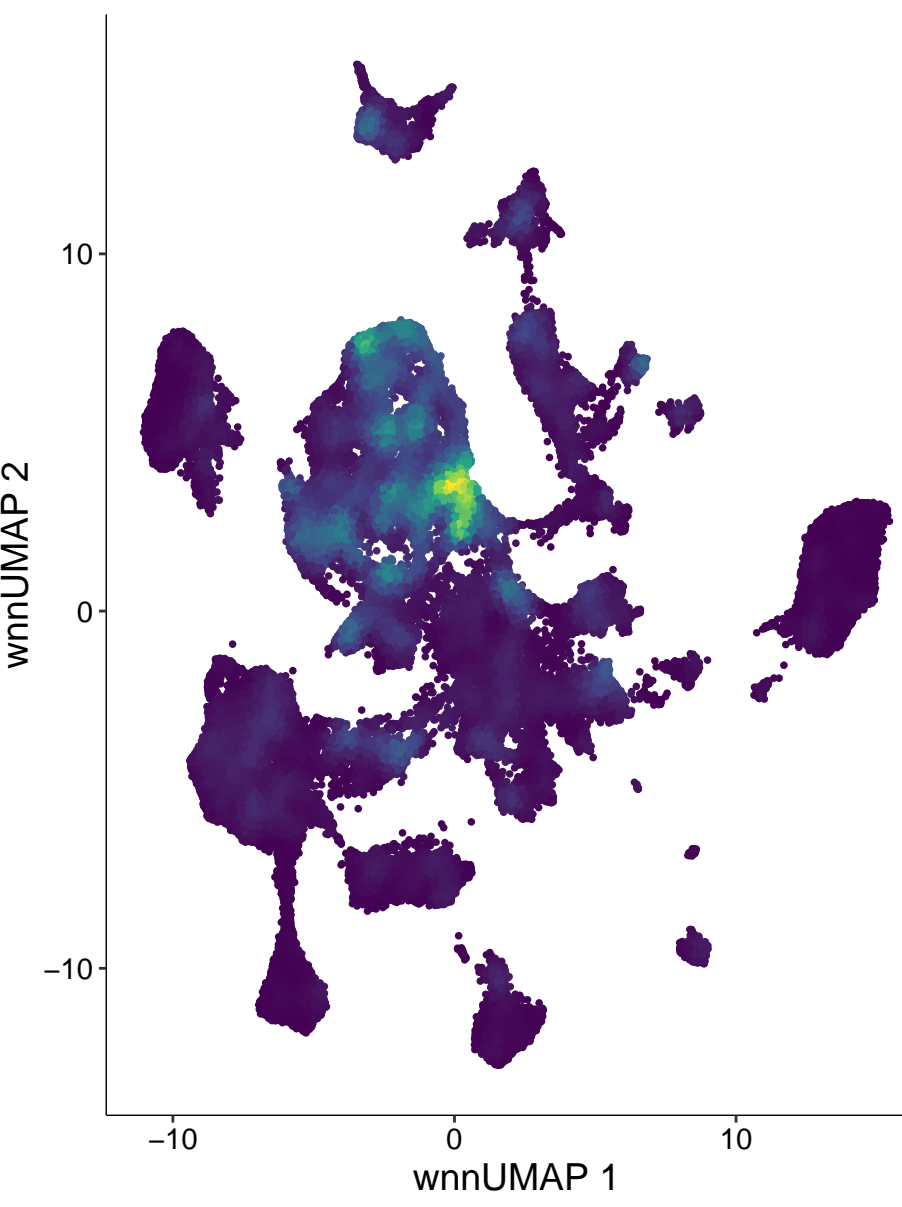
chr12-25672758-25673257
