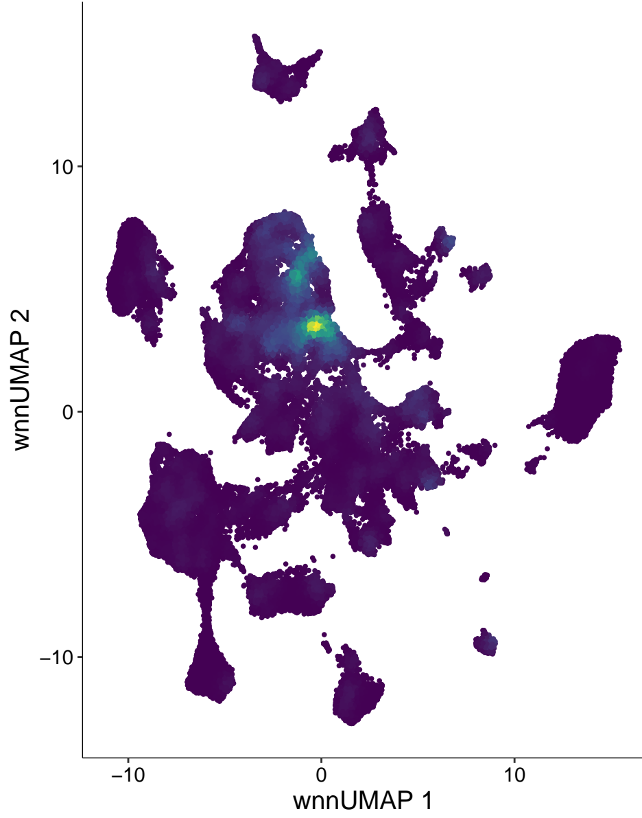
chr9-44531904-44532403
