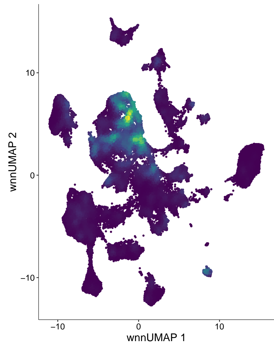
chr4-73517411-73517910
