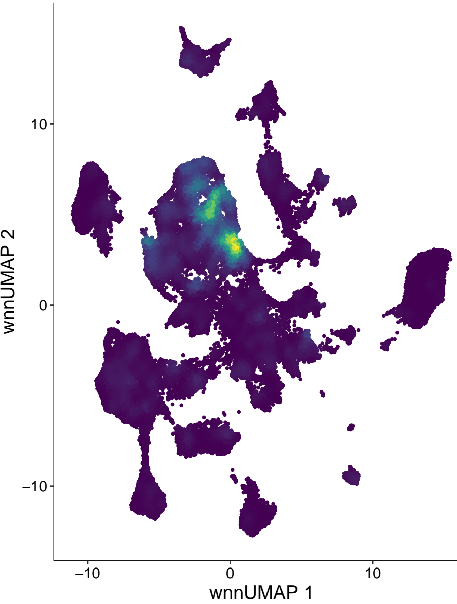
chr4-40499784-40500283
