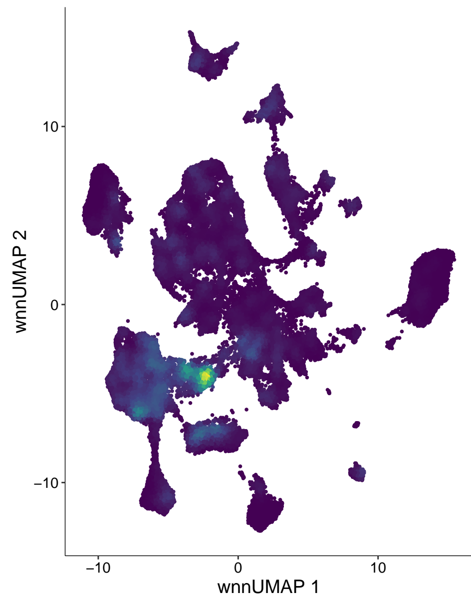
chr1-167328680-167329179
