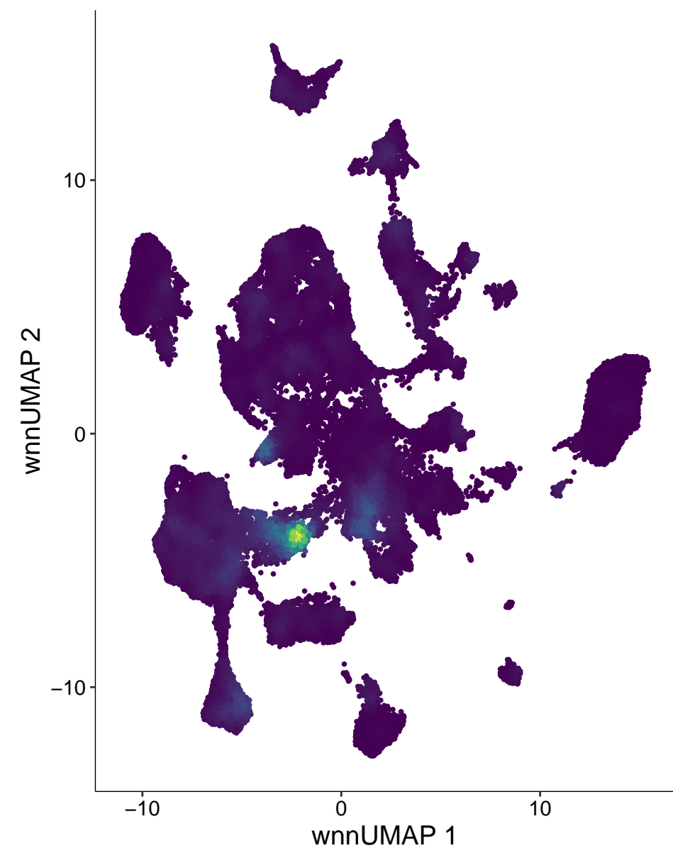
chr6-84700507-84701006
