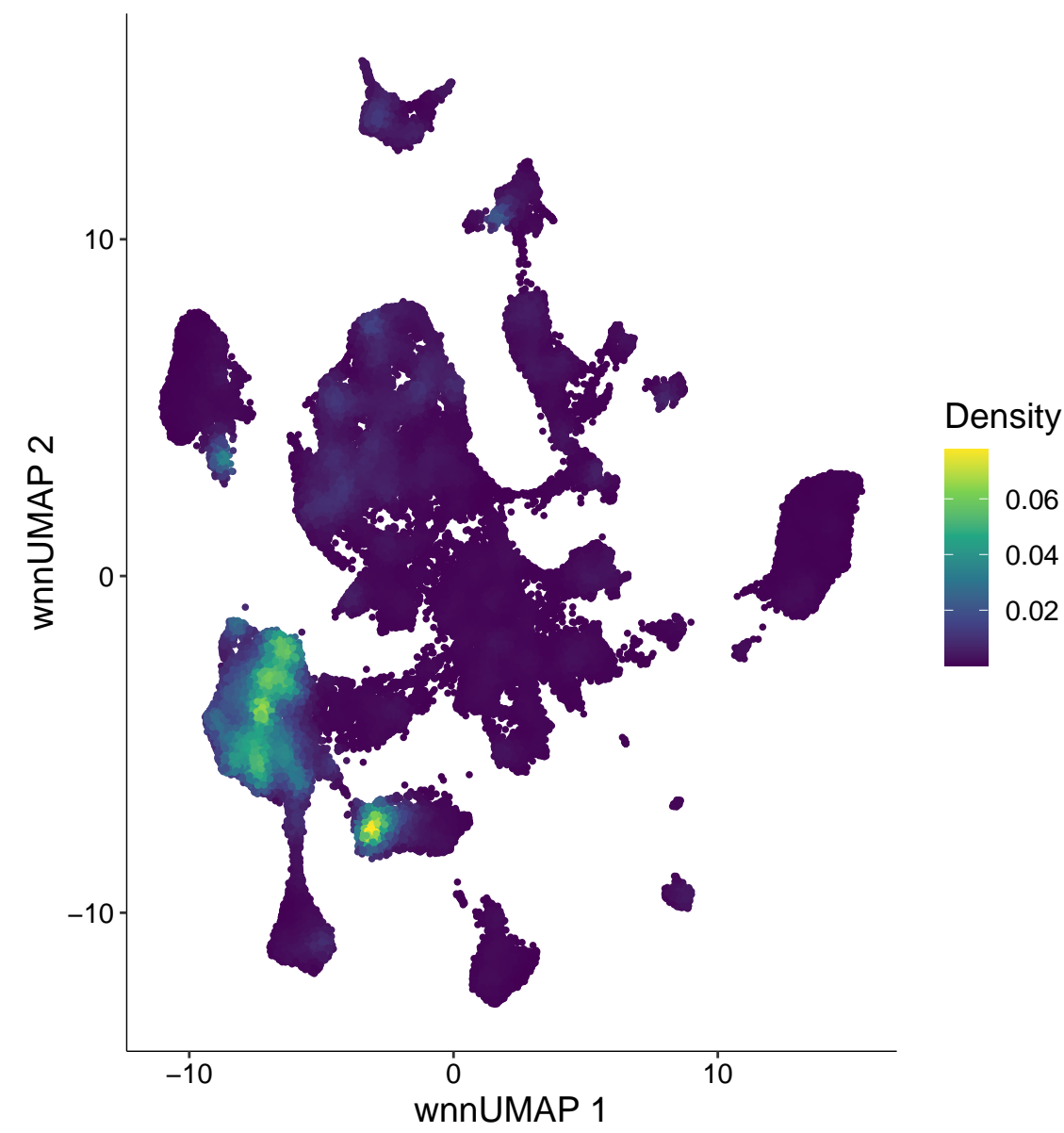
chr15-75781878-75782377
