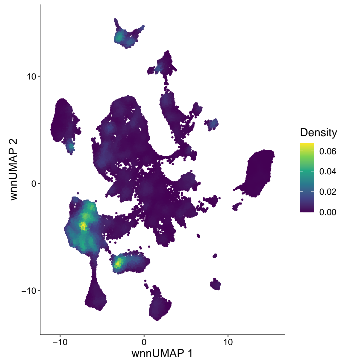
chr6-82437161-82437660
