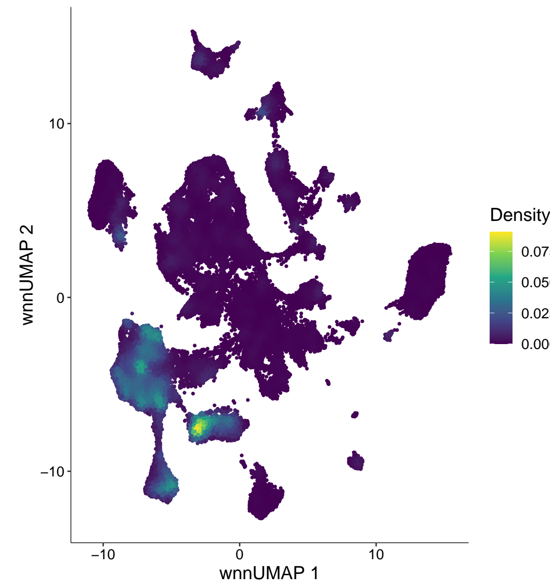
chr6-78552273-78552772
