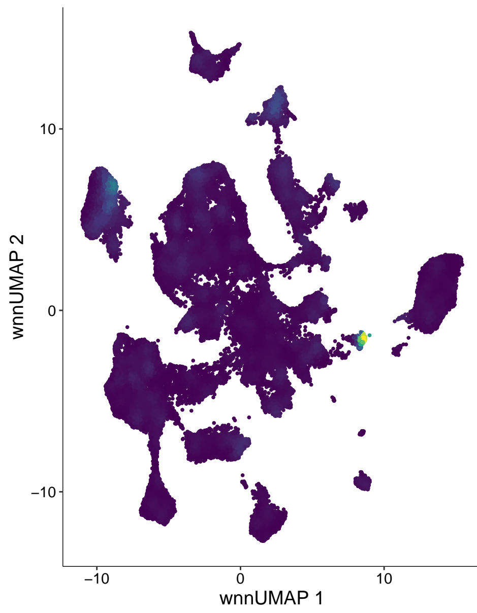
chr2-132449268-132449767
