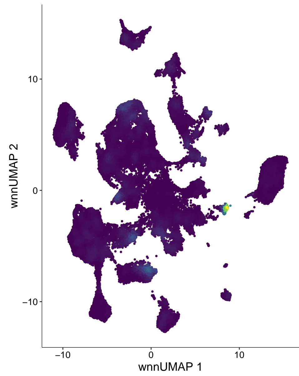
chr10-96747156-96747655
