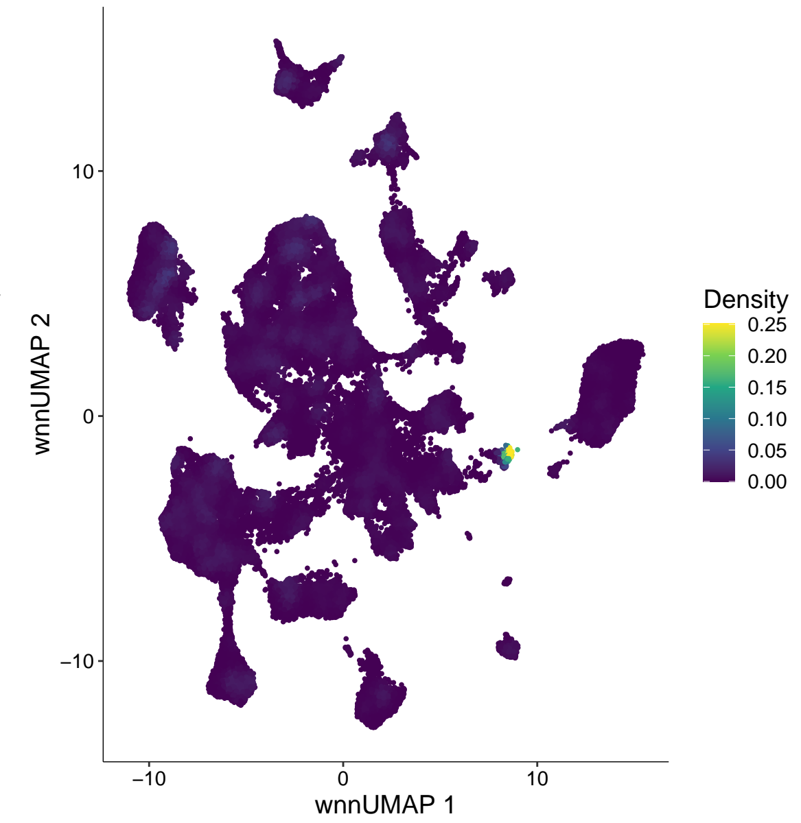
chr6-127443952-127444451
