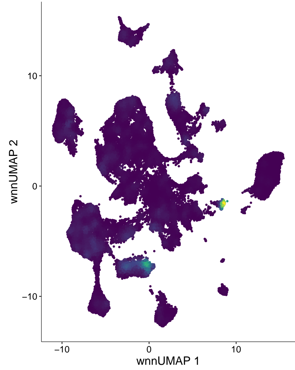
chr8-90536090-90536589
