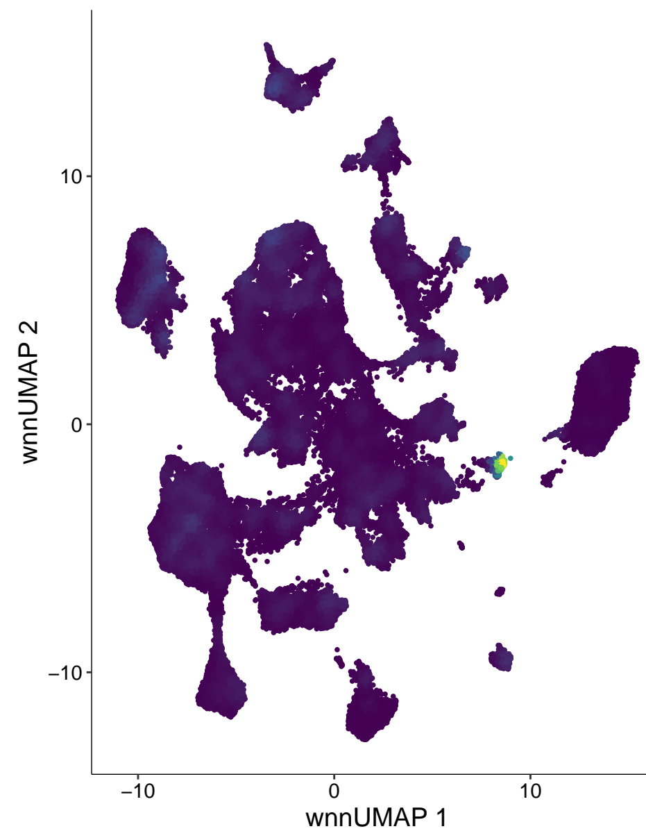
chr16-89429476-89429975
