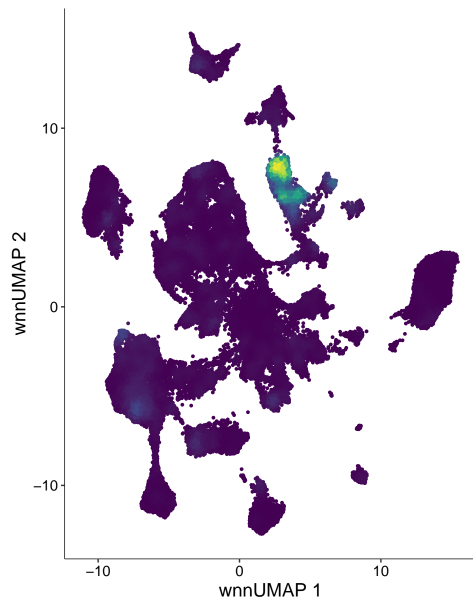
chr16-50174350-50174849
