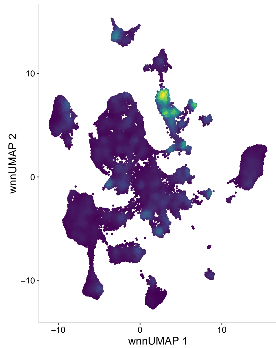
chr4-103535309-103535808
