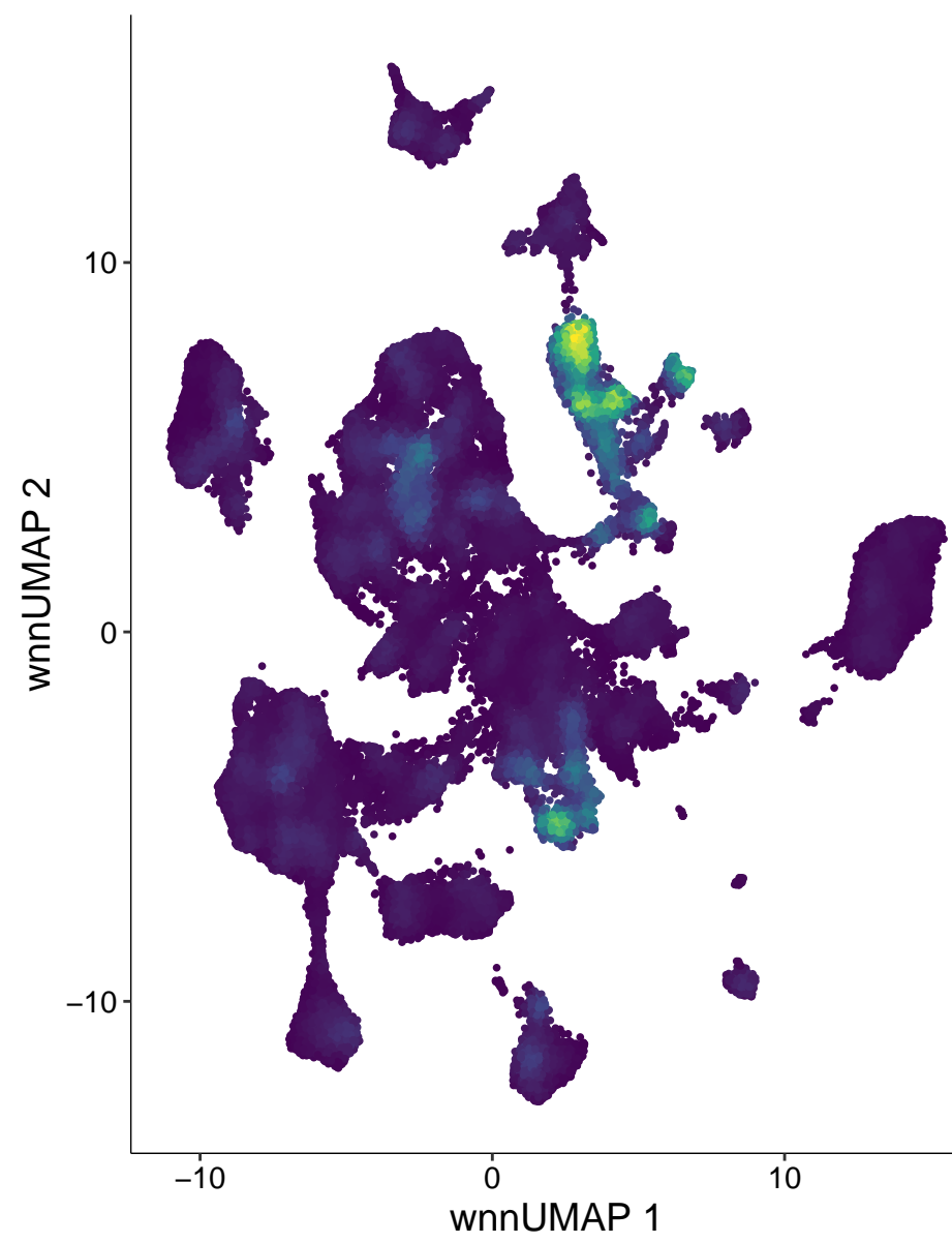
chr5-24484882-24485381
