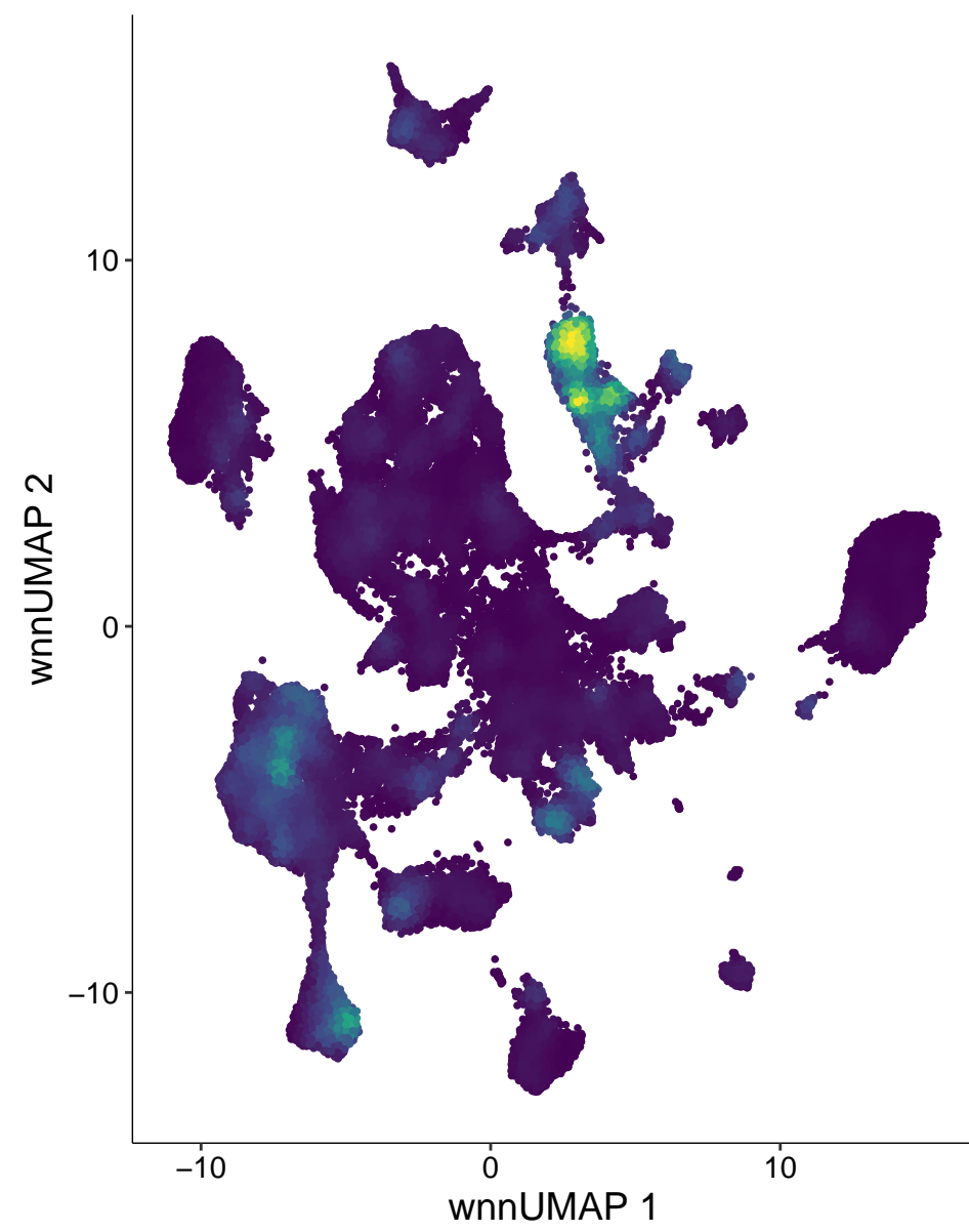
chr4-136905018-136905517
