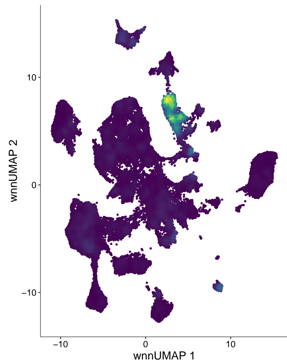
chr13-57637666-57638165
