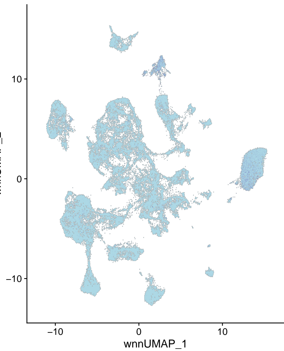
chr16-91191672-91192171
