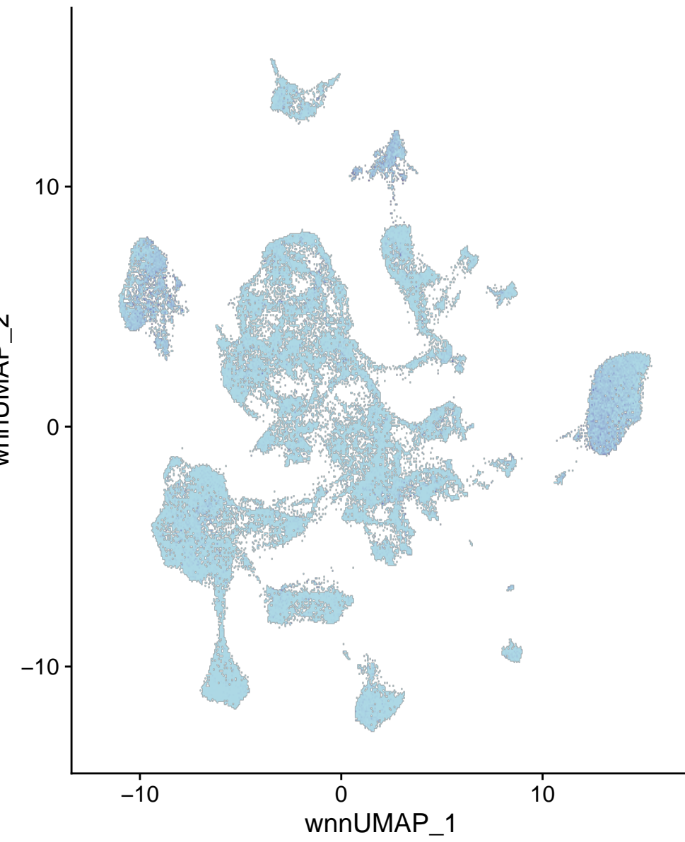
chr4-22488251-22488750
