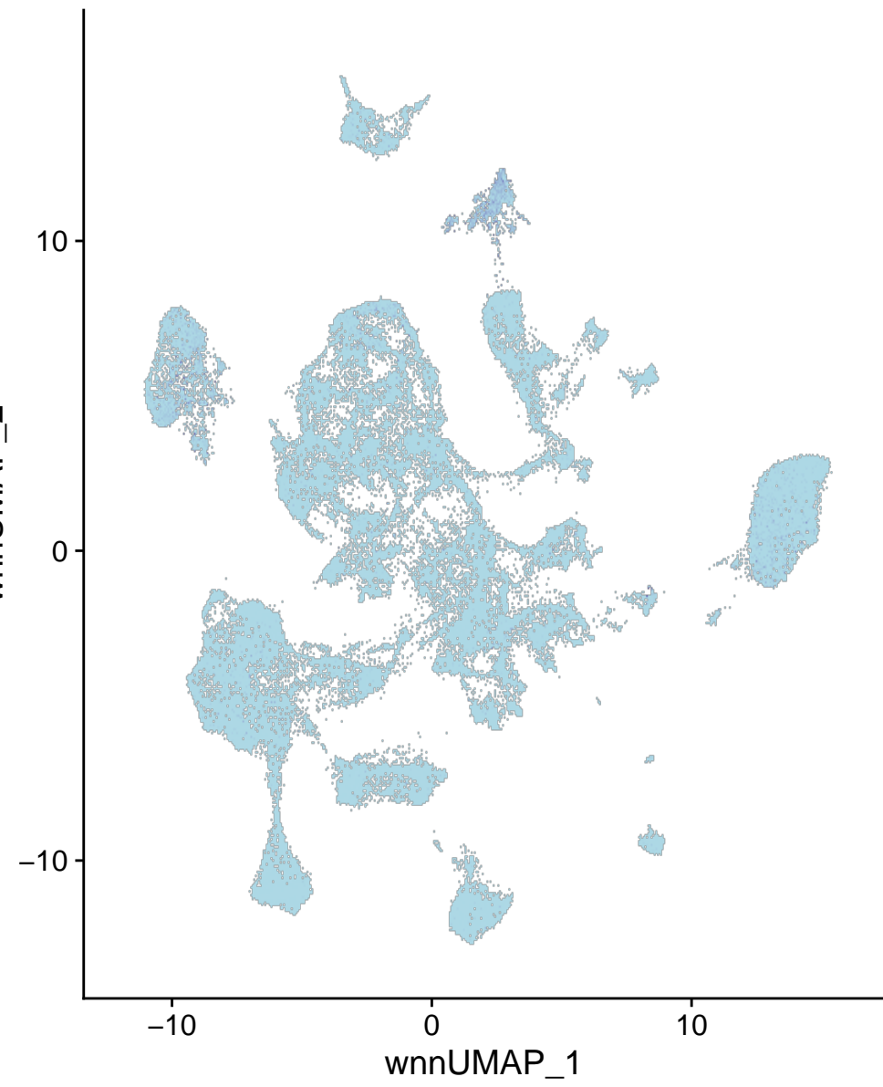
chr1-89137129-89137628
