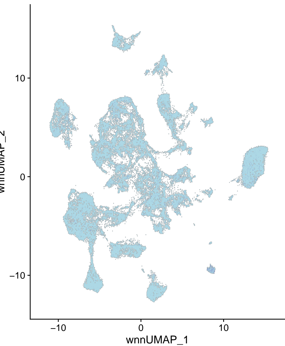
chr9-56700801-56701300
