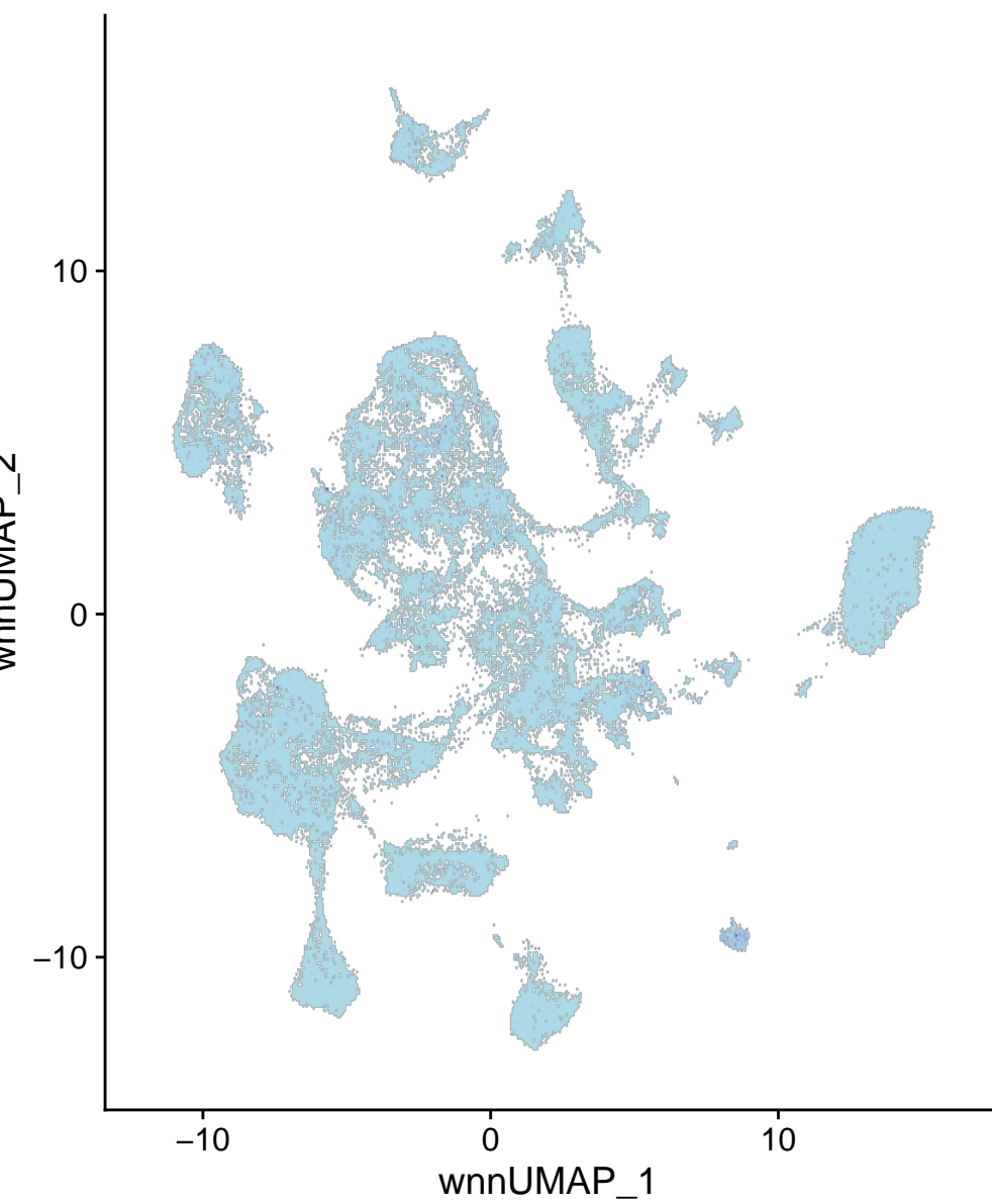
chr17-67451711-67452210
