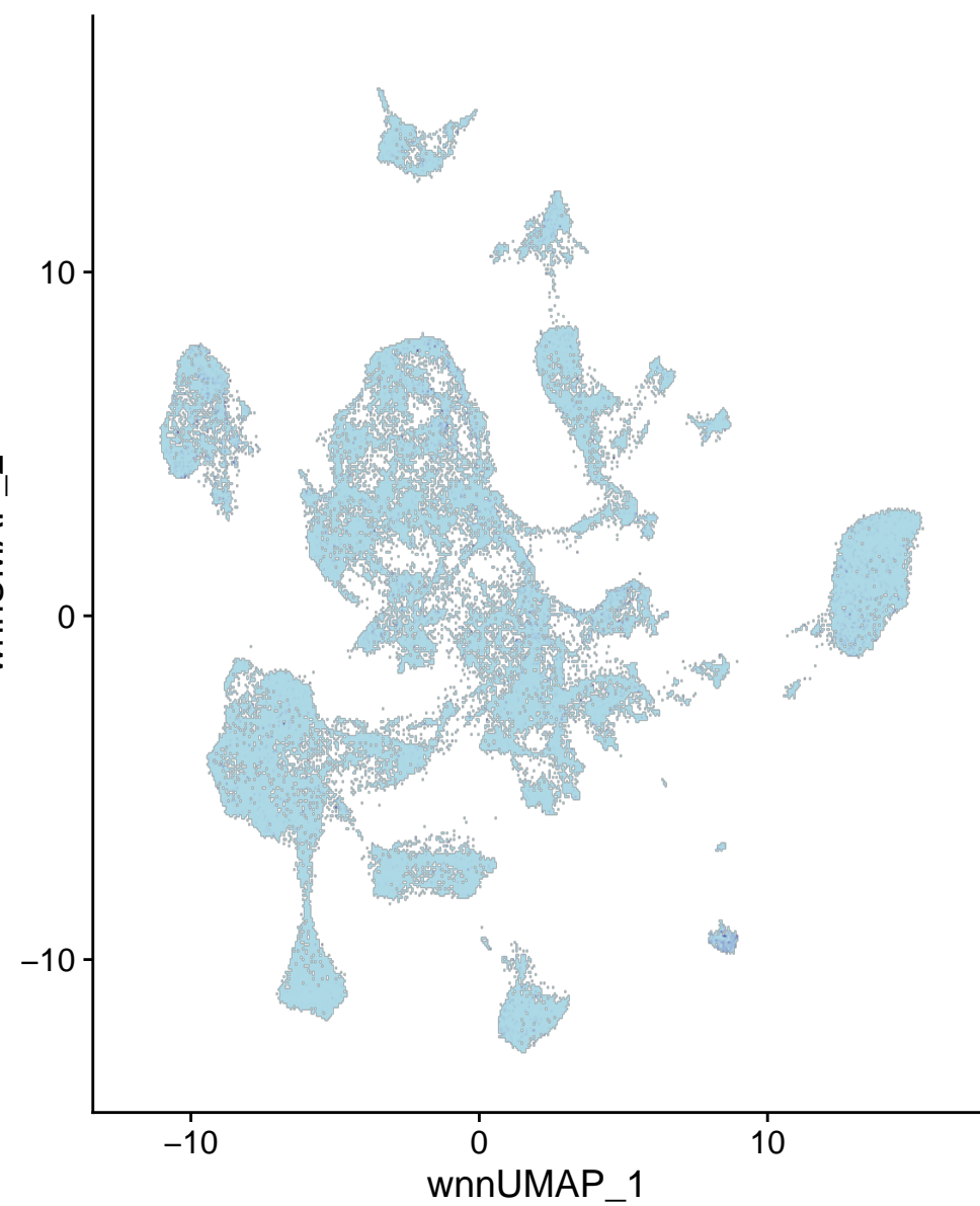
chr15-78082014-78082513
