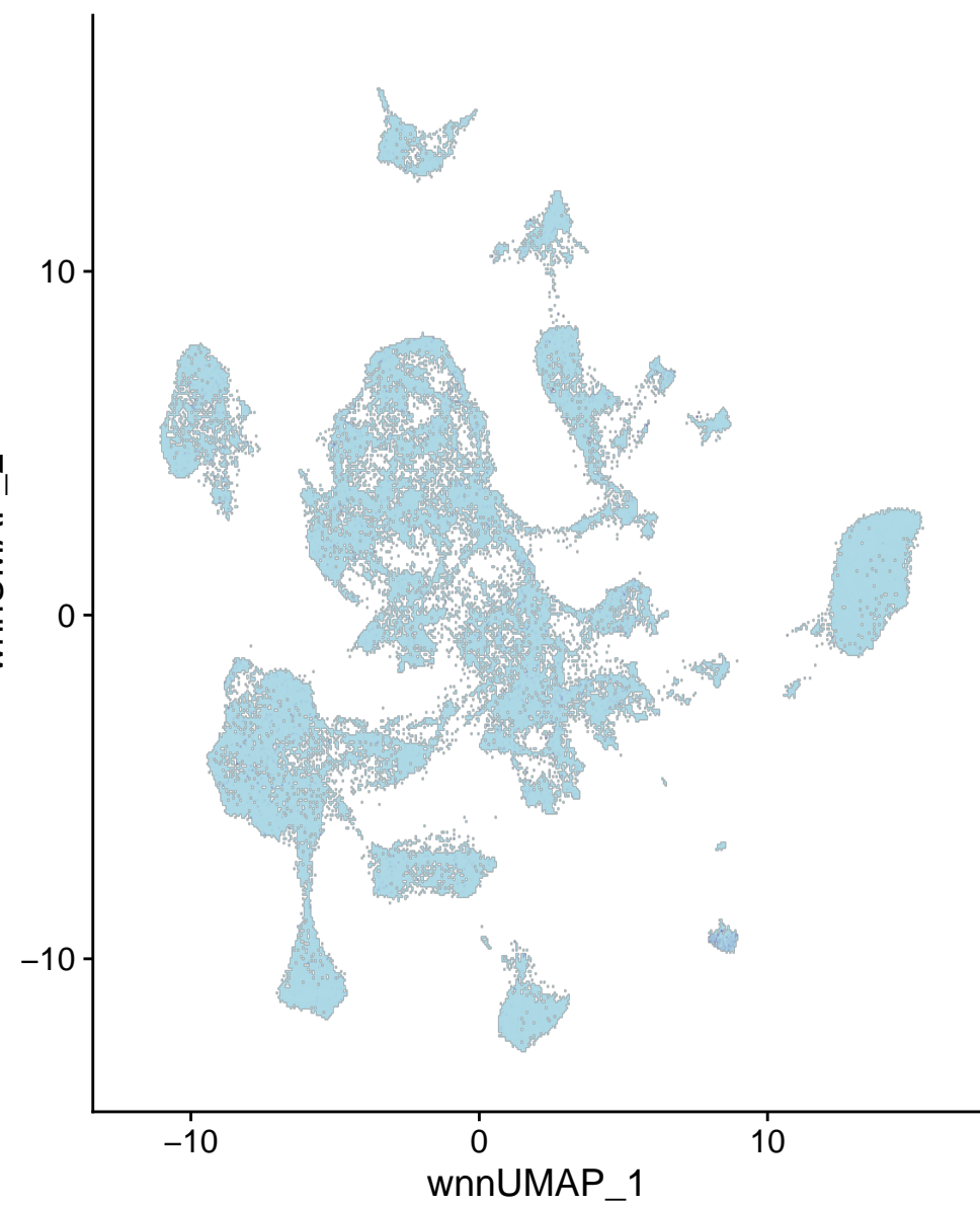
chr1-159358578-159359077
