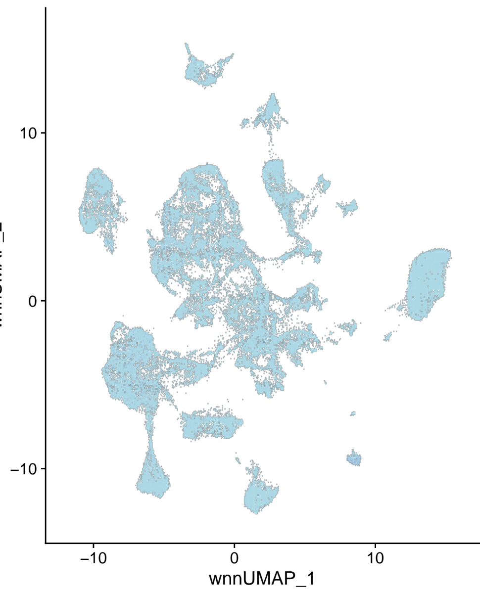
chr5-95978352-95978851
