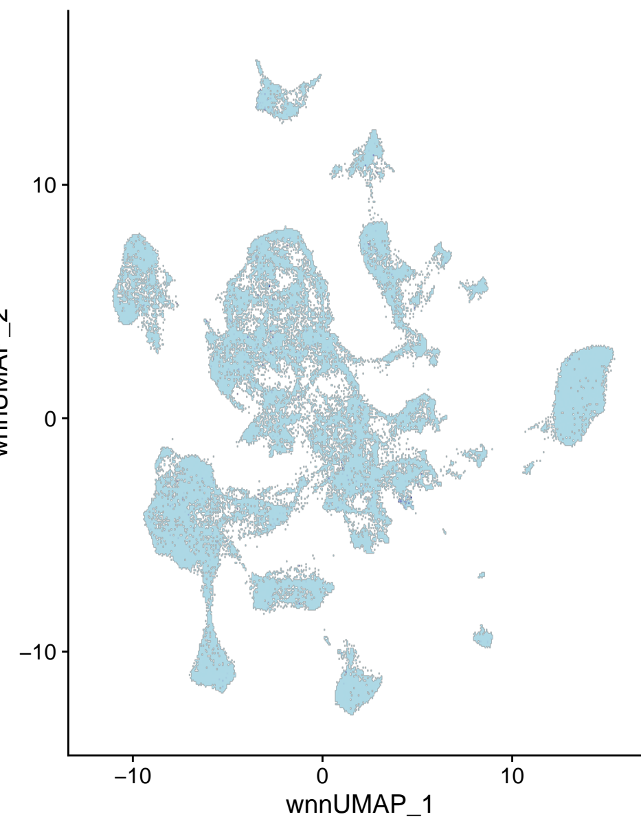
chr14-15681482-15681981
