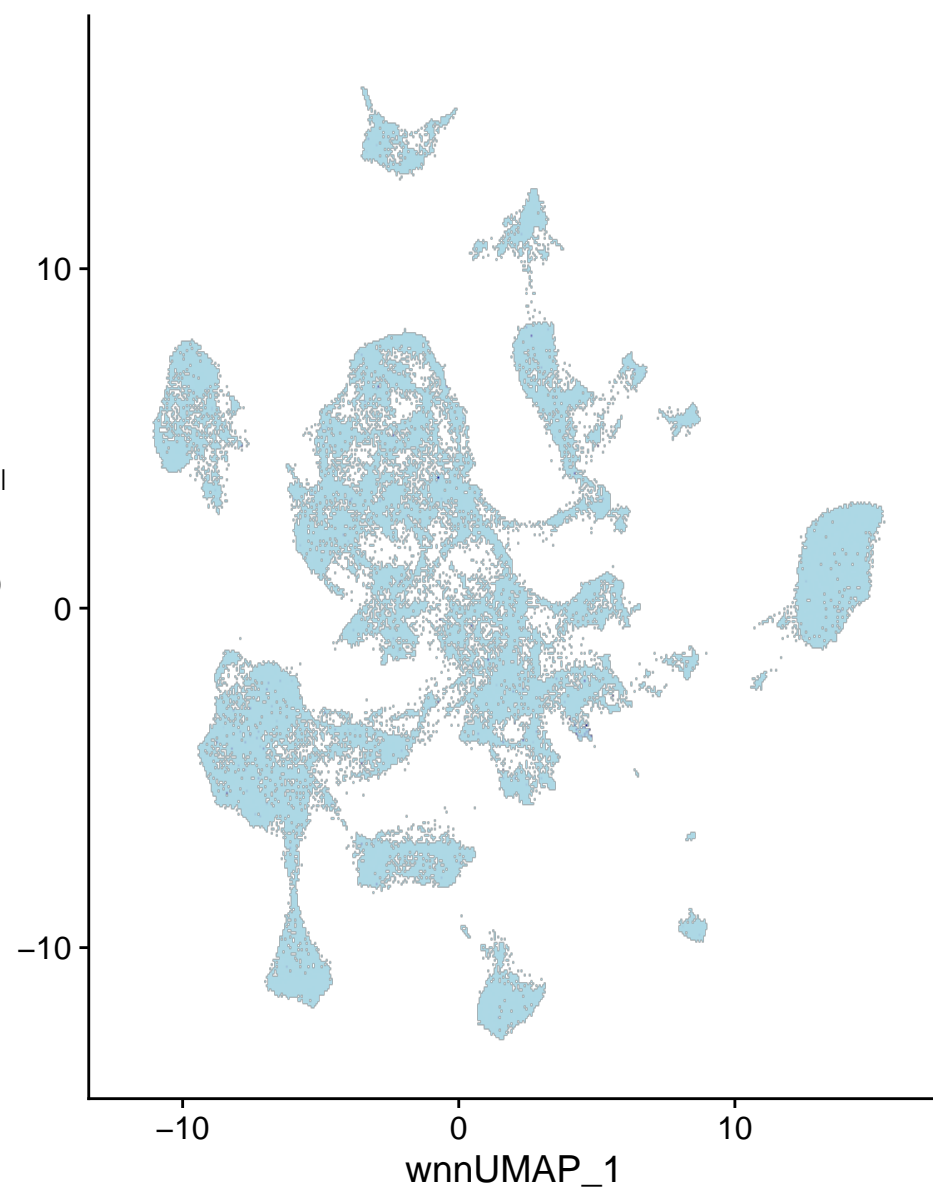
chr10-26228125-26228624
