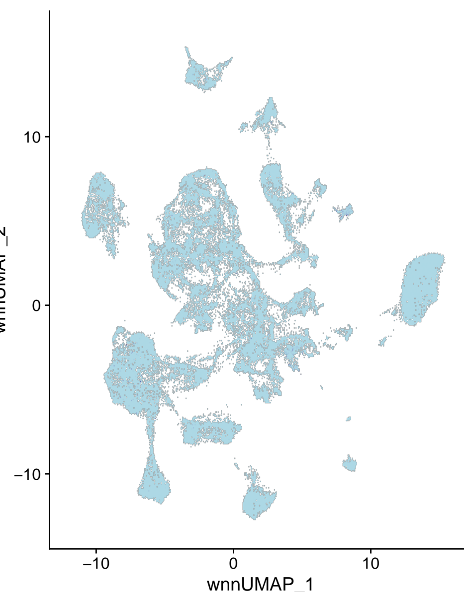
chr9-76829465-76829964
