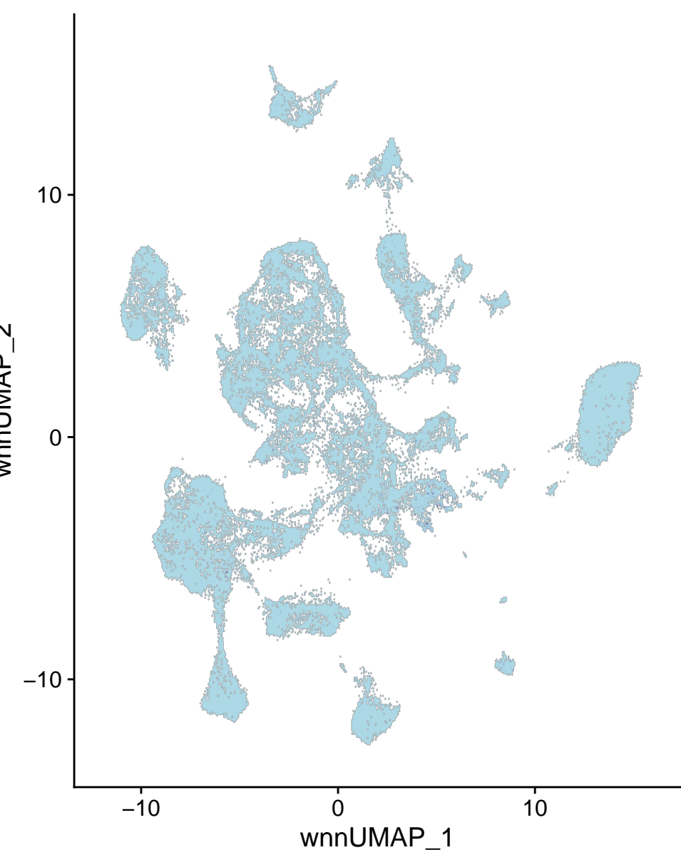
chr6-11583527-11584026
