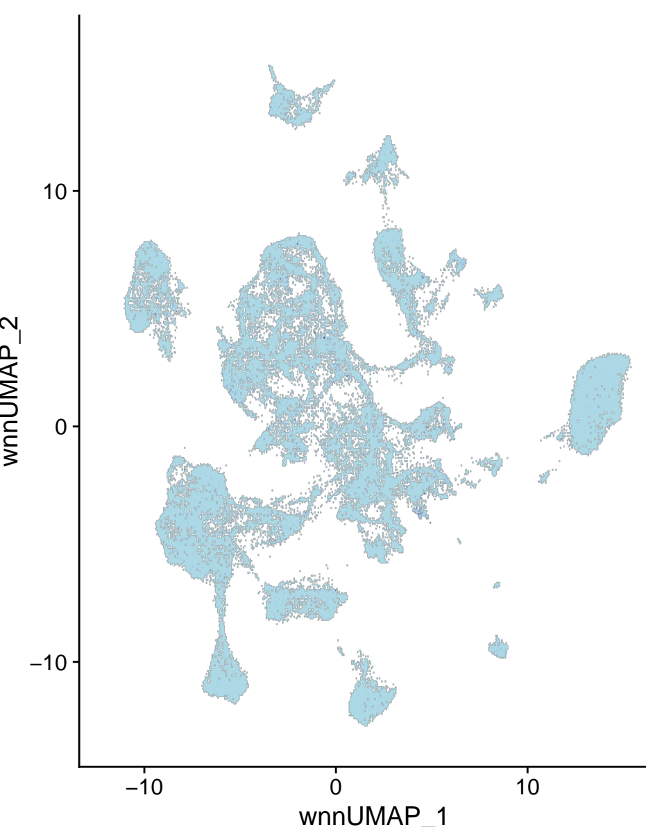
chr8-121458574-121459073
