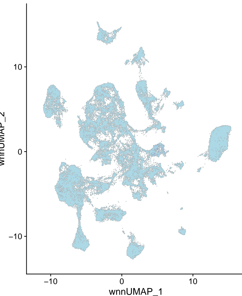
chr4-142298743-142299242
