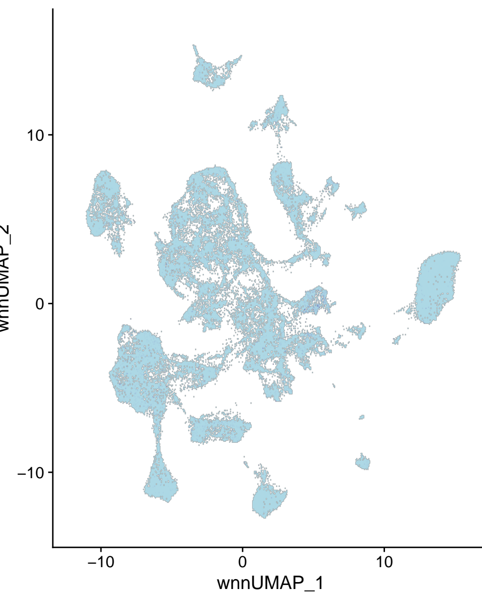
chr4-142298743-142299242
