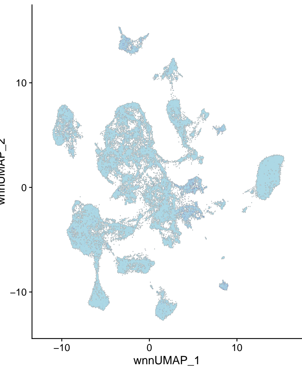
chr4-57058477-57058976
