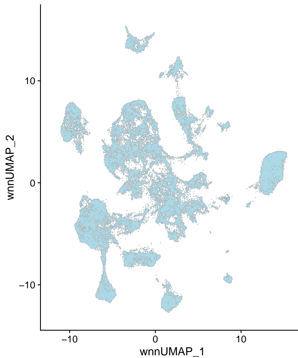
chr16-89429476-89429975
