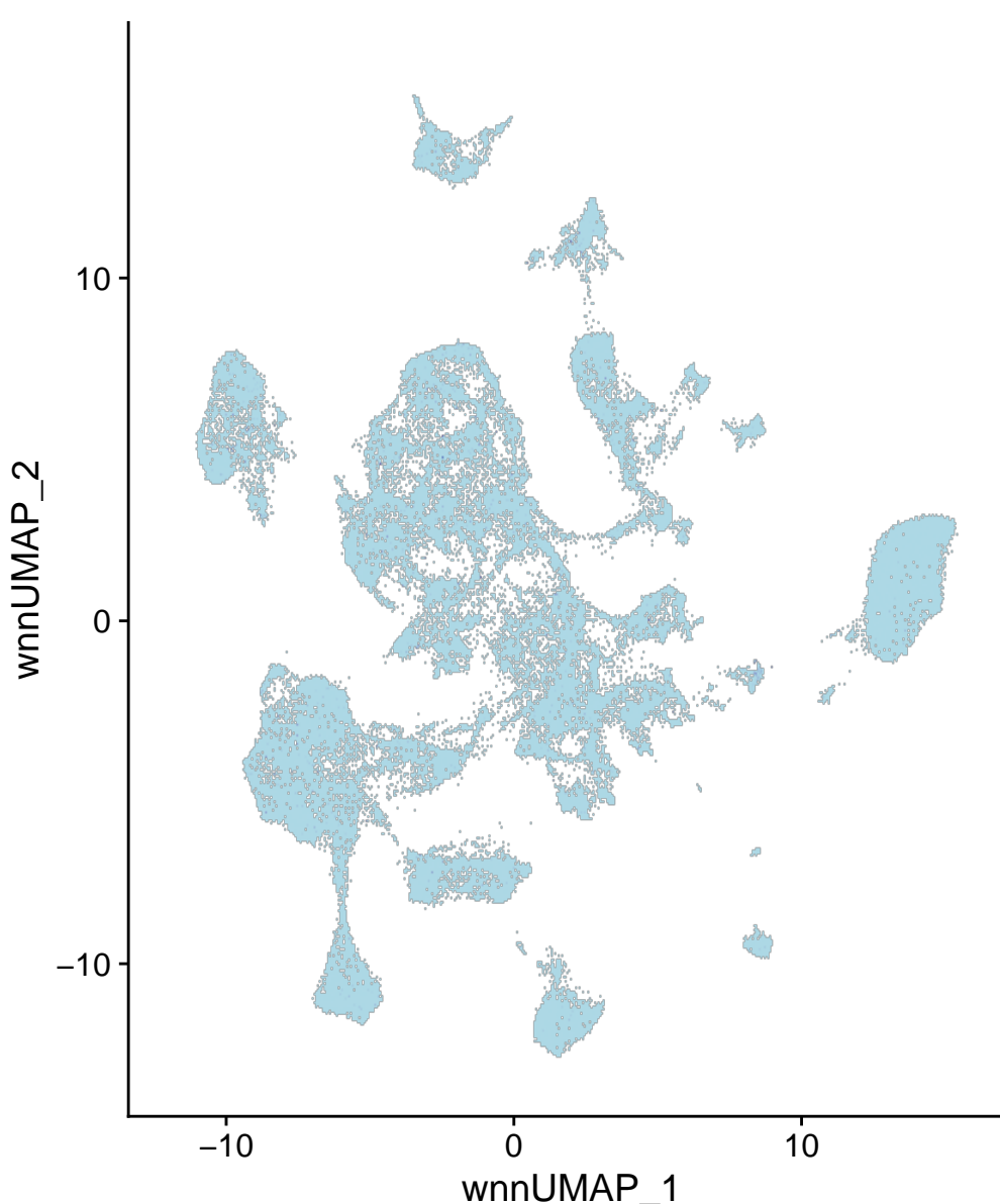
chr6-127443952-127444451
