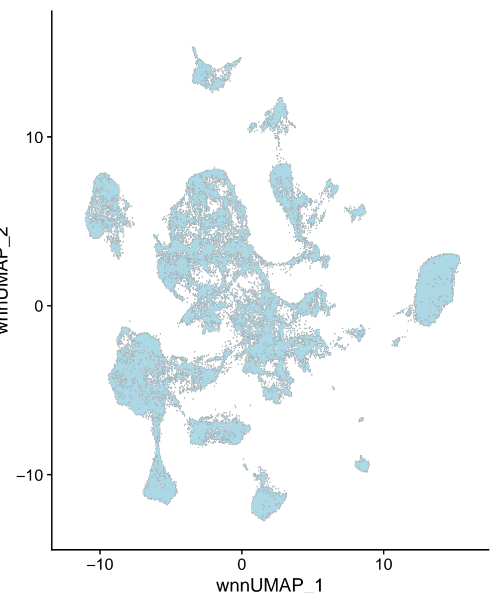
chr8-90536090-90536589
