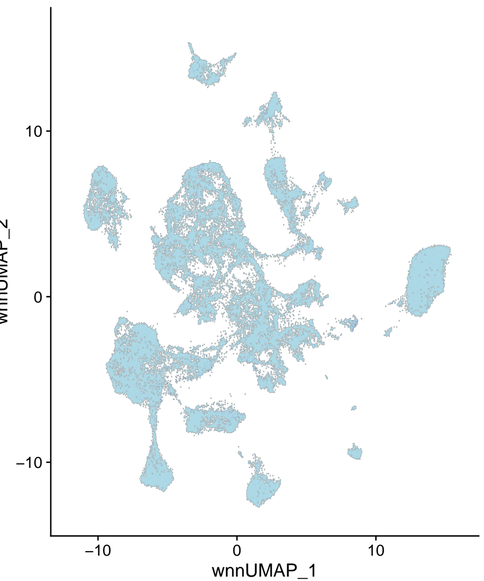
chr10-96747156-96747655
