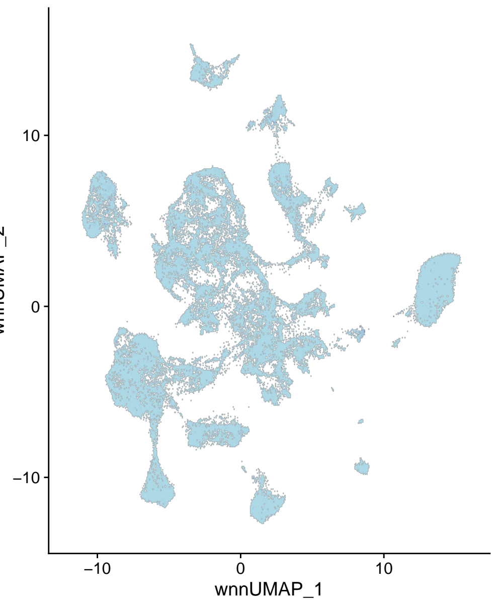
chr2-132449268-132449767
