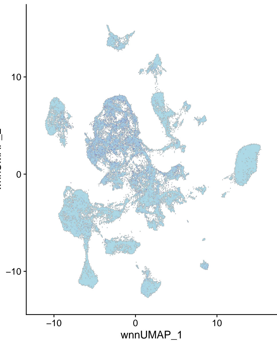
chr13-11968706-11969205
