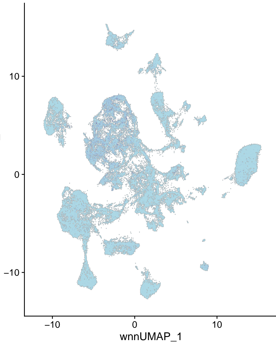
chr8-69149118-69149617
