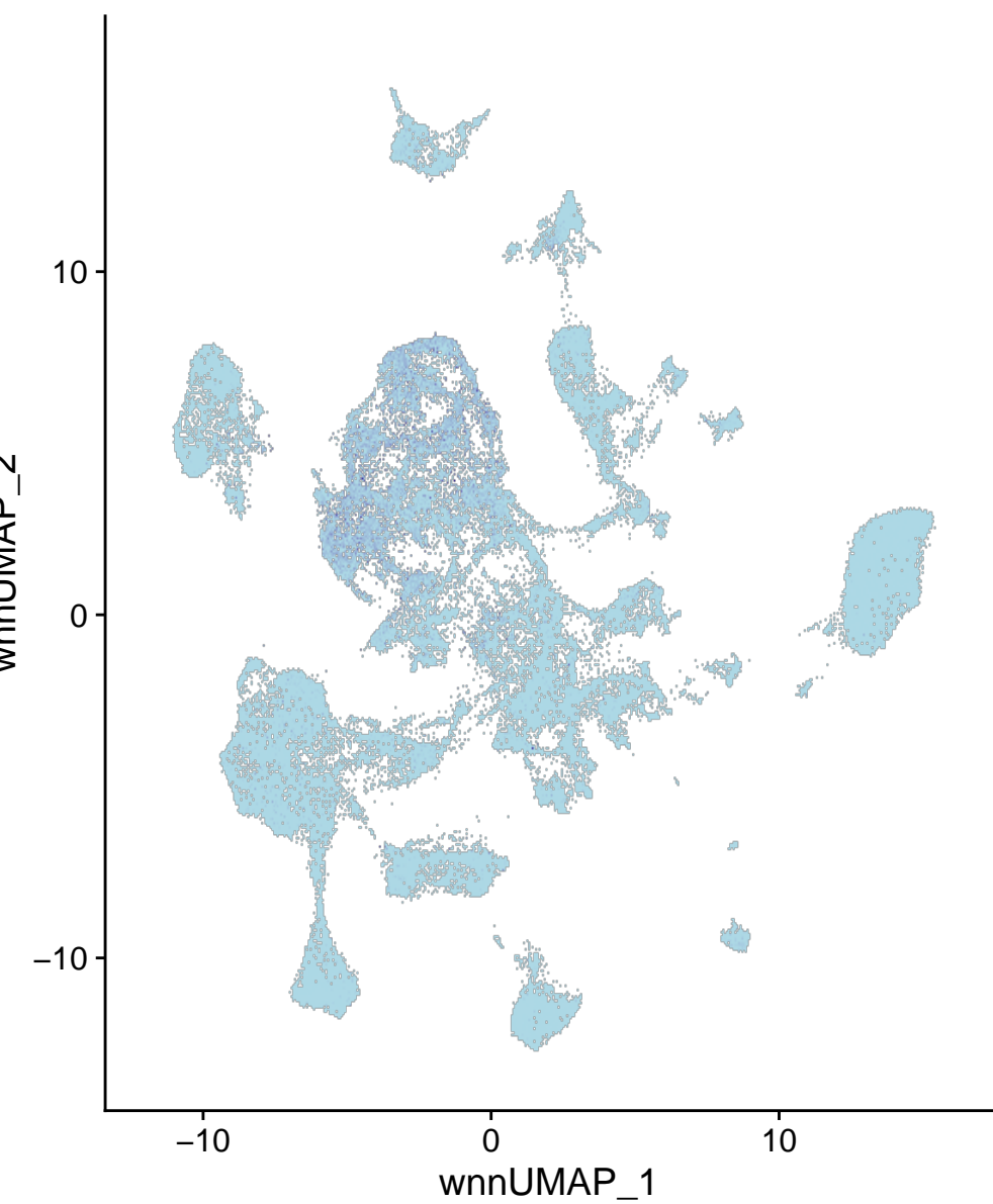
chr15-74667543-74668042
