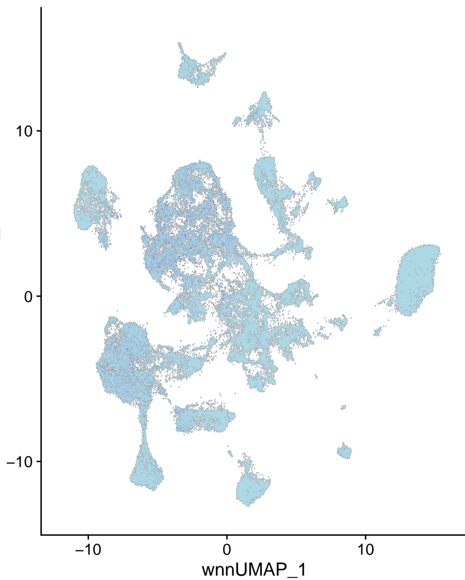
chr5-101825302-101825801
