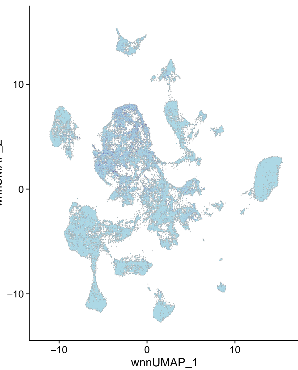
chr17-30770283-30770782
