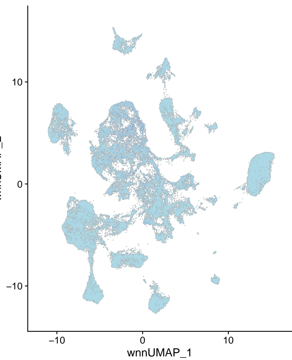
chr1-184879079-184879578
