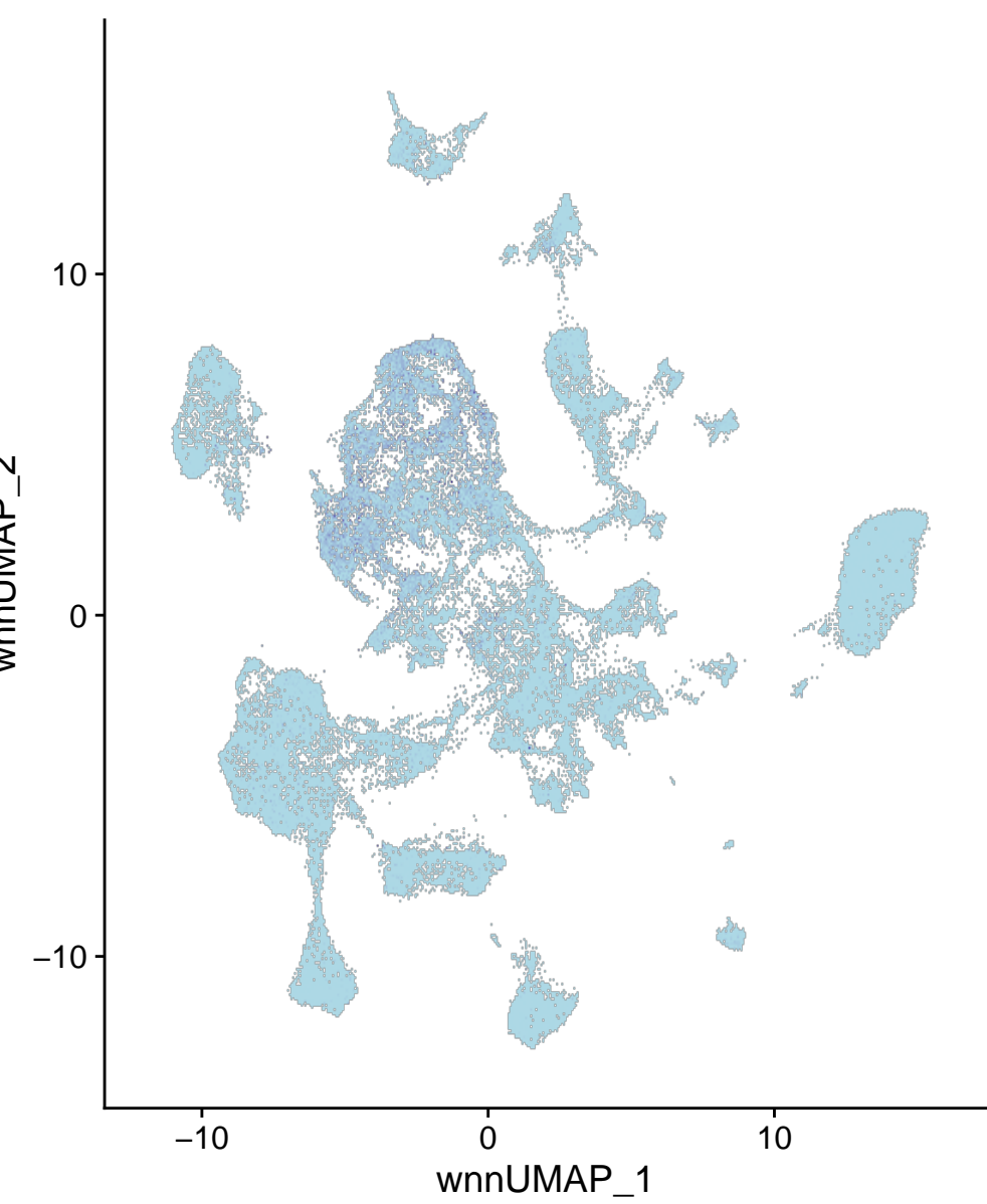
chr18-78205868-78206367
