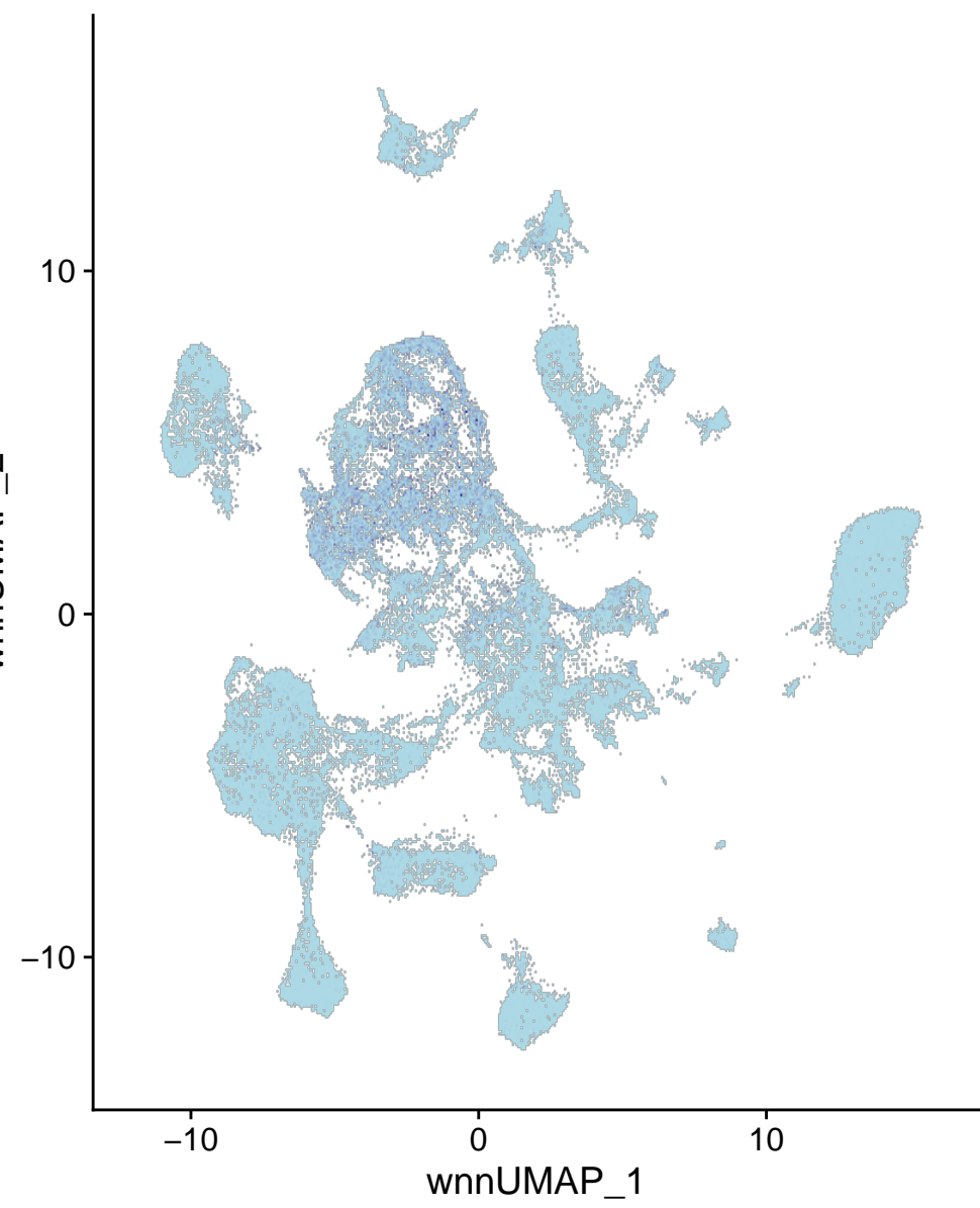
chr11-72175856-72176355
