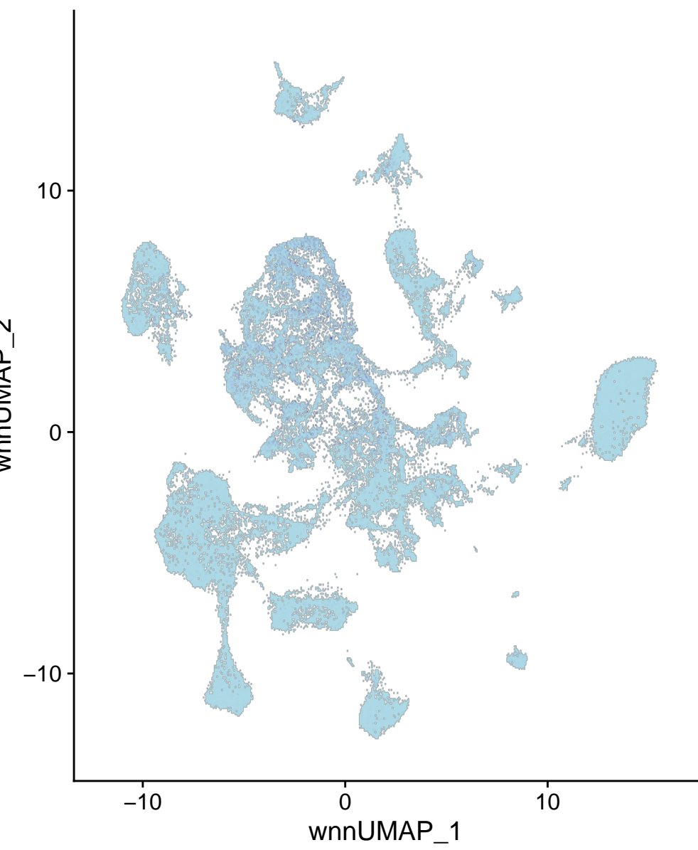
chr14-70920269-70920768
