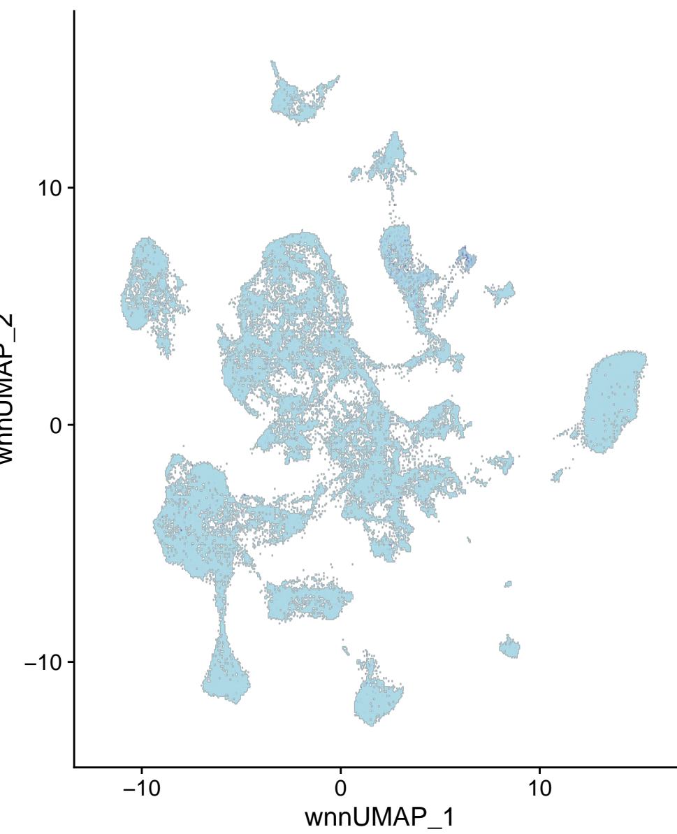
chr11-95571180-95571679
