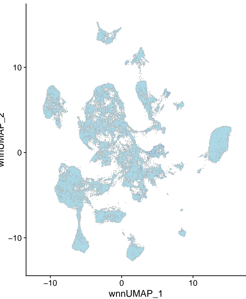
chr11-100516169-100516668
