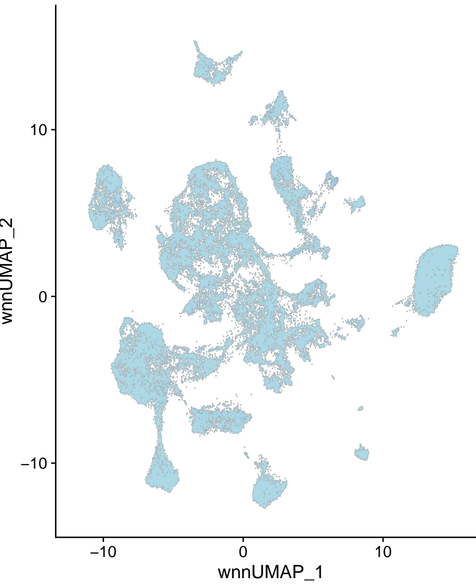
chr4-93184202-93184701
